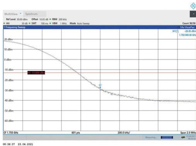
Band4-20MHz-QPSK-20300-1RB#99
