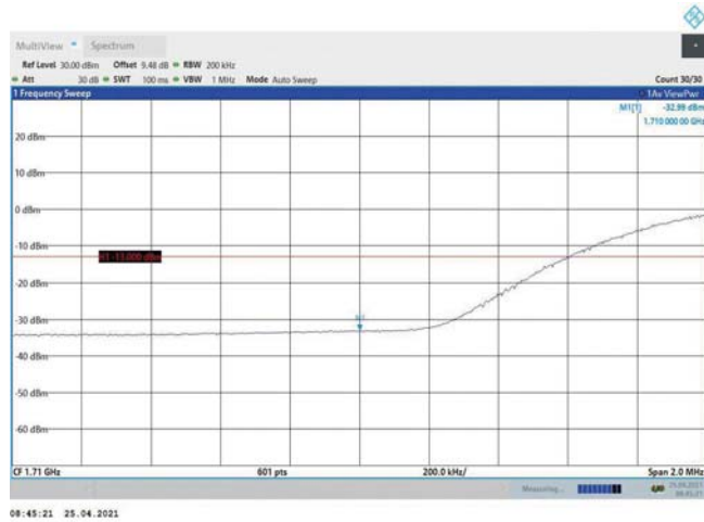
Band4-20MHz-QPSK-20050-100RB#0
