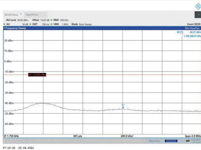
Band4-10MHz-QPSK-20350-1RB#0
