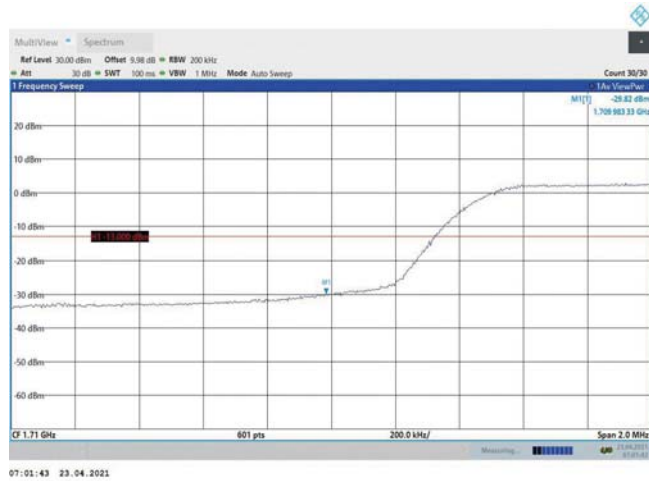
Band4-10MHz-QPSK-20000-50RB#0
