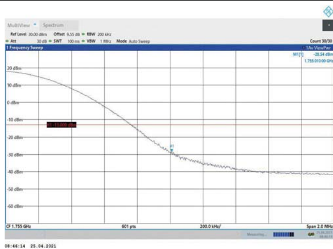
Band4-20MHz-QPSK-20300-1RB#99
