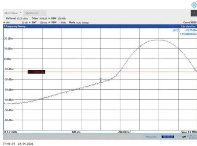
Band4-10MHz-QPSK-20000-1RB#0
