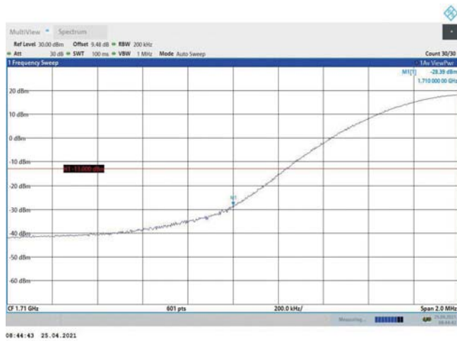
Band4-20MHz-QPSK-20050-1RB#0
