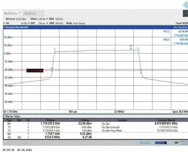
Band4-10MHz-QPSK-20000-50RB#0-8.974
