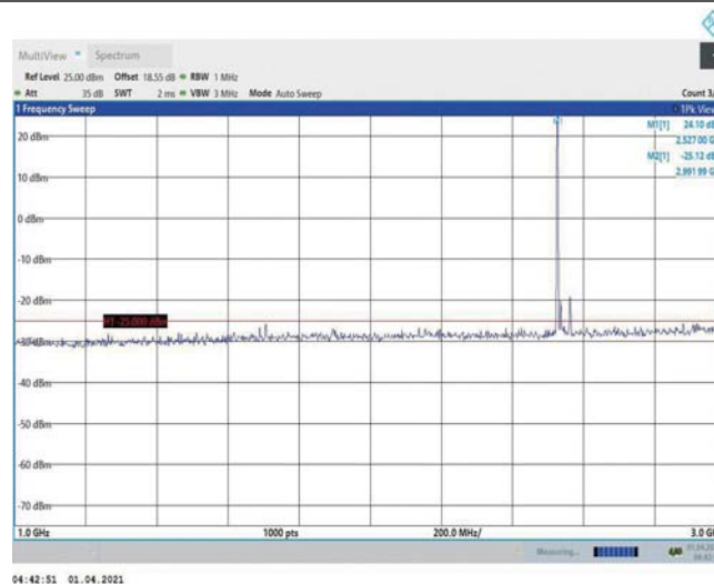
Band7-20MHz-QPSK-21100-1RB#0-Range2:1000~3000MHz
