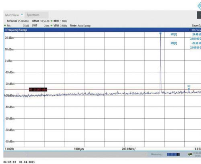
Band7-10MHz-QPSK-21400-1RB#0-Range2:1000~3000MHz
