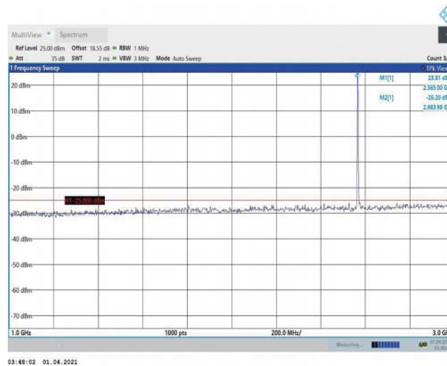
Band7-5MHz-QPSK-21425-1RB#0-Range2:1000~3000MHz
