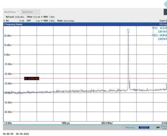
Band7-10MHz-QPSK-20800-1RB#0-Range2:1000~3000MHz
