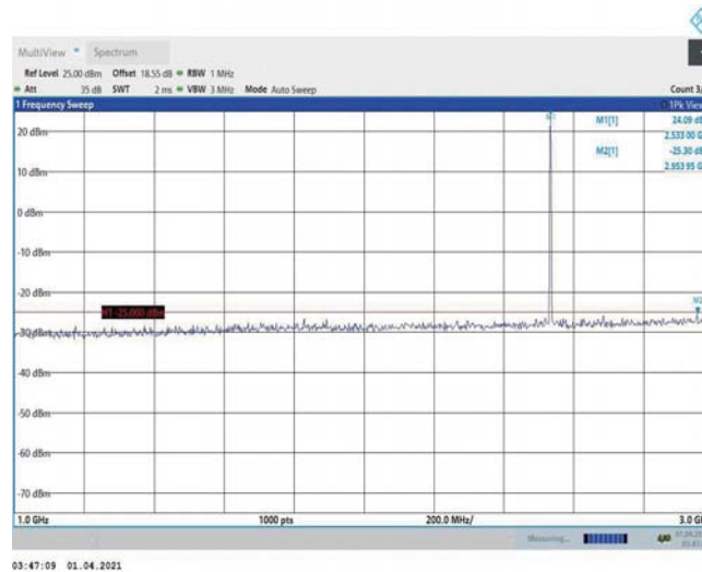
Band7-5MHz-QPSK-21100-1RB#0-Range2:1000~3000MHz
