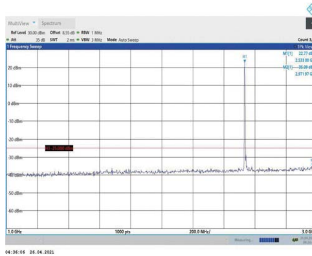
Band7-5MHz-QPSK-21100-1RB#0-Range2:1000~3000MHz
