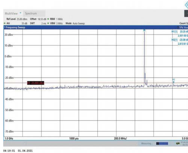
Band7-15MHz-QPSK-20825-1RB#0-Range2:1000~3000MHz
