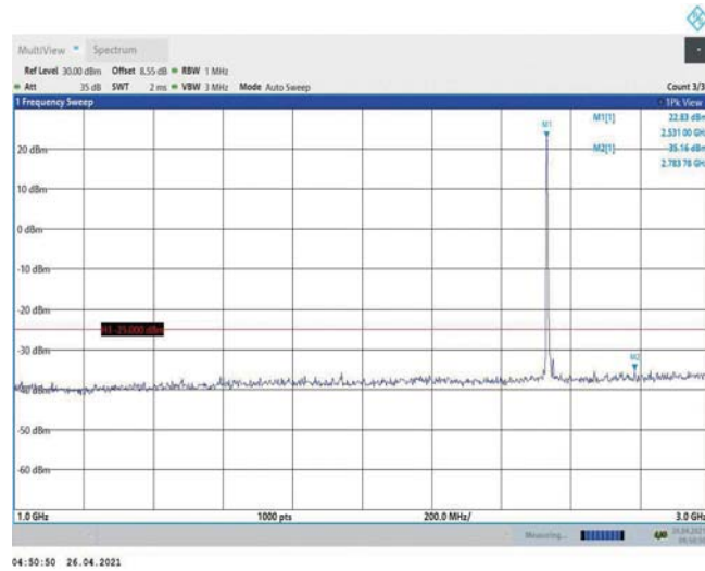
Band7-10MHz-QPSK-21100-1RB#0-Range2:1000~3000MHz
