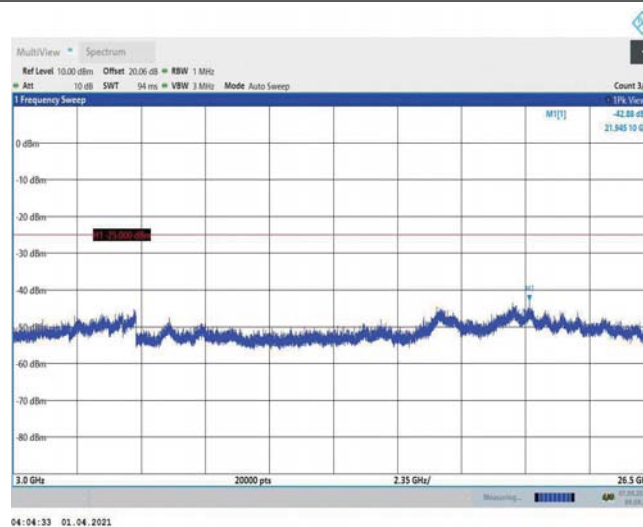
Band7-10MHz-QPSK-21100-1RB#0-Range3:3000~26500MHz
