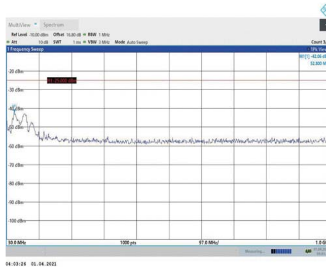
Band7-10MHz-QPSK-20800-1RB#0-Range1:30~1000MHz
