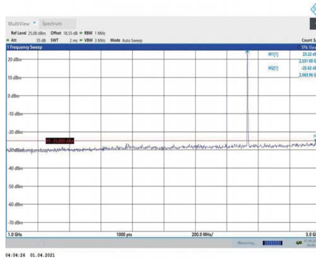
Band7-10MHz-QPSK-21100-1RB#0-Range2:1000~3000MHz
