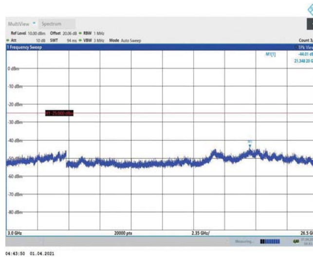
Band7-20MHz-QPSK-21350-1RB#0-Range3:3000~26500MHz
