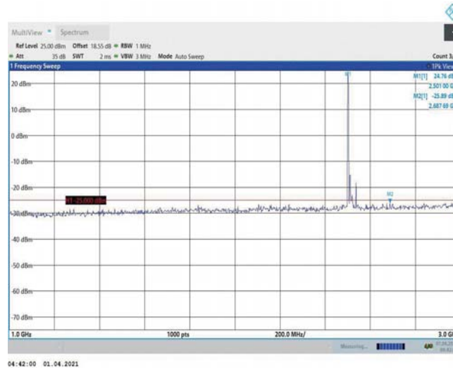
Band7-20MHz-QPSK-20850-1RB#0-Range2:1000~3000MHz
