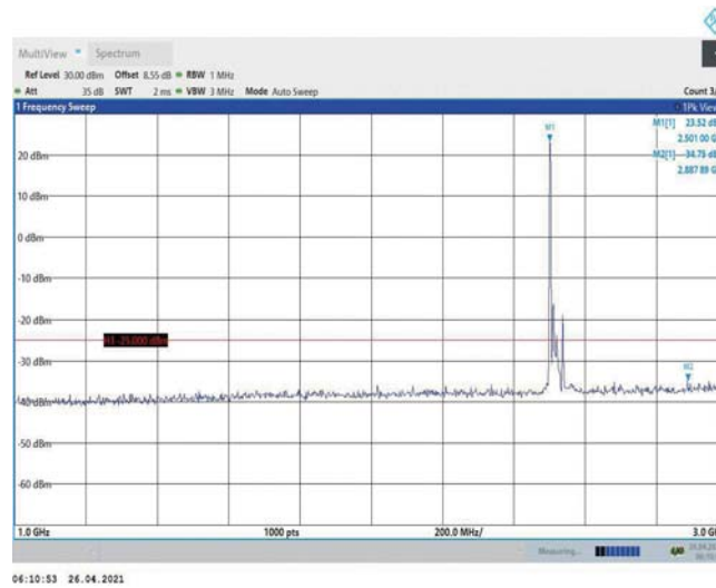
Band7-20MHz-QPSK-20850-1RB#0-Range2:1000~3000MHz
