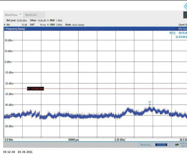
Band7-20MHz-QPSK-21350-1RB#0-Range3:3000~26500MHz
