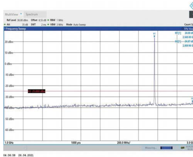
Band7-5MHz-QPSK-21425-1RB#0-Range2:1000~3000MHz
