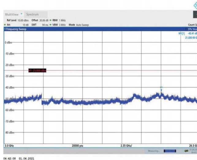
Band7-20MHz-QPSK-20850-1RB#0-Range3:3000~26500MHz
