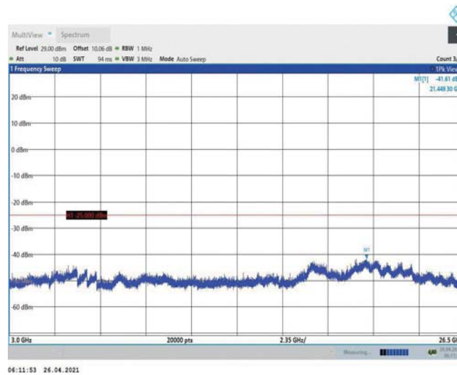
Band7-20MHz-QPSK-21100-1RB#0-Range3:3000~26500MHz
