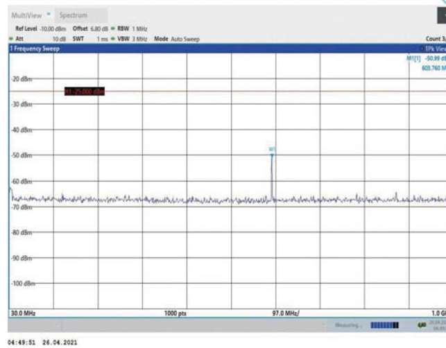
Band7-10MHz-QPSK-20800-1RB#0-Range1:30~1000MHz
