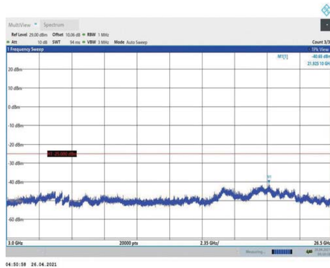
Band7-10MHz-QPSK-21100-1RB#0-Range3:3000~26500MHz
