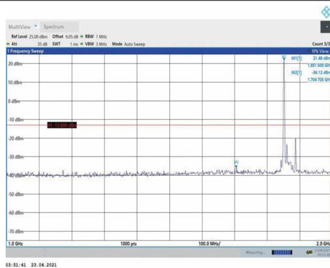
Band2-20MHz-QPSK-18700-1RB#0-Range2:1000~2000MHz
