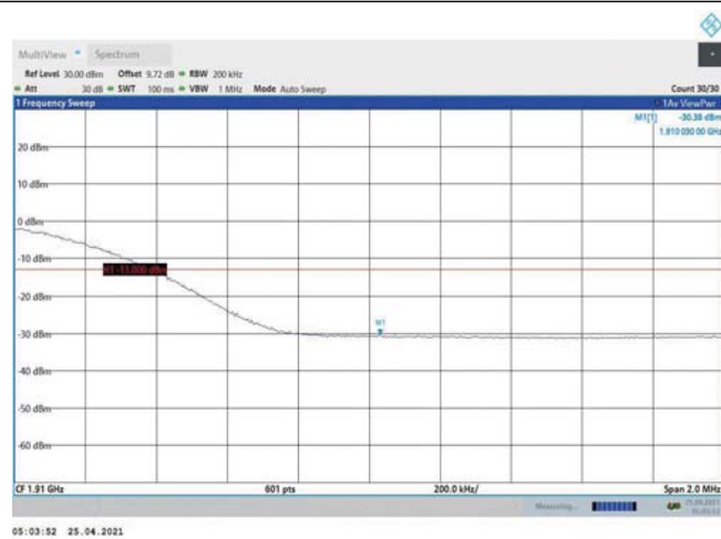
Band2-20MHz-QPSK-19100-100RB#0
