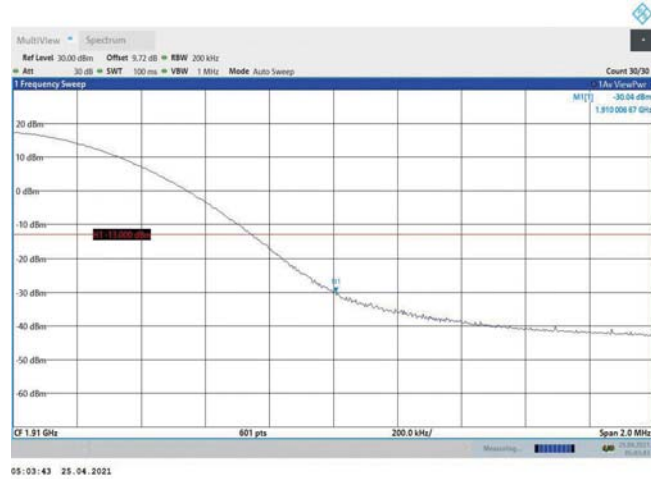
Band2-20MHz-16QAM-19100-1RB#99
