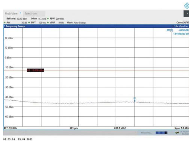
Band2-20MHz-16QAM-19100-1RB#0
