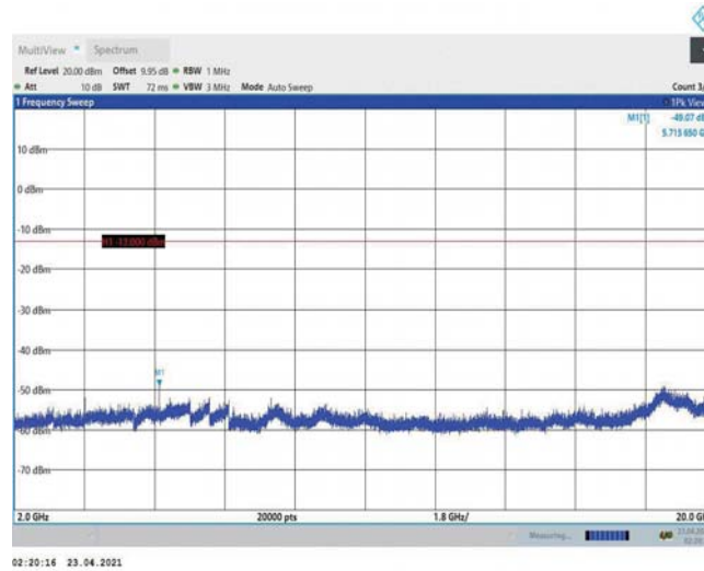
Band2-5MHz-QPSK-19175-1RB#0-Range3:2000~20000MHz
