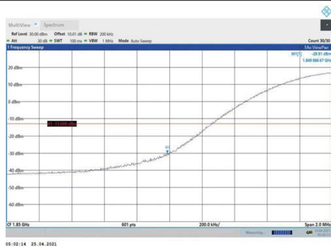
Band2-20MHz-16QAM-18700-1RB#0
