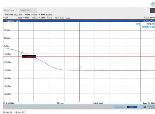
Band2-20MHz-16QAM-19100-100RB#0
