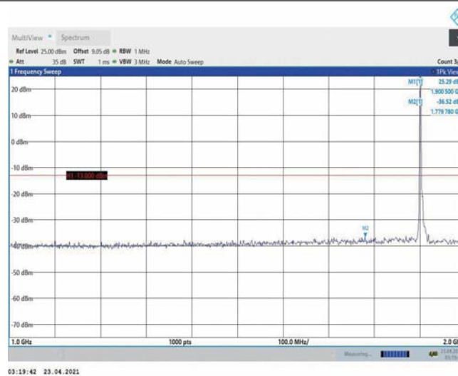
Band2-10MHz-QPSK-19150-1RB#0-Range2:1000~2000MHz
