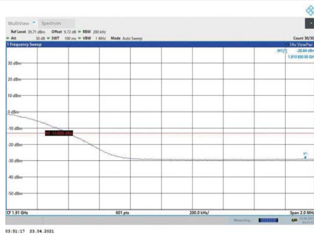
Band2-20MHz-16QAM-19100-100RB#0
