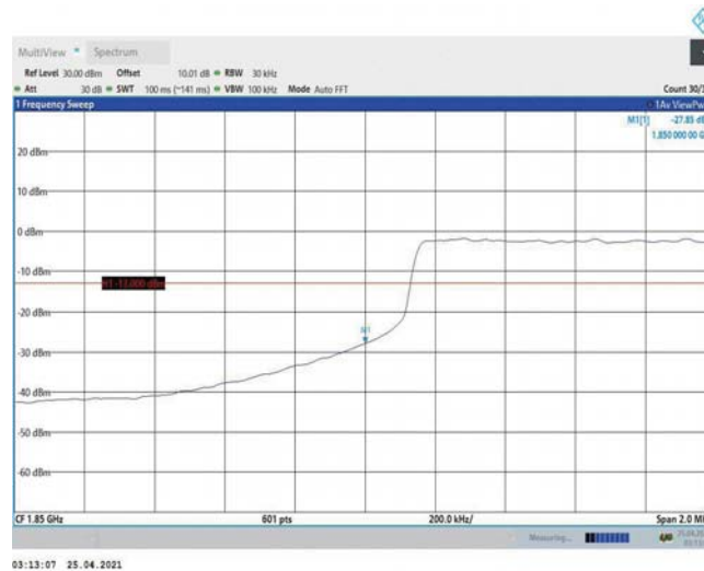
Band2-3MHz-QPSK-18615-15RB#0
