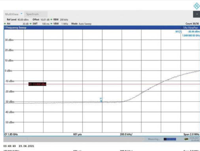
Band2-20MHz-QPSK-18700-100RB#0
