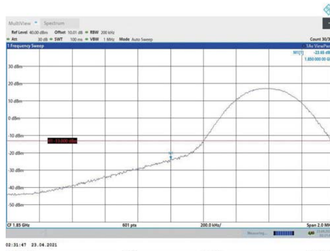
Band2-10MHz-QPSK-18650-1RB#0
