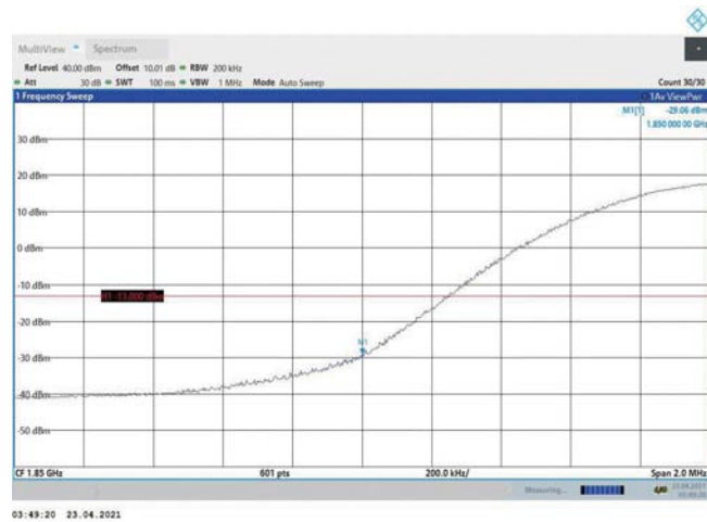
Band2-20MHz-16QAM-18700-1RB#0
