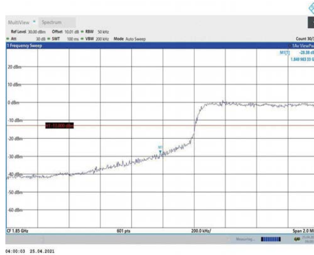
Band2-5MHz-QPSK-18625-25RB#0
