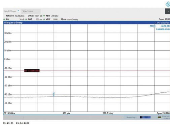
Band2-20MHz-16QAM-18700-1RB#99
