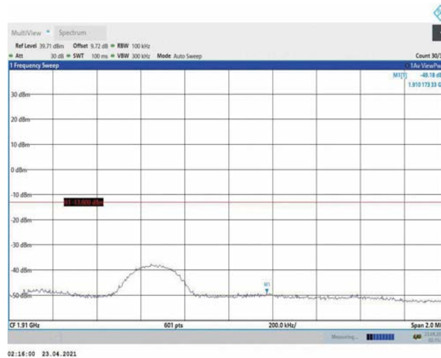
Band2-5MHz-QPSK-19175-1RB#0
