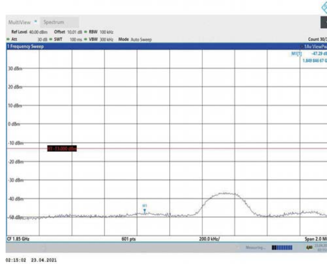
Band2-5MHz-QPSK-18625-1RB#24
