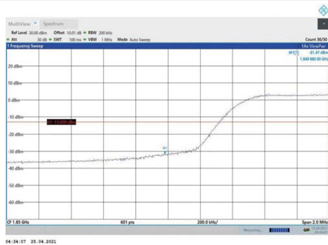
Band2-10MHz-QPSK-18650-50RB#0
