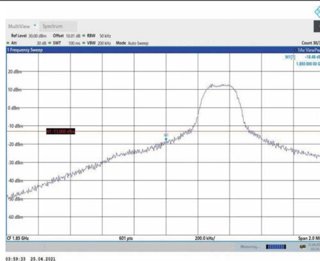
Band2-5MHz-16QAM-18625-1RB#0
