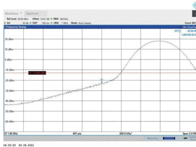
Band2-10MHz-QPSK-18650-1RB#0
