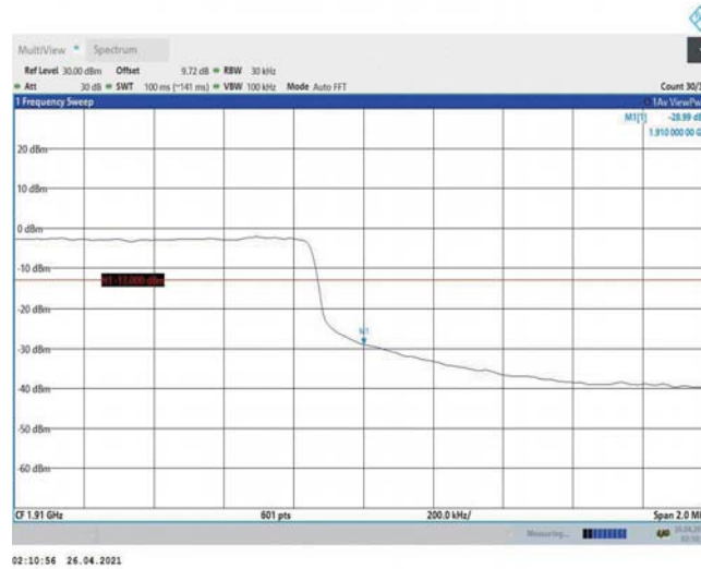
Band2-3MHz-QPSK-19185-15RB#0
