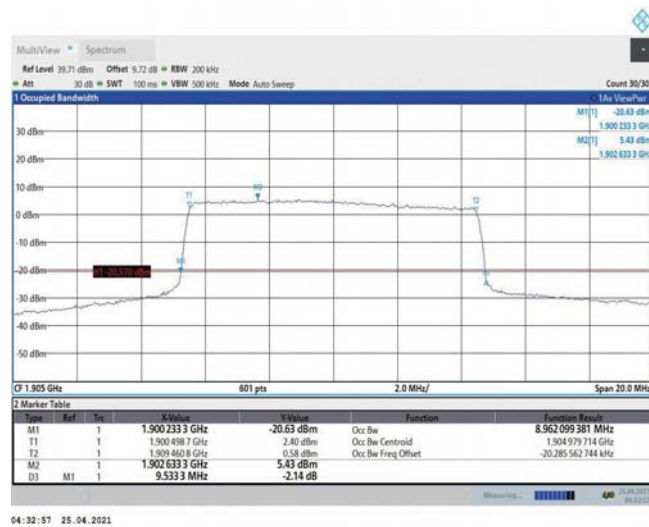
Band2-10MHz-QPSK-19150-50RB#0-8.962
