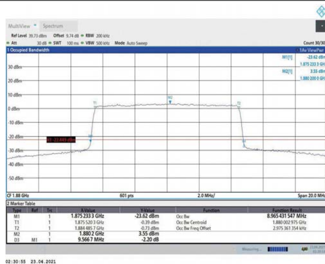
Band2-10MHz-16QAM-18900-50RB#0-8.965
