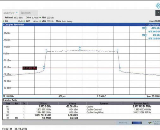
Band2-10MHz-QPSK-18900-50RB#0-8.978
