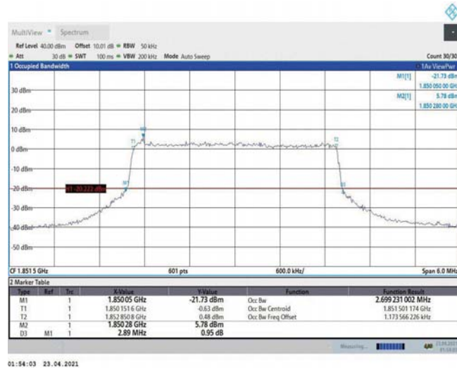
Band2-3MHz-QPSK-18615-15RB#0-2.699
