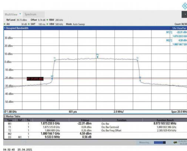
Band2-10MHz-16QAM-18900-50RB#0-8.973
