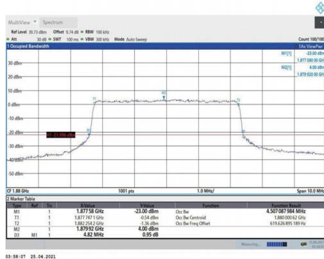
Band2-5MHz-QPSK-18900-25RB#0-4.507
