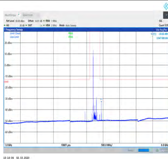
1-N78-3700-3800-PC2-30-100-L-1-DFT-QPSK-Edge _1RB_Left-1@0-1000-6000-Ant1-3947.00--33.82--13 -PASS
