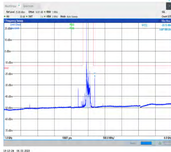
1-N78-3450-3550-PC2-30-100-L-1-DFT-QPSK-Edge _1RB_Left-1@0-1000-6000-Ant1-3697.00--23.13--13 -PASS
