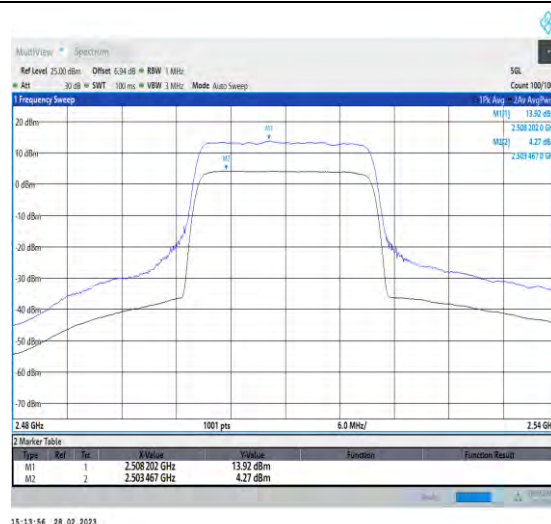
1-N7-PC3-15-20-L-2-CP-256QAM-Outter_Full-106@ 0-Ant1-9.65-100%-0.00-9.65-PASS-≤13
