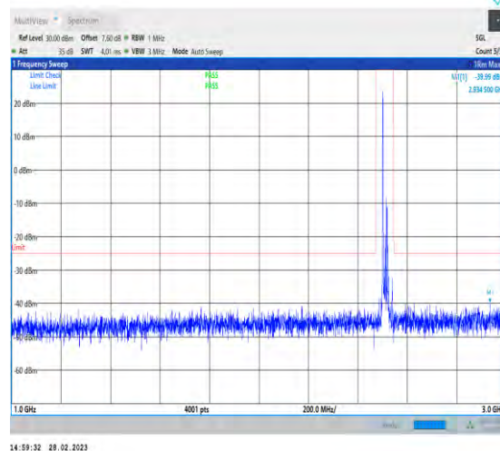
1-N7-PC3-15-20-L-1-DFT-PI2BPSK-Inner_1RB_Left- 1@1-1000-3000-Ant1-2934.50--39.99--25-PASS
