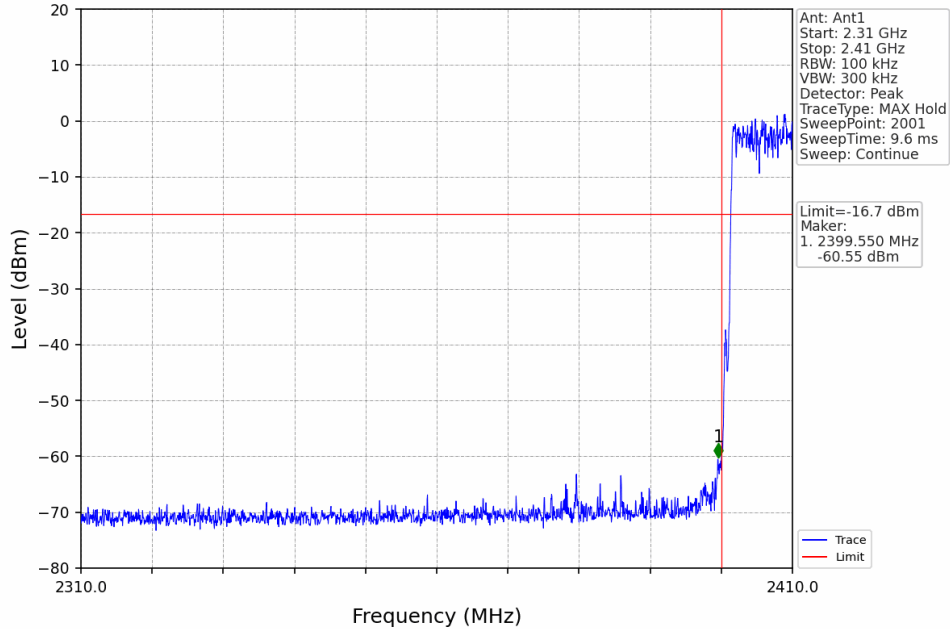
Pi/4DQPSK_2DH5_HOPP_Ant1_NTNV
