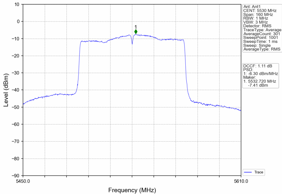
802.11ac(VHT80)_LCH_5530MHz_Ant1_NTNV
