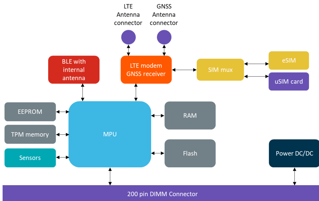
FIGURE 1: S-2CONNECT CREO SOM BLOCK DIAGRAM
