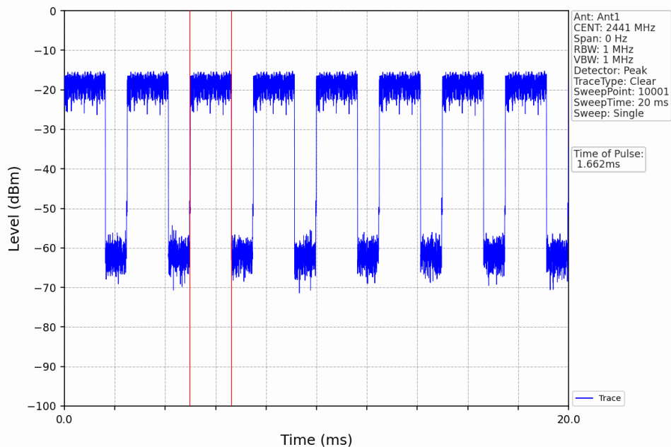
Pi/4DQPSK_2DH3_HOPP_Ant1_NTNV
