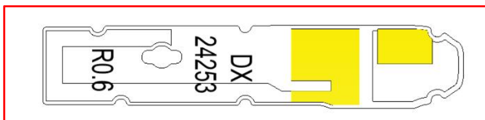
天线外观图
