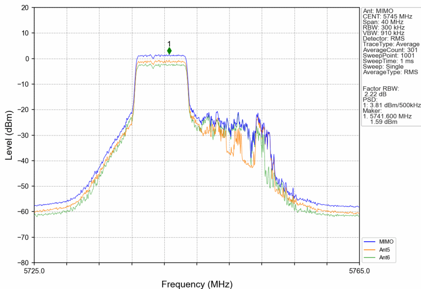
802.11be(EHT20)_LCH_5745MHz_26+52_/_MIMO_NTNV
