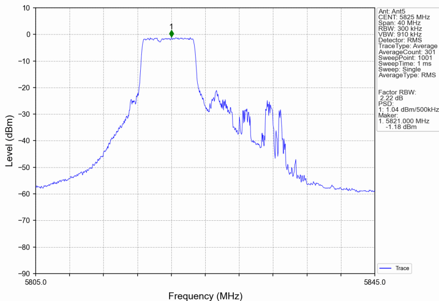
802.11be(EHT20)_HCH_5825MHz_26+52_/_Ant5_NTNV
