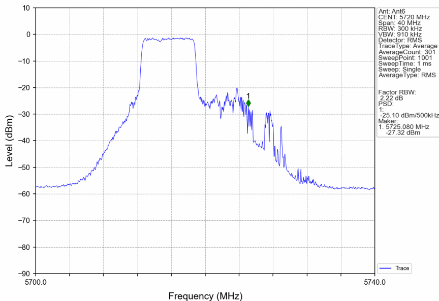
802.11be(EHT20)_HCH_5720MHz_26+52_/_Ant6_NTNV
