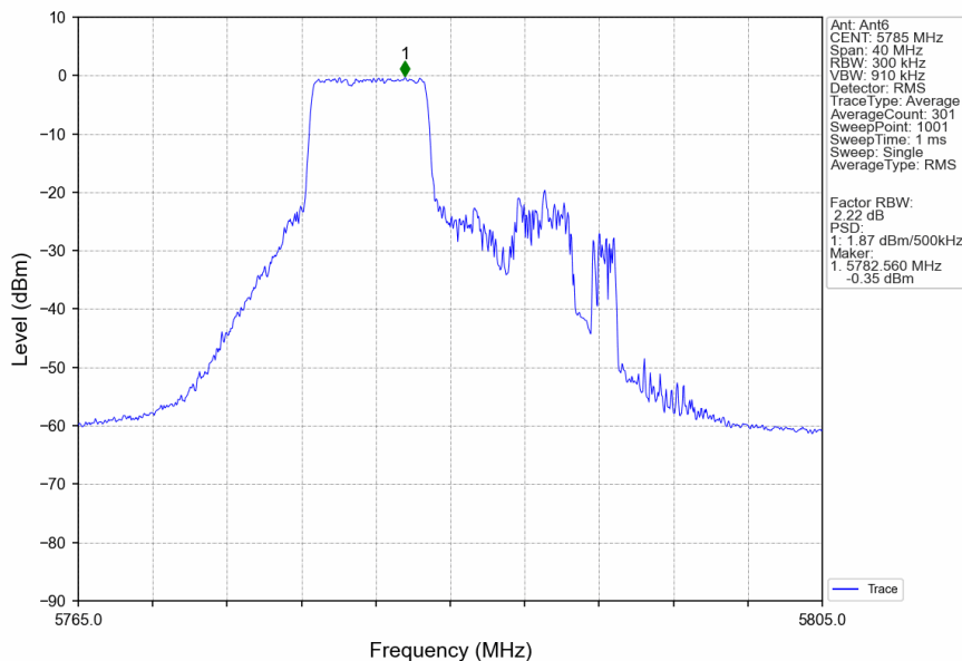
802.11be(EHT20)_MCH_5785MHz_26+52_/_Ant6_NTNV
