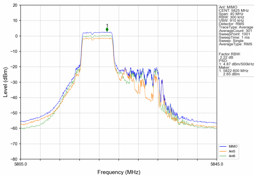
802.11be(EHT20)_HCH_5825MHz_26+52_/_MIMO_NTNV
