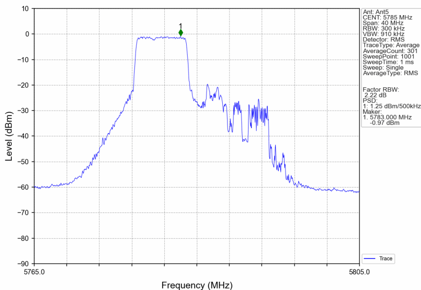
802.11be(EHT20)_MCH_5785MHz_26+52_/_Ant5_NTNV
