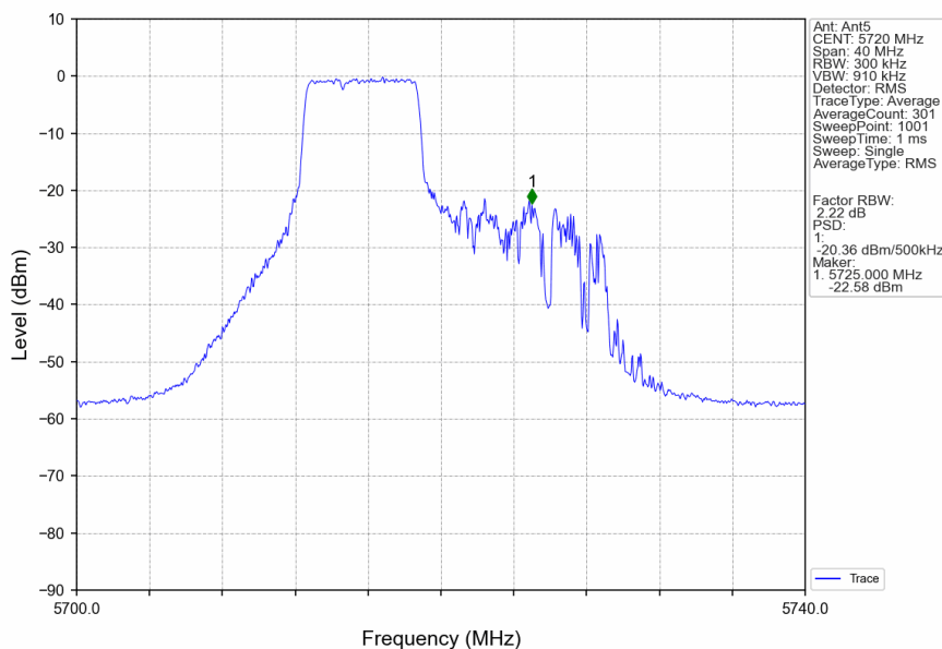
802.11be(EHT20)_HCH_5720MHz_26+52_/_Ant5_NTNV
