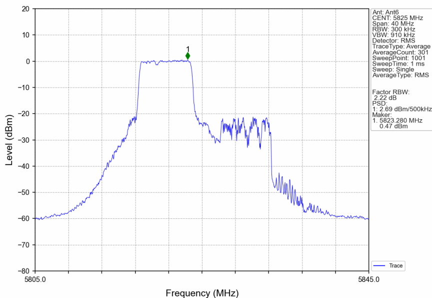
802.11be(EHT20)_HCH_5825MHz_26+52_/_Ant6_NTNV
