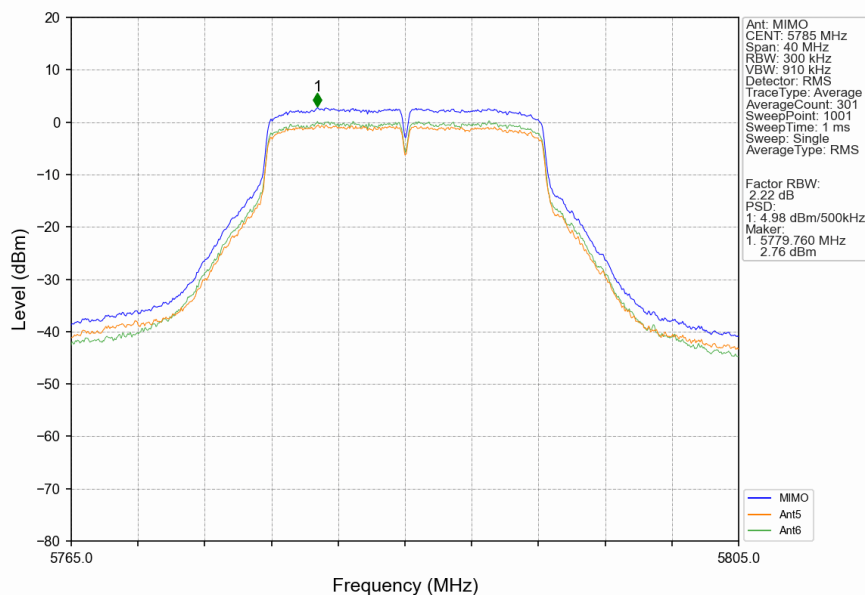
802.11a_MCH_5785MHz_MIMO_NTNV
