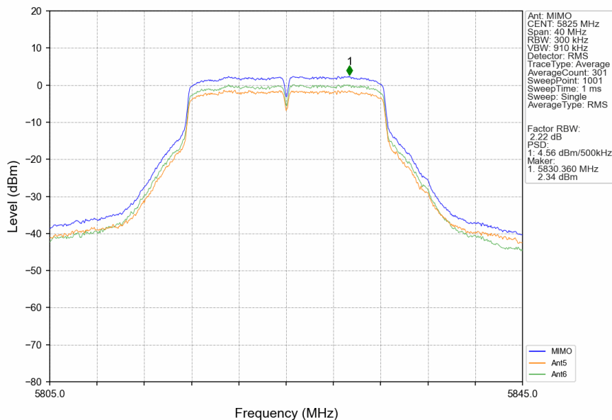
802.11a_HCH_5825MHz_MIMO_NTNV
