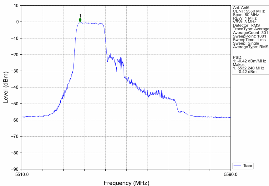
802.11be(EHT40)_MCH_5550MHz_26+106_/_Ant6_NTNV
