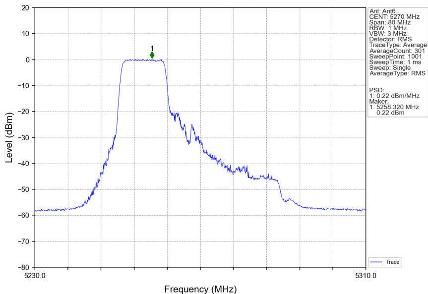
802.11be(EHT40)_LCH_5270MHz_26+106_/_Ant6_NTNV
