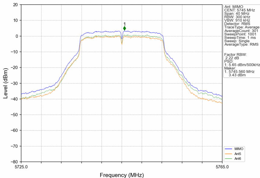
802.11a_LCH_5745MHz_MIMO_NTNV
