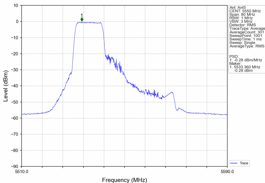
802.11be(EHT40)_MCH_5550MHz_26+106_/_Ant5_NTNV
