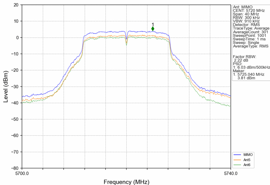
802.11a_HCH_5720MHz_MIMO_NTNV
