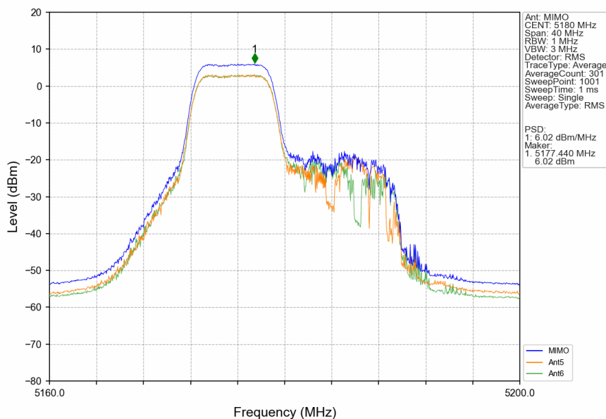
802.11be(EHT20)_LCH_5180MHz_26+52_/_MIMO_NTNV
