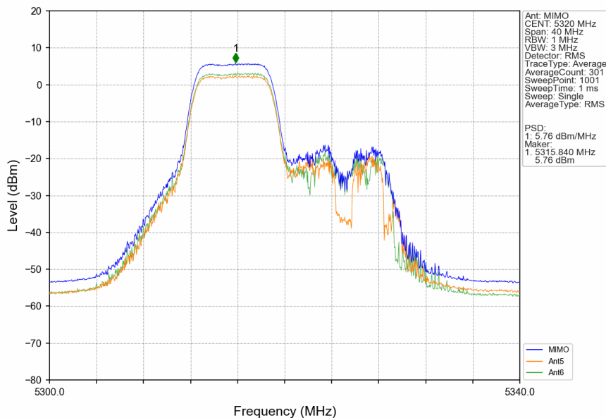
802.11be(EHT20)_HCH_5320MHz_26+52_/_MIMO_NTNV
