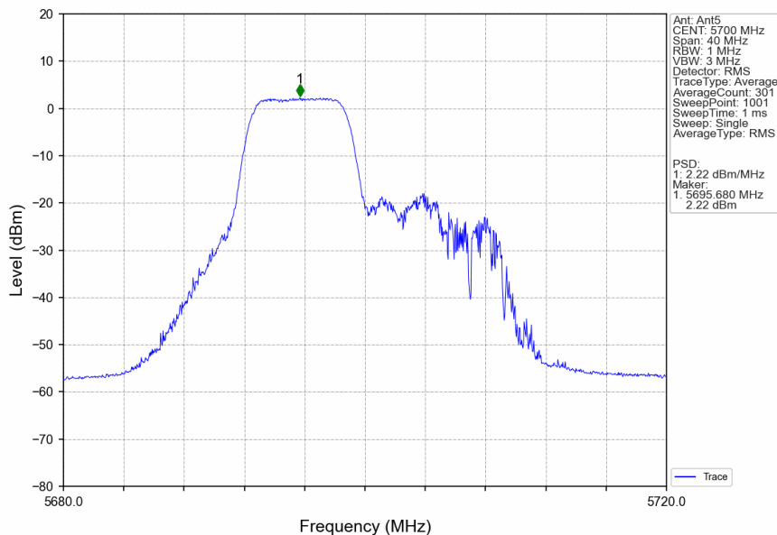
802.11be(EHT20)_HCH_5700MHz_26+52_/_Ant5_NTNV
