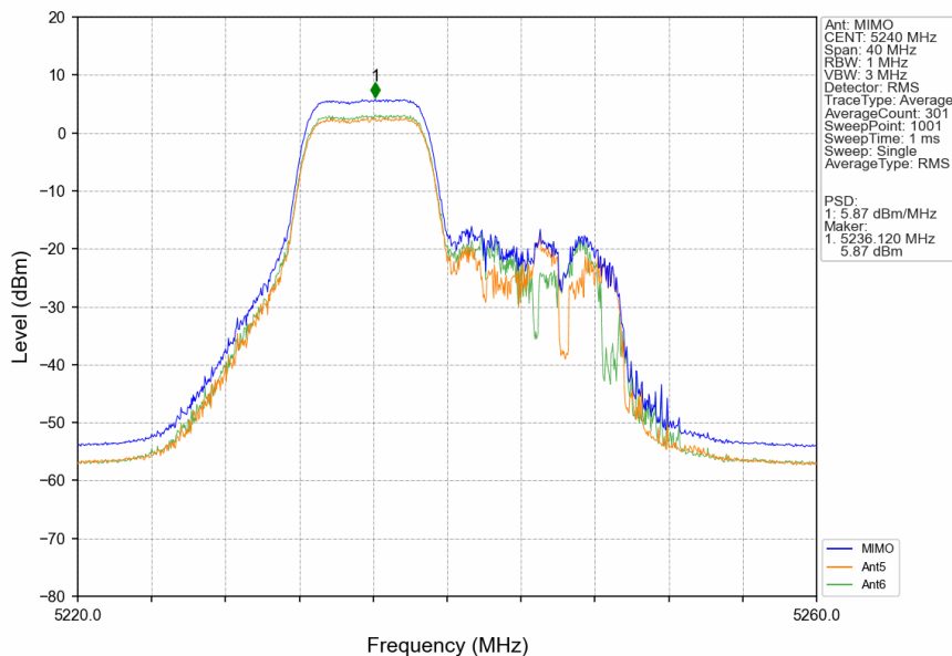
802.11be(EHT20)_HCH_5240MHz_26+52_/_MIMO_NTNV
