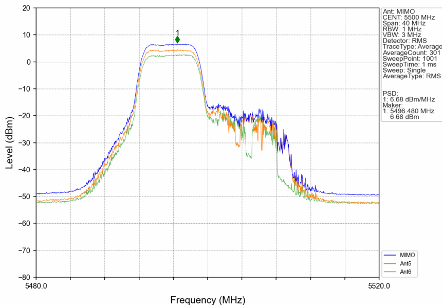
802.11be(EHT20)_LCH_5500MHz_26+52_/_MIMO_NTNV
