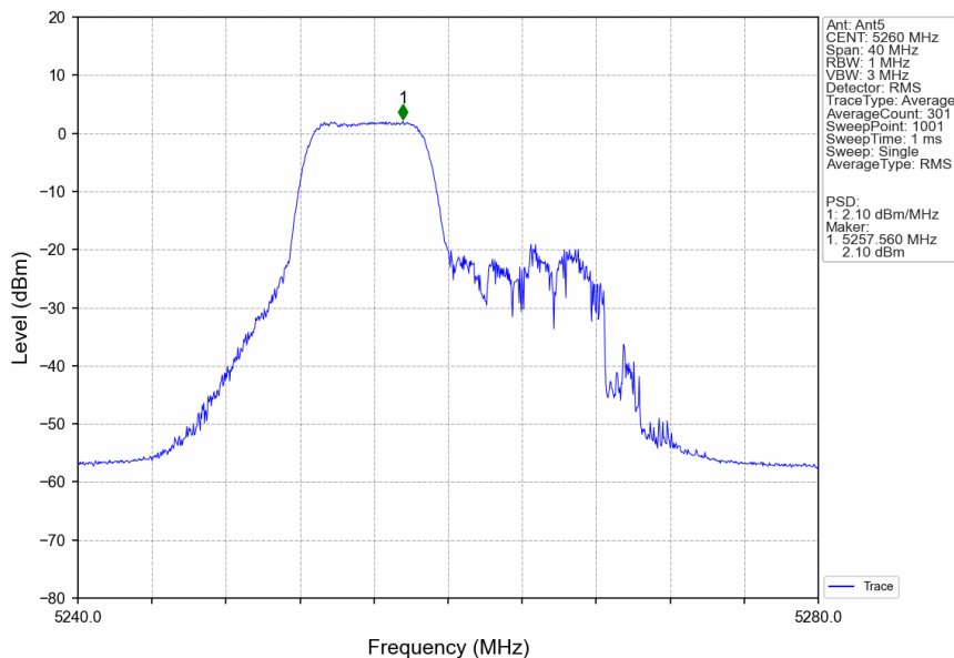
802.11be(EHT20)_LCH_5260MHz_26+52_/_Ant5_NTNV
