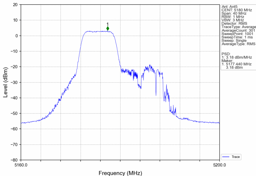
802.11be(EHT20)_LCH_5180MHz_26+52_/_Ant5_NTNV
