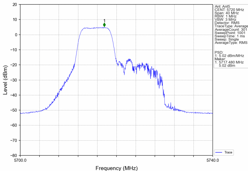
802.11be(EHT20)_HCH_5720MHz_26+52_/_Ant5_NTNV
