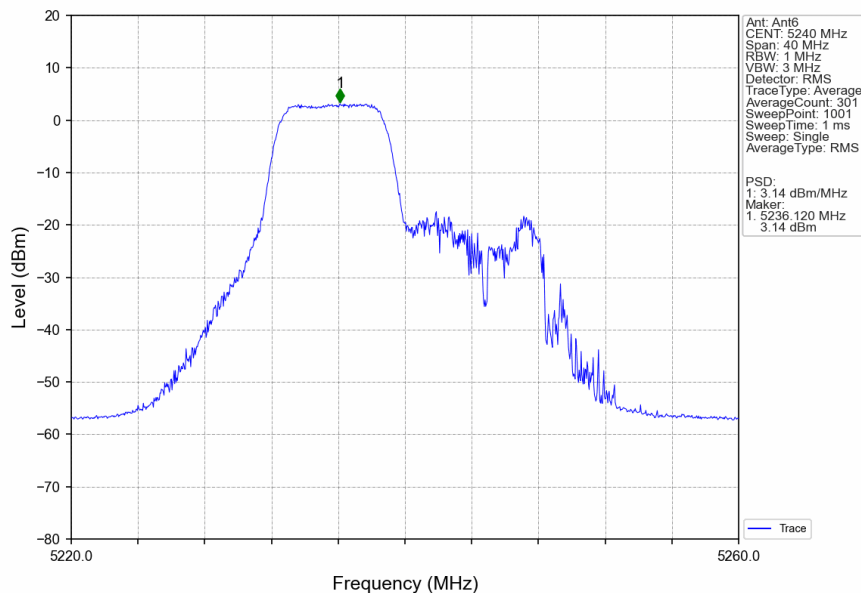
802.11be(EHT20)_HCH_5240MHz_26+52_/_Ant6_NTNV
