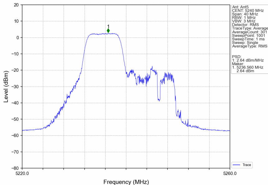
802.11be(EHT20)_HCH_5240MHz_26+52_/_Ant5_NTNV
