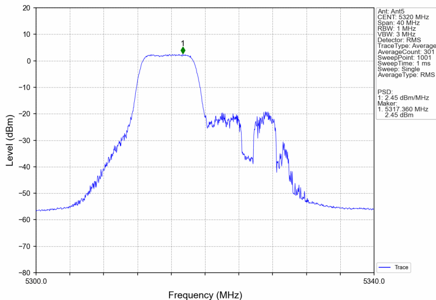
802.11be(EHT20)_HCH_5320MHz_26+52_/_Ant5_NTNV
