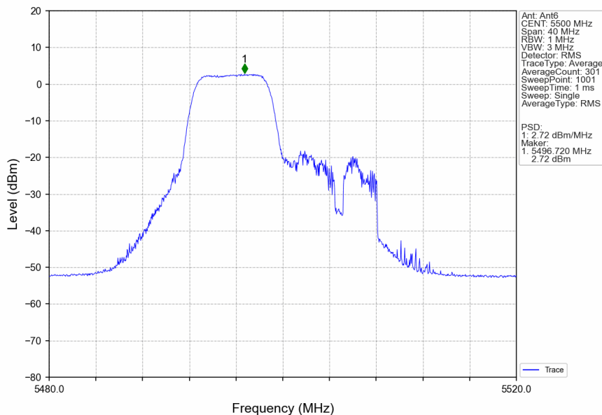
802.11be(EHT20)_LCH_5500MHz_26+52_/_Ant6_NTNV
