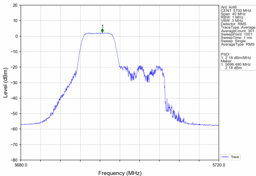
802.11be(EHT20)_HCH_5700MHz_26+52_/_Ant6_NTNV
