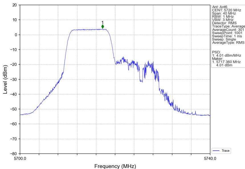
802.11ax(HEW20)_HCH_5720MHz_RU106_Left_Ant6_NTNV
