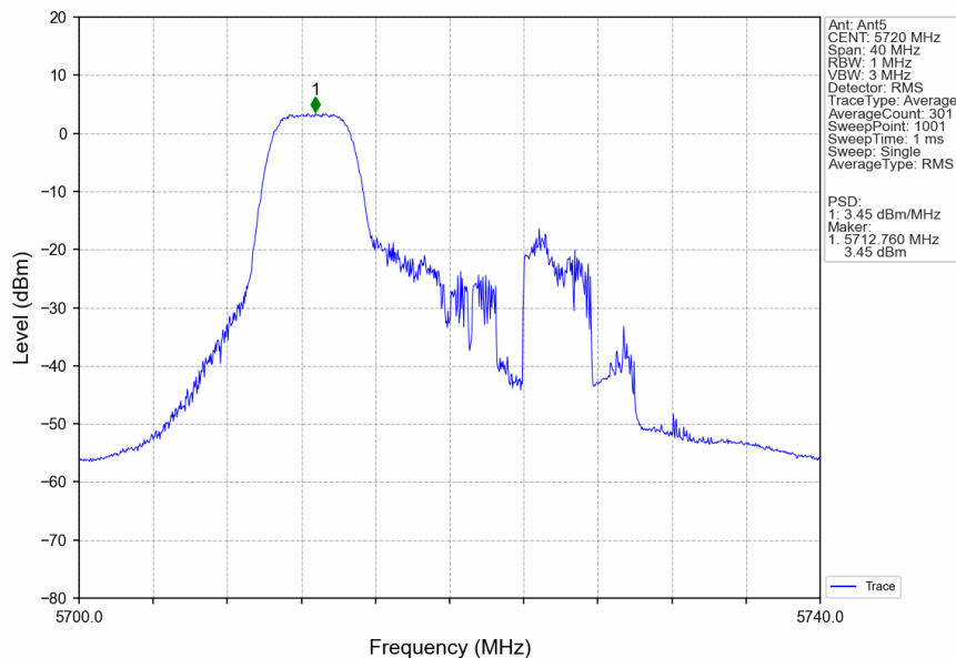
802.11ax(HEW20)_HCH_5720MHz_RU52_Left_Ant5_NTNV
