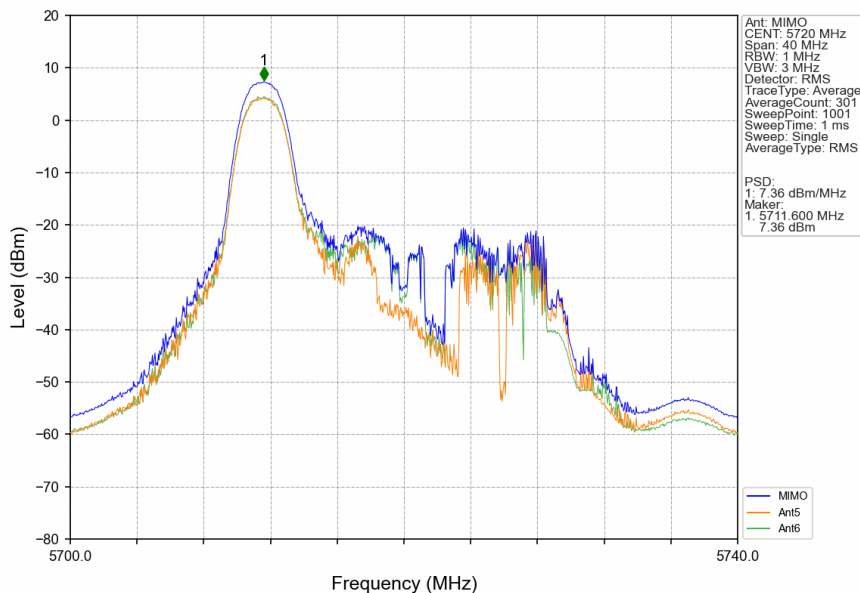
802.11ax(HEW20)_HCH_5720MHz_RU26_Left_MIMO_NTNV
