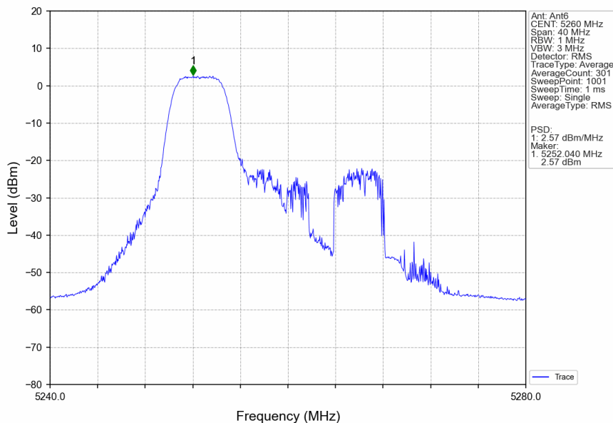
802.11ax(HEW20)_LCH_5260MHz_RU52_Left_Ant6_NTNV
