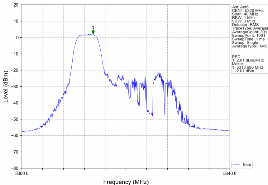
802.11ax(HEW20)_HCH_5320MHz_RU52_Left_Ant6_NTNV
