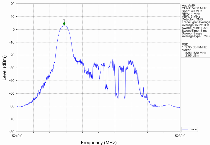
802.11ax(HEW20)_LCH_5260MHz_RU26_Left_Ant6_NTNV
