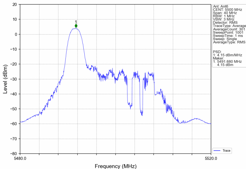
802.11ax(HEW20)_LCH_5500MHz_RU26_Left_Ant6_NTNV
