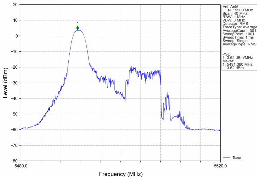
802.11ax(HEW20)_LCH_5500MHz_RU26_Left_Ant5_NTNV
