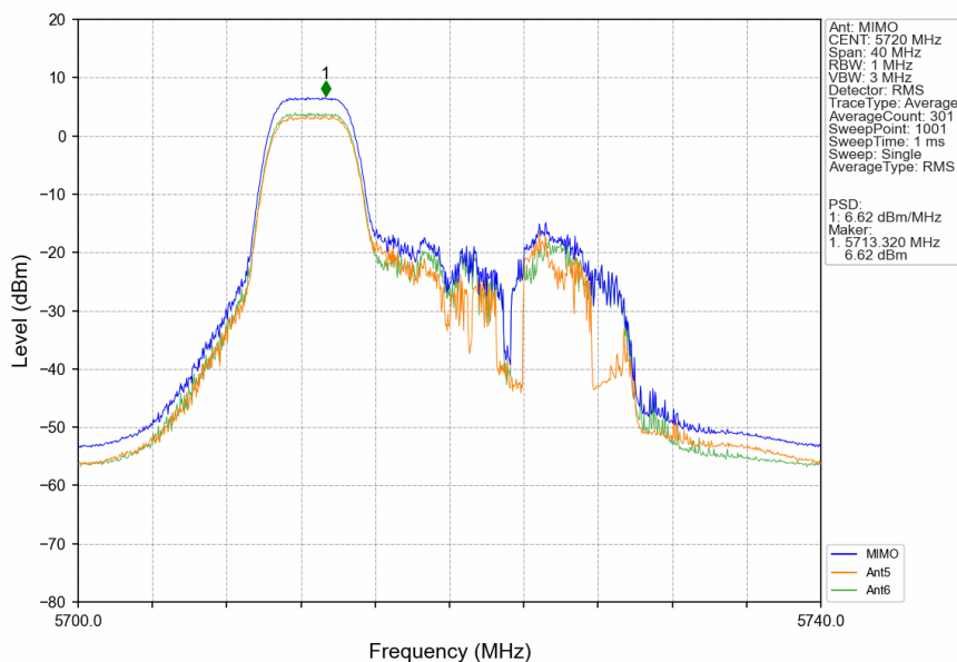
802.11ax(HEW20)_HCH_5720MHz_RU52_Left_MIMO_NTNV
