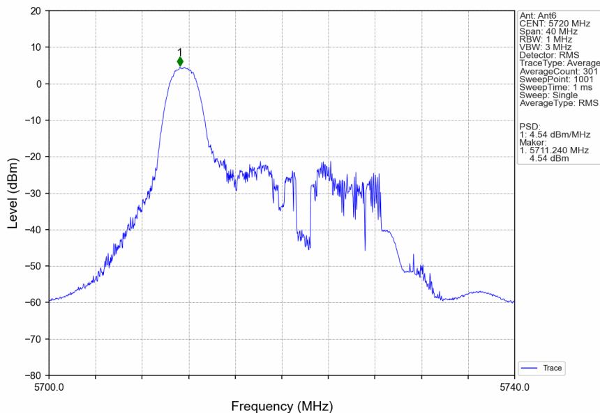
802.11ax(HEW20)_HCH_5720MHz_RU26_Left_Ant6_NTNV
