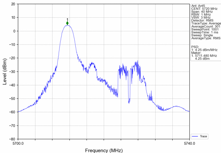
802.11ax(HEW20)_HCH_5720MHz_RU26_Left_Ant5_NTNV
