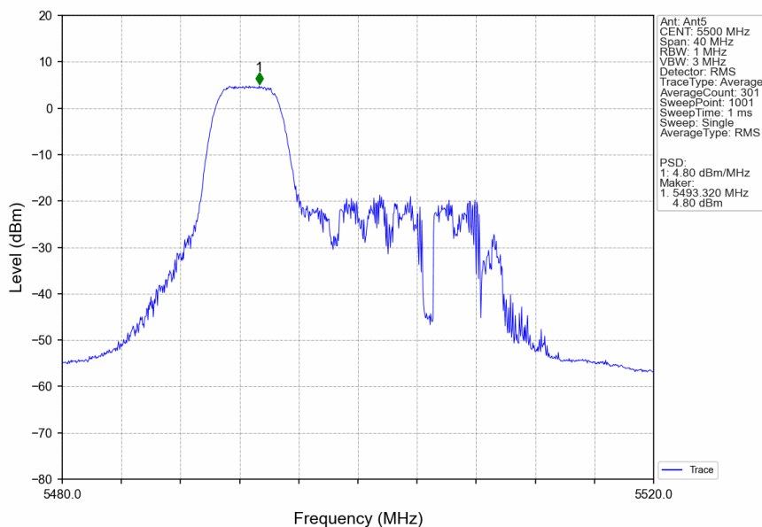
802.11ax(HEW20)_LCH_5500MHz_RU52_Left_Ant5_NTNV
