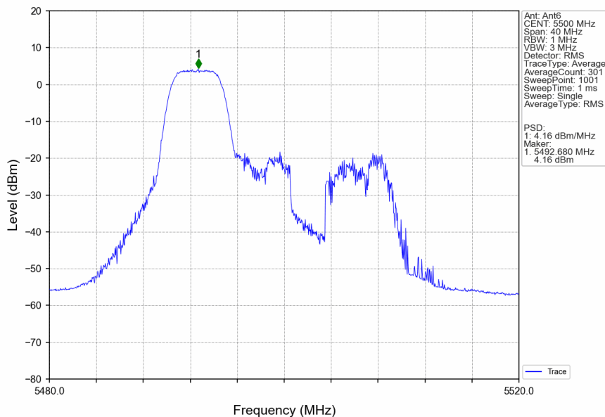
802.11ax(HEW20)_LCH_5500MHz_RU52_Left_Ant6_NTNV
