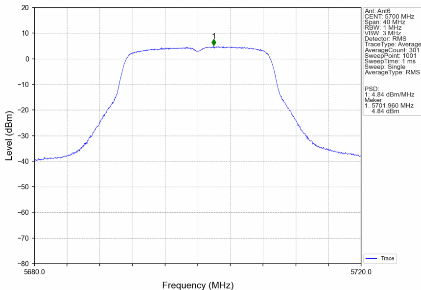
802.11ac(VHT20)_HCH_5700MHz_Ant6_NTNV
