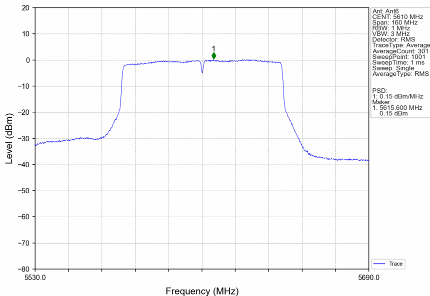
802.11ac(VHT80)_HCH_5610MHz_Ant6_NTNV
