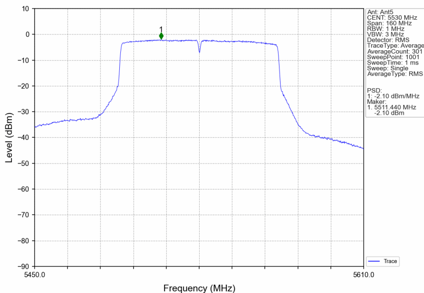
802.11ac(VHT80)_LCH_5530MHz_Ant5_NTNV
