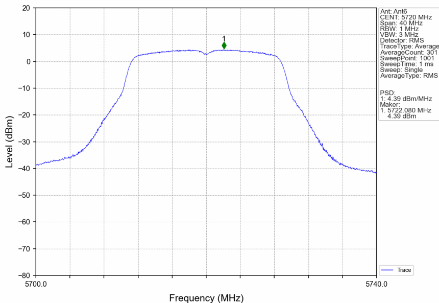
802.11ac(VHT20)_HCH_5720MHz_Ant6_NTNV
