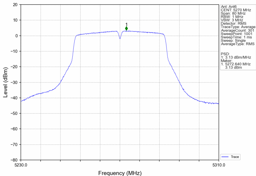
802.11ac(VHT40)_LCH_5270MHz_Ant6_NTNV
