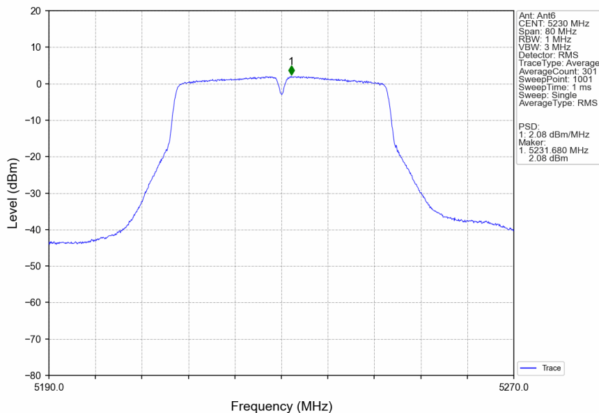
802.11ac(VHT40)_HCH_5230MHz_Ant6_NTNV
