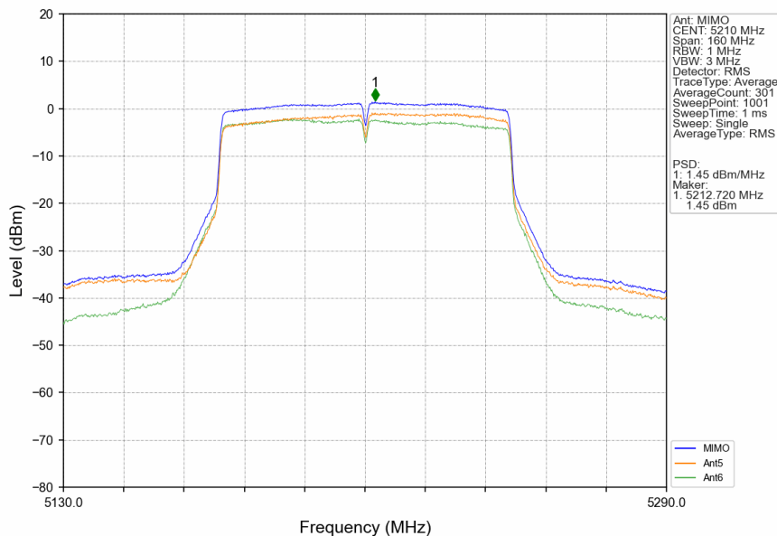
802.11ac(VHT80)_MCH_5210MHz_MIMO_NTNV
