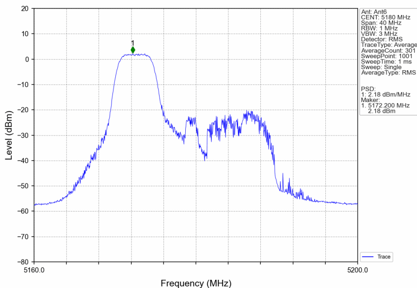
802.11ax(HEW20)_LCH_5180MHz_RU52_Left_Ant6_NTNV
