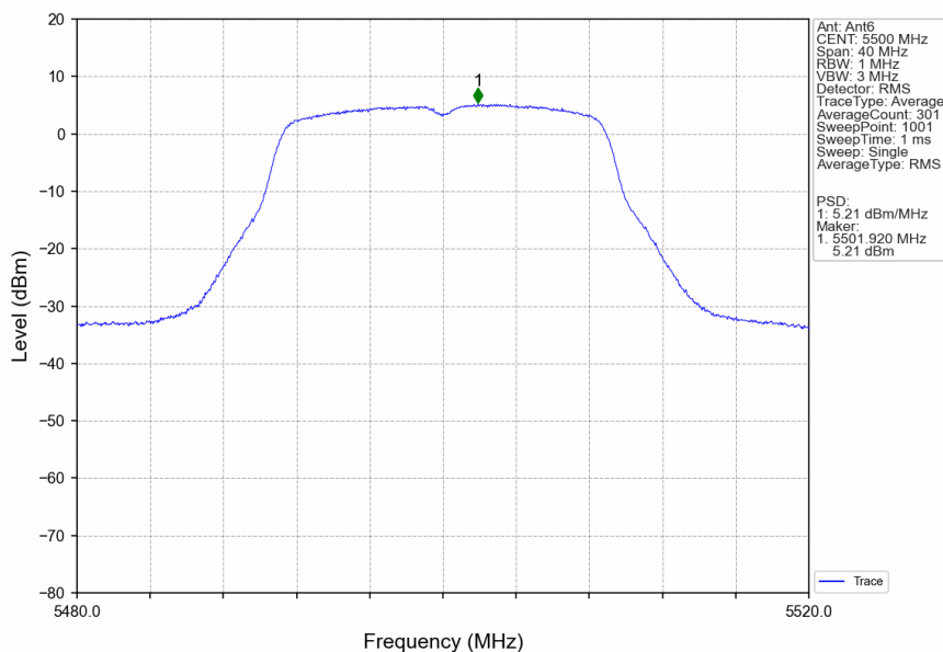
802.11ac(VHT20)_LCH_5500MHz_Ant6_NTNV
