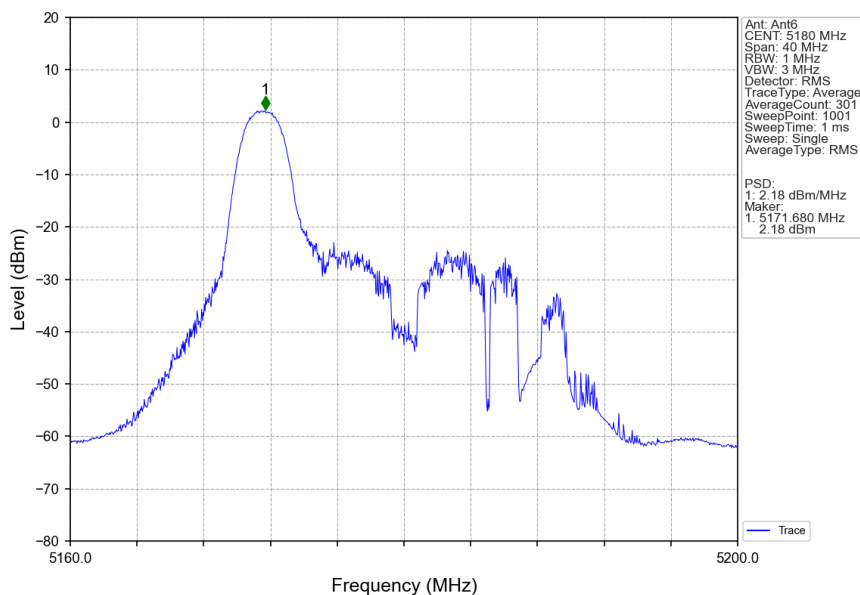
802.11ax(HEW20)_LCH_5180MHz_RU26_Left_Ant6_NTNV
