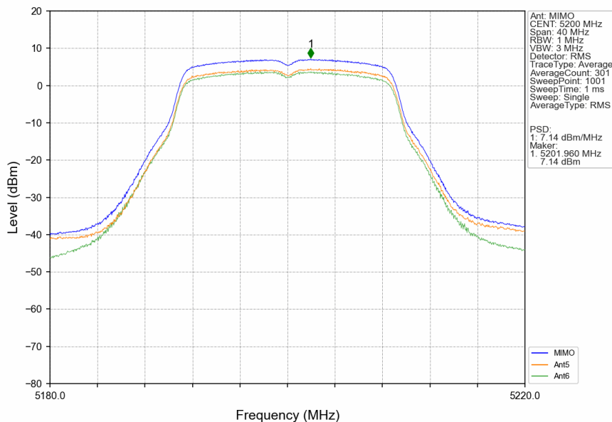
802.11n(HT20)_MCH_5200MHz_MIMO_NTNV
