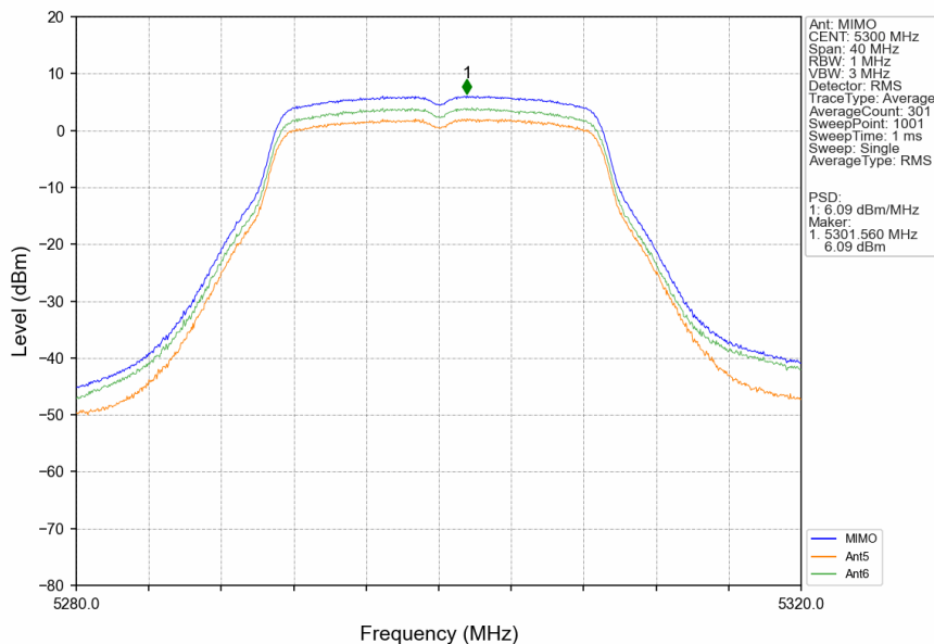
802.11n(HT20)_MCH_5300MHz_MIMO_NTNV
