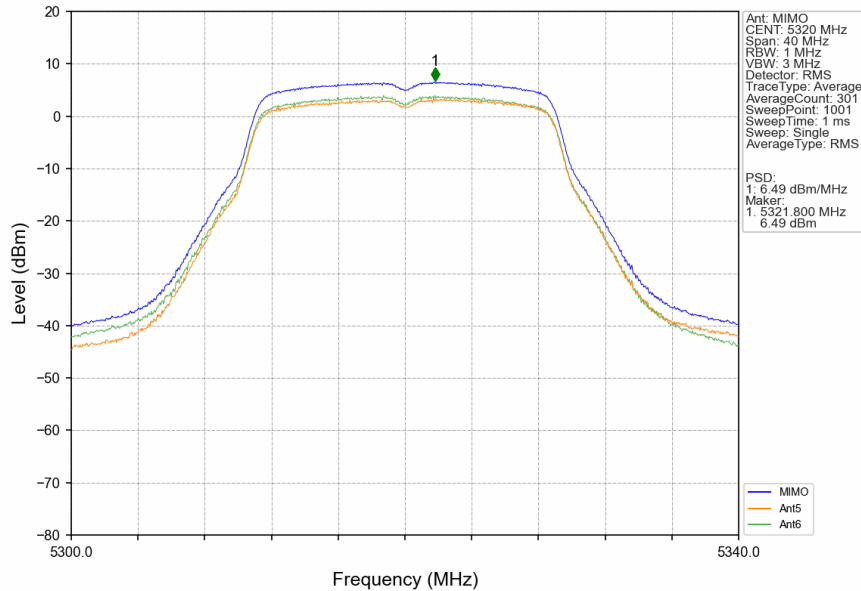
802.11n(HT20)_HCH_5320MHz_MIMO_NTNV
