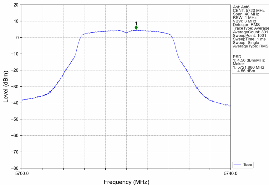
802.11n(HT20)_HCH_5720MHz_Ant6_NTNV
