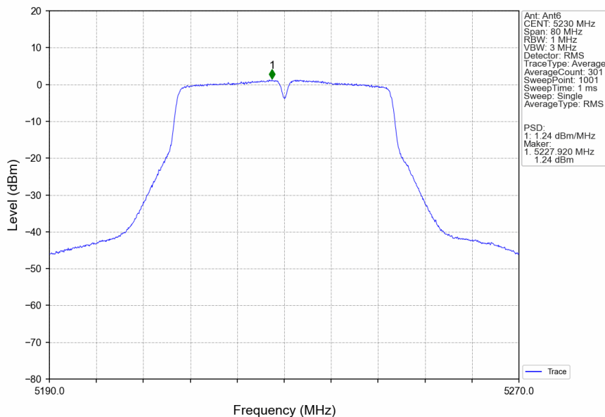
802.11n(HT40)_HCH_5230MHz_Ant6_NTNV
