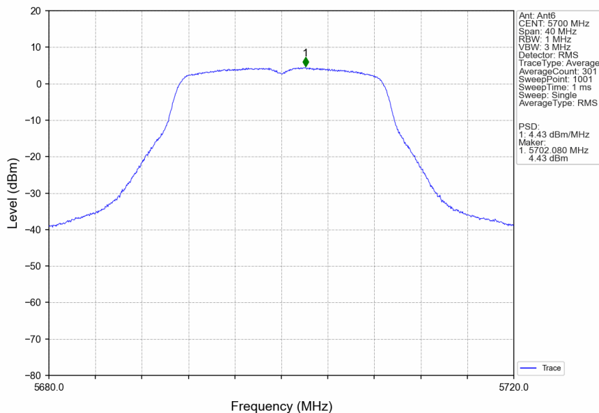
802.11n(HT20)_HCH_5700MHz_Ant6_NTNV
