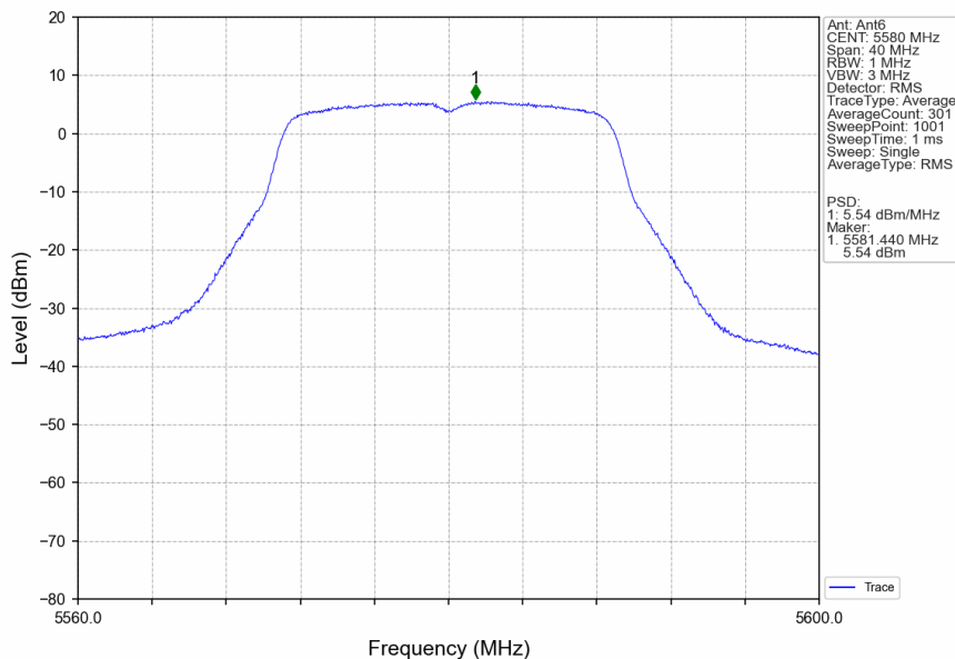
802.11n(HT20)_MCH_5580MHz_Ant6_NTNV
