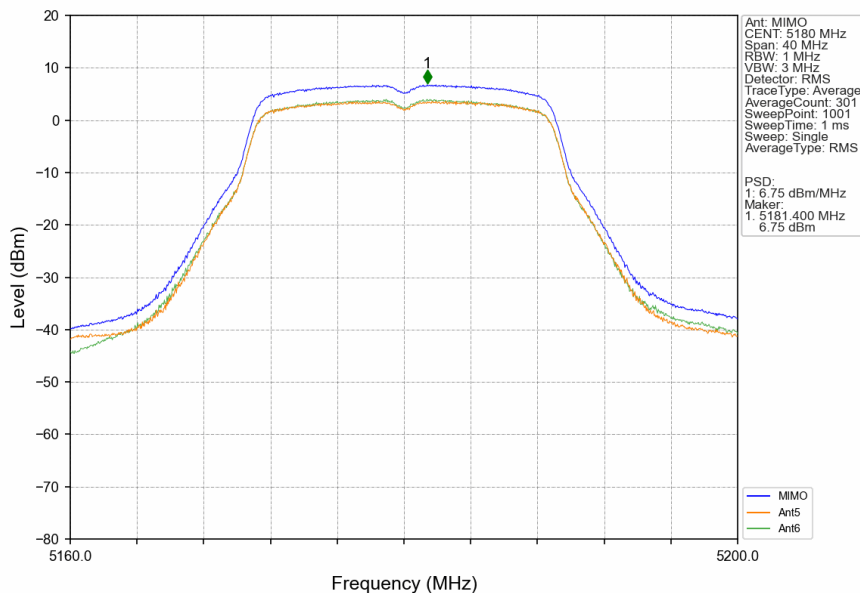
802.11n(HT20)_LCH_5180MHz_MIMO_NTNV
