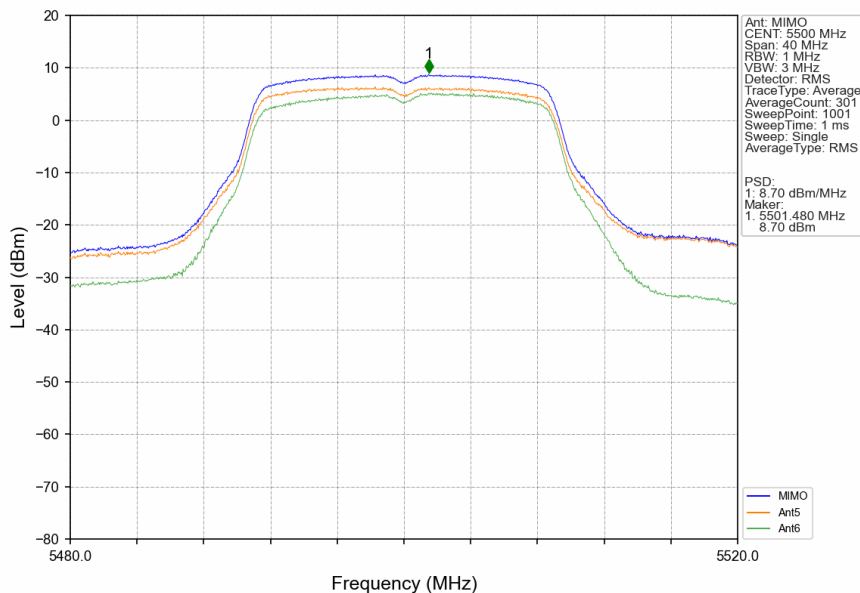
802.11n(HT20)_LCH_5500MHz_MIMO_NTNV
