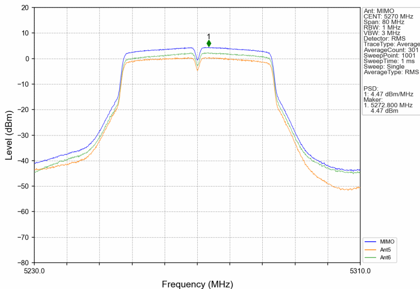
802.11n(HT40)_LCH_5270MHz_MIMO_NTNV
