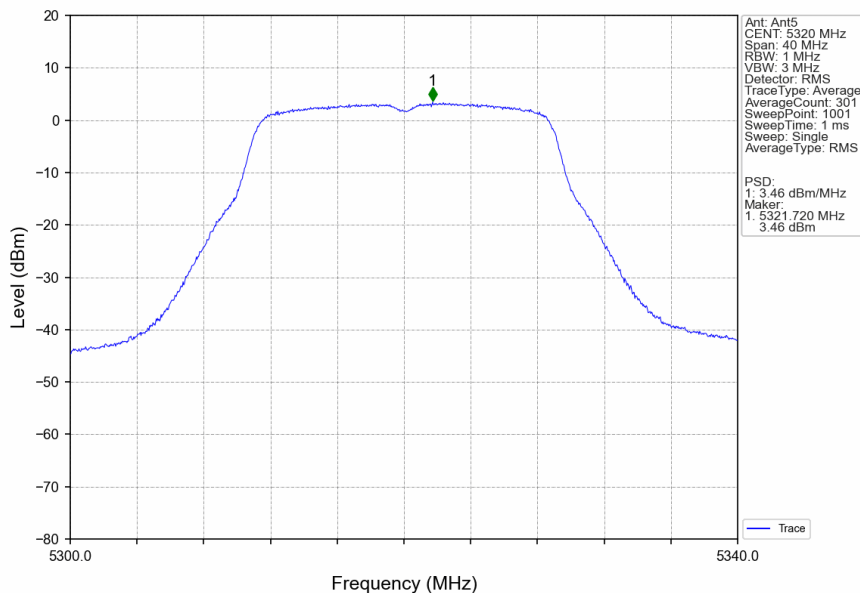
802.11n(HT20)_HCH_5320MHz_Ant5_NTNV
