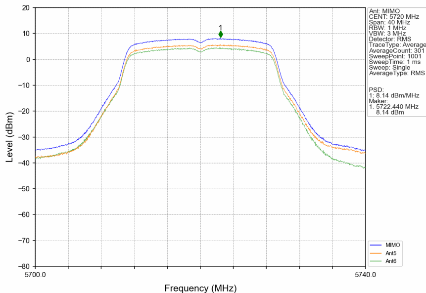
802.11n(HT20)_HCH_5720MHz_MIMO_NTNV
