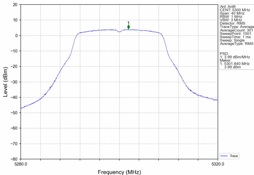
802.11n(HT20)_MCH_5300MHz_Ant6_NTNV
