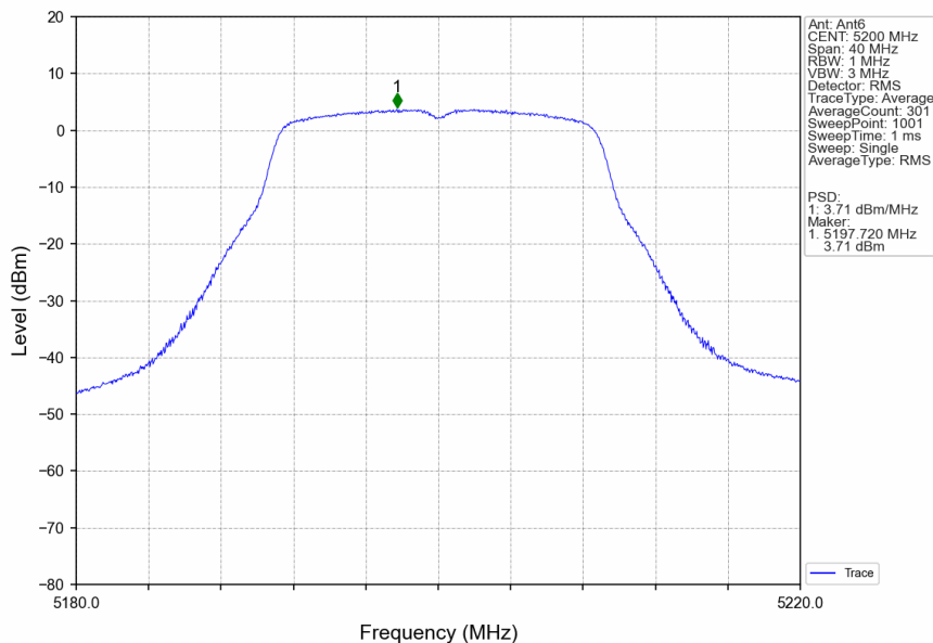
802.11n(HT20)_MCH_5200MHz_Ant6_NTNV
