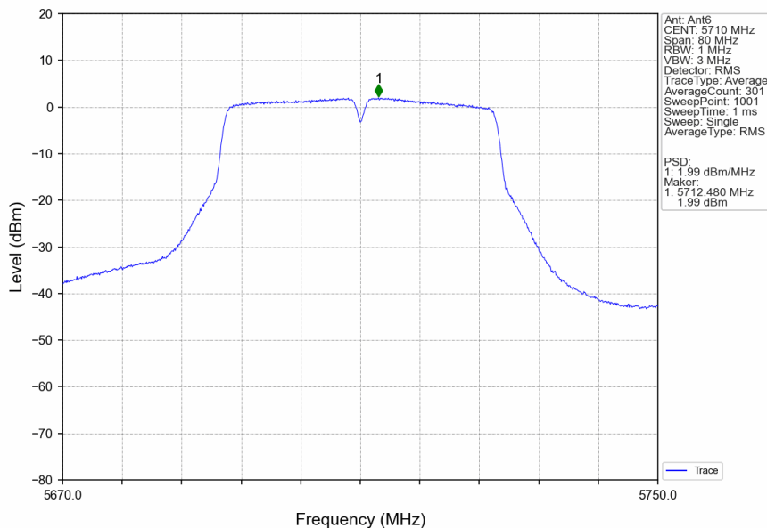
802.11n(HT40)_HCH_5710MHz_Ant6_NTNV
