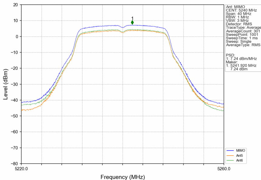
802.11n(HT20)_HCH_5240MHz_MIMO_NTNV
