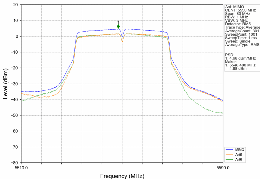
802.11n(HT40)_MCH_5550MHz_MIMO_NTNV
