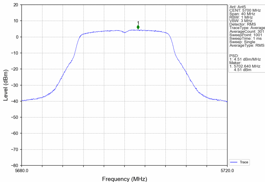
802.11n(HT20)_HCH_5700MHz_Ant5_NTNV
