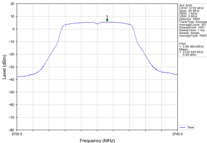
802.11n(HT20)_HCH_5720MHz_Ant5_NTNV
