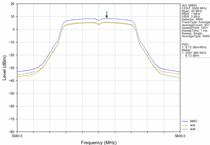
802.11n(HT20)_MCH_5580MHz_MIMO_NTNV
