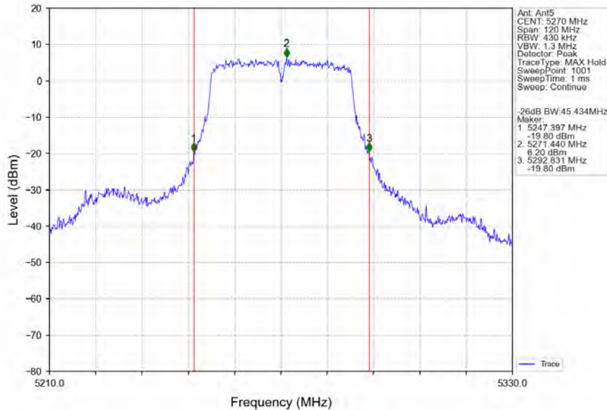
802.11ac(VHT40) LCH 5270MHz Ant5 NTN
