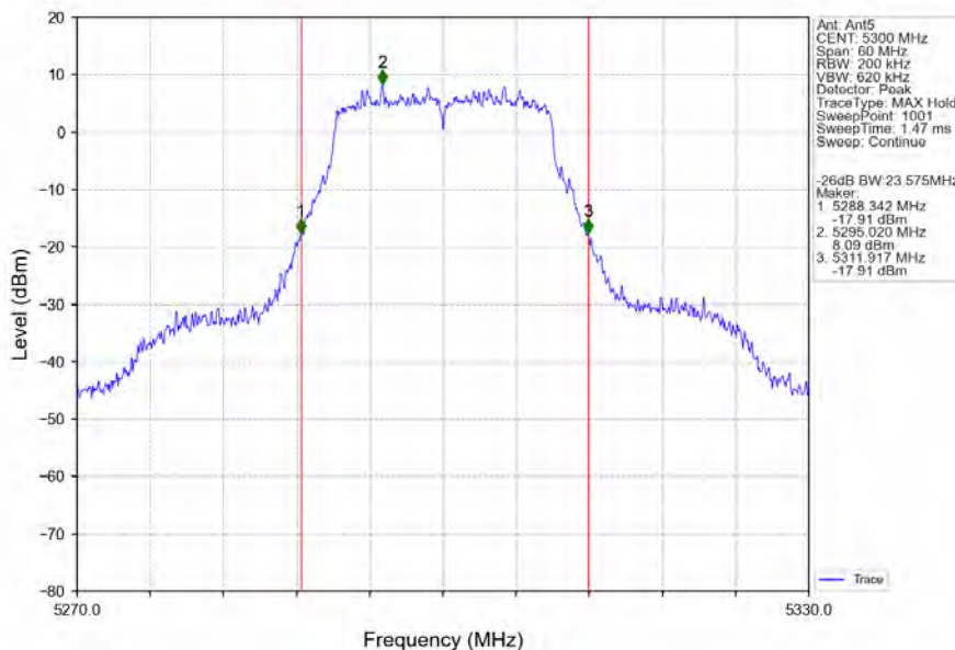
802.11n(HT20) MCH_5300MHz_Ant5_NTNV
