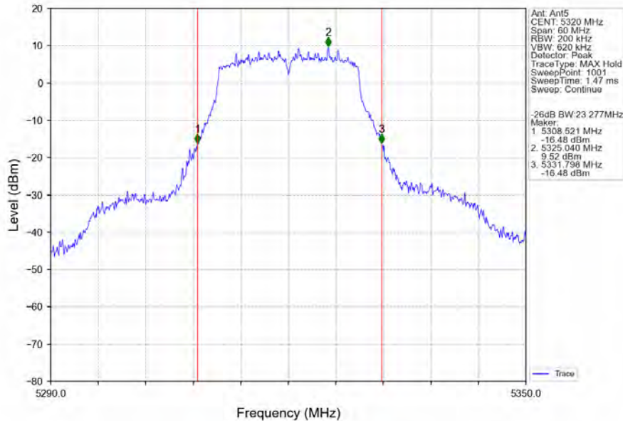
802.11n(HT20) HCH 5320MHz Ant5 NTNV
