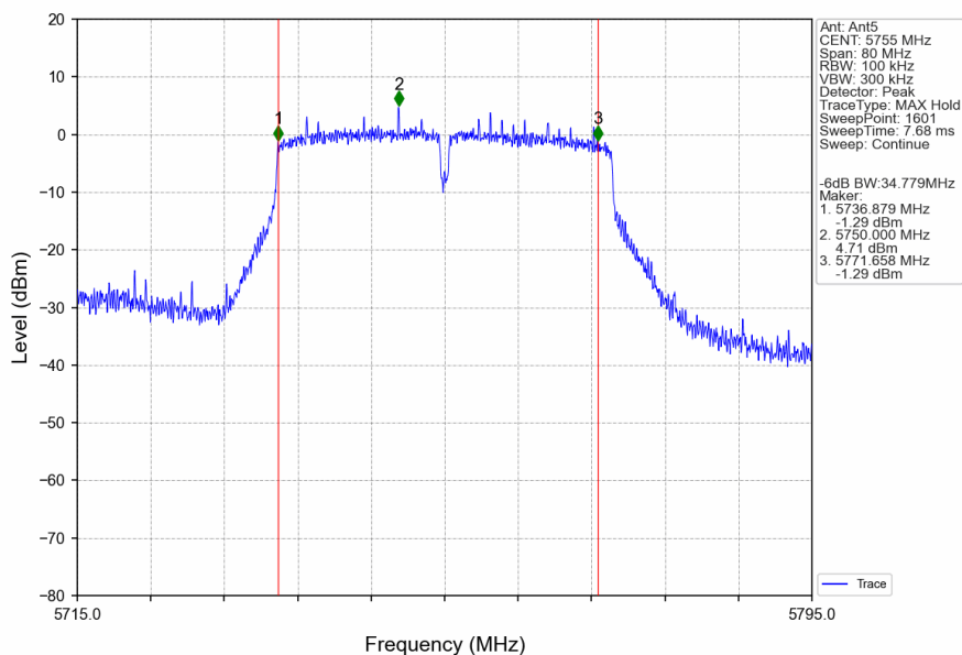
802.11ac(VHT40)_LCH_5755MHz_Ant5_NTNV
