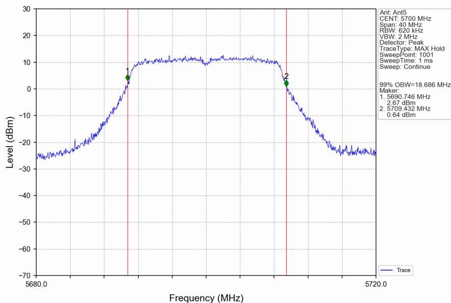
802.11n(HT20)_HCH_5700MHz_Ant5_NTNV
