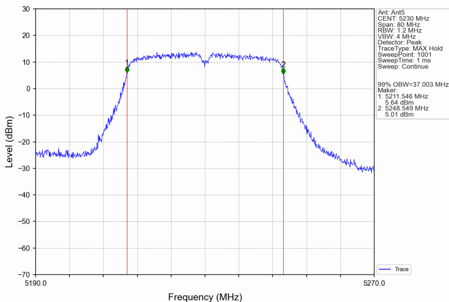
802.11n(HT40)_HCH_5230MHz_Ant5_NTNV
