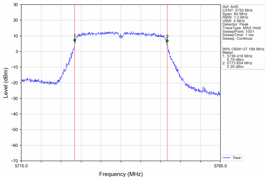
802.11ac(VHT40)_LCH_5755MHz_Ant5_NTNV
