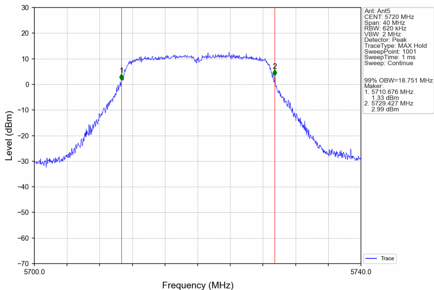
802.11n(HT20)_HCH_5720MHz_Ant5_NTNV
