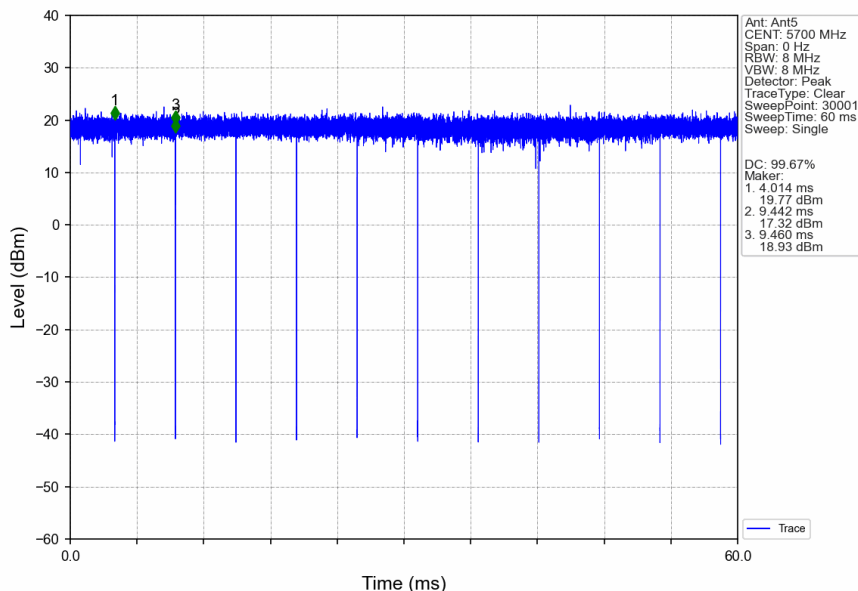
802.11ac(VHT20)_HCH_5700MHz_Ant5_NTNV
