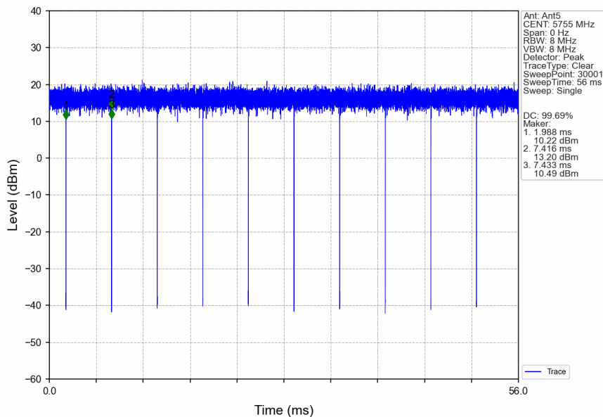
802.11ac(VHT40)_LCH_5755MHz_Ant5_NTNV
