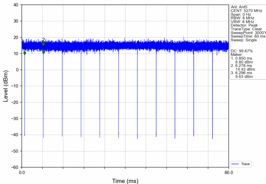
802.11ac(VHT40)_LCH_5270MHz_Ant5_NTNV
