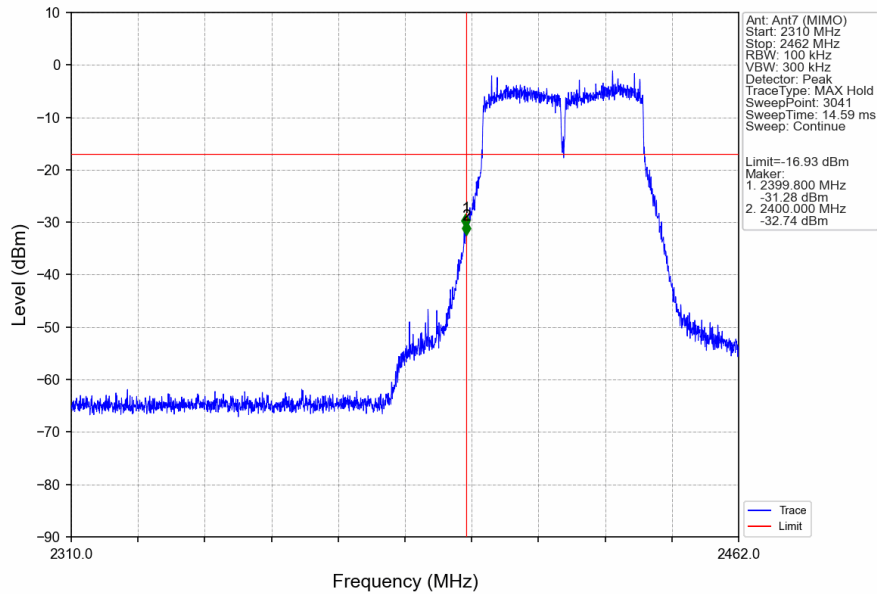
802.11n(HT40)_LCH_2422MHz_Ant7 (MIMO)_NTNV
