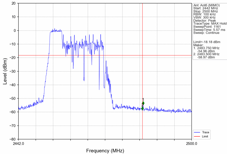
802.11ax(HEW20)_HCH_2462MHz_RU52_Left_Ant6 (MIMO)_NTNV
