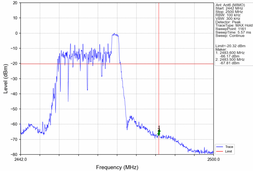
802.11ax(HEW20)_HCH_2462MHz_RU26_Right_Ant6 (MIMO)_NTNV
