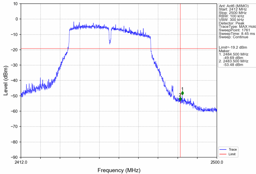
802.11n(HT40)_HCH_2452MHz_Ant6 (MIMO)_NTNV
