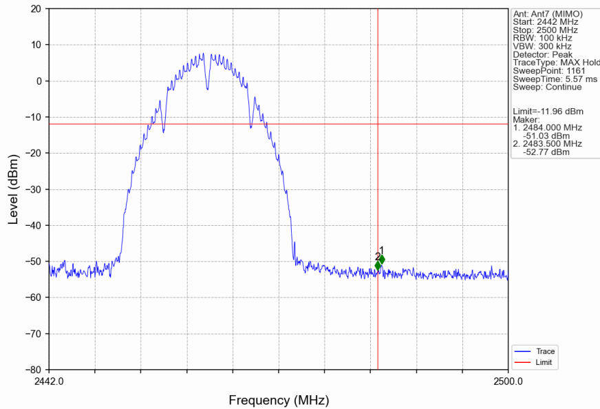
802.11b_HCH_2462MHz_Ant7 (MIMO)_NTNV
