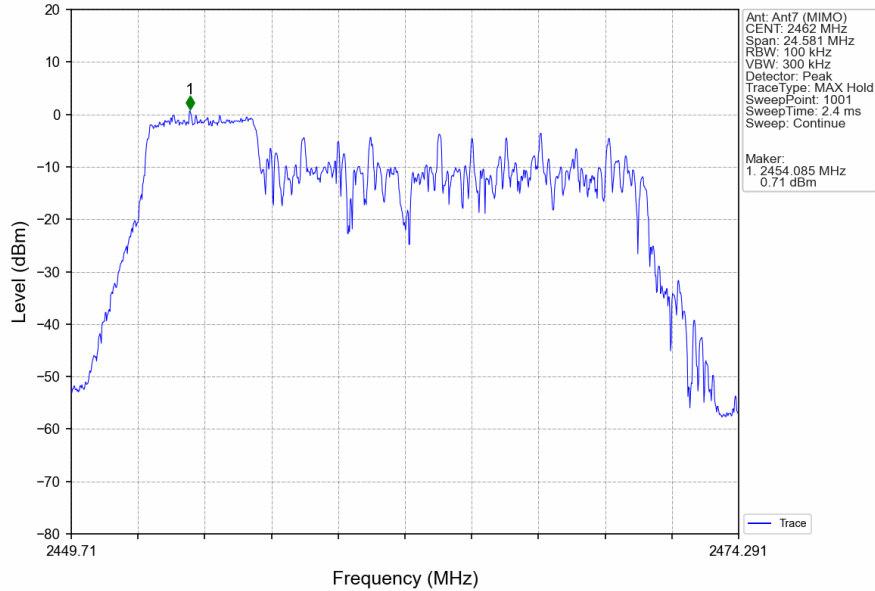
802.11ax(HEW20)_HCH_2462MHz_RU52_Left_Ant7 (MIMO)_NTNV
