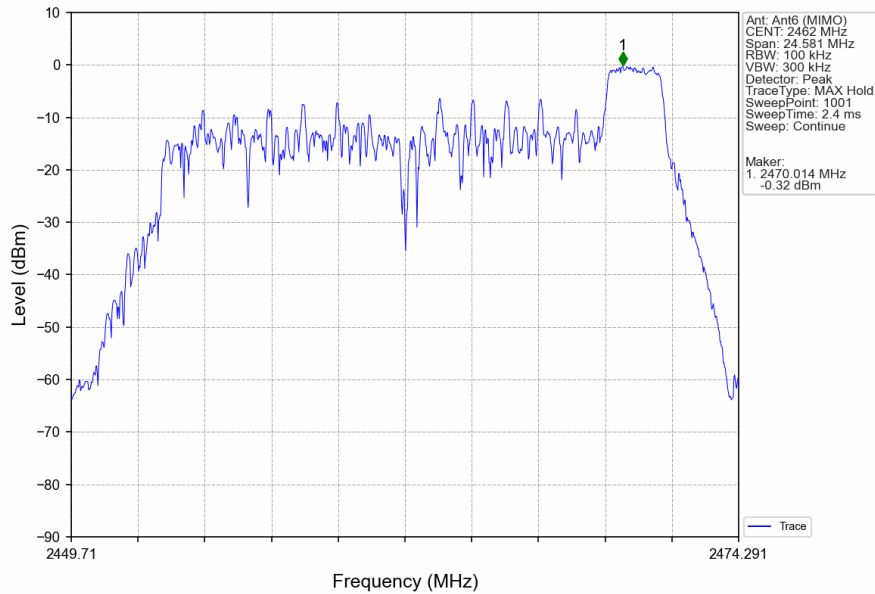
802.11ax(HEW20)_HCH_2462MHz_RU26_Right_Ant6 (MIMO)_NTNV
