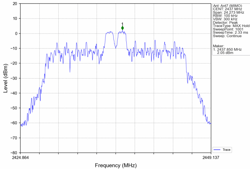
802.11ax(HEW20)_MCH_2437MHz_RU26_Mid_Ant7 (MIMO)_NTNV
