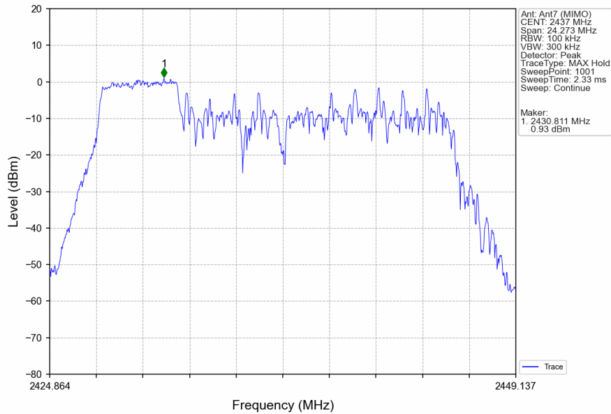
802.11ax(HEW20)_MCH_2437MHz_RU52_Left_Ant7 (MIMO)_NTNV
