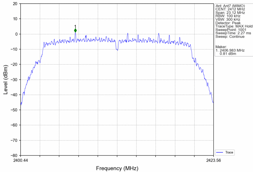
802.11ac(VHT20)_LCH_2412MHz_Ant7 (MIMO)_NTNV
