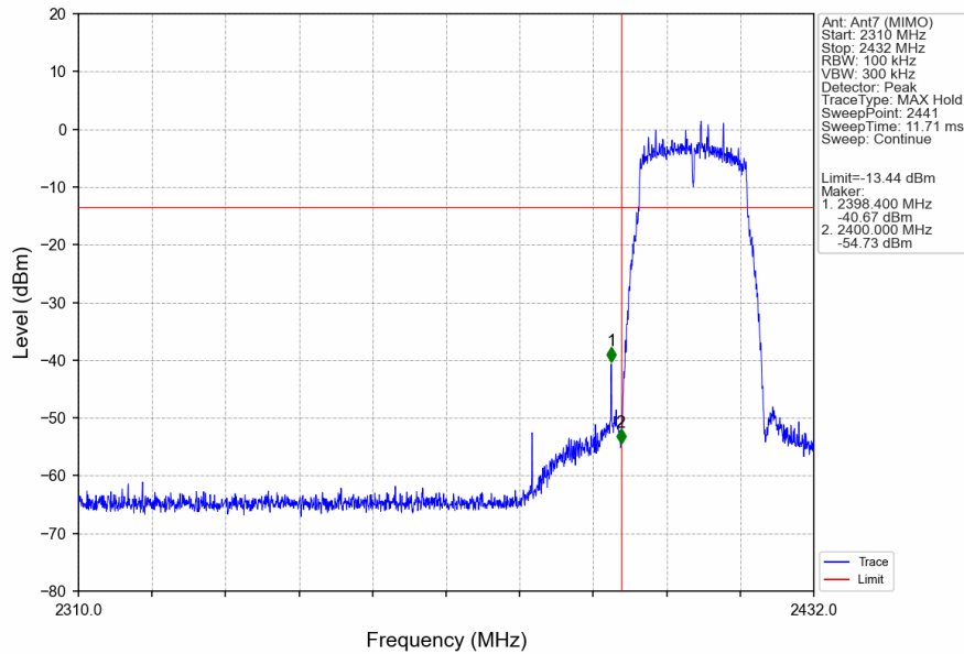
802.11n(HT20)_LCH_2412MHz_Ant7 (MIMO)_NTNV
