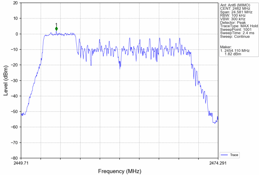
802.11ax(HEW20)_HCH_2462MHz_RU52_Left_Ant6 (MIMO)_NTNV
