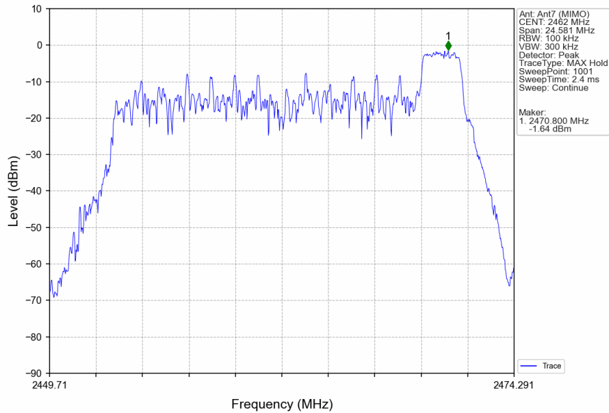
802.11ax(HEW20)_HCH_2462MHz_RU26_Right_Ant7 (MIMO)_NTNV
