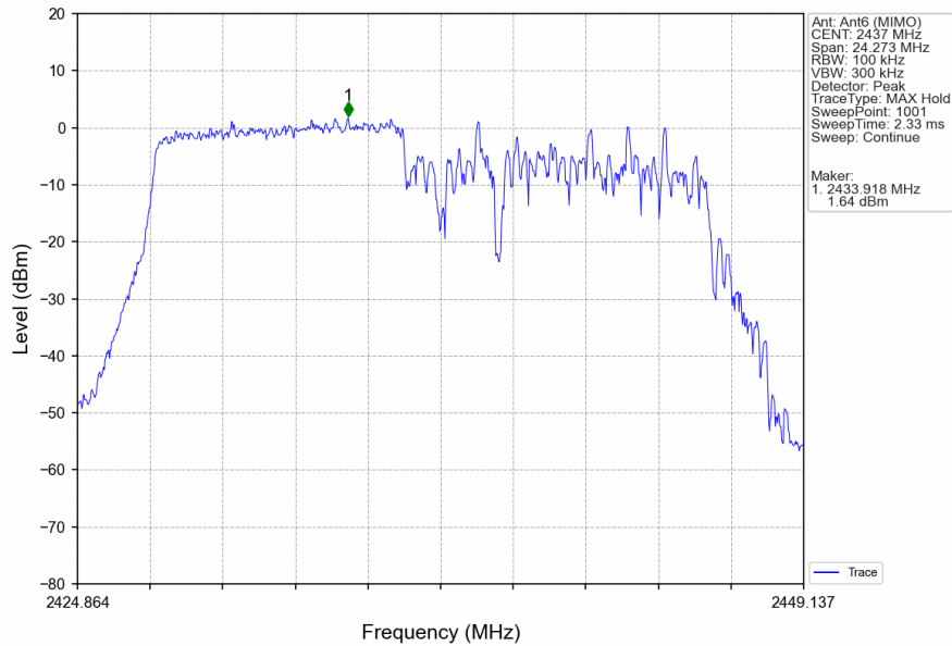
802.11ax(HEW20)_MCH_2437MHz_RU106_Left_Ant6 (MIMO)_NTNV
