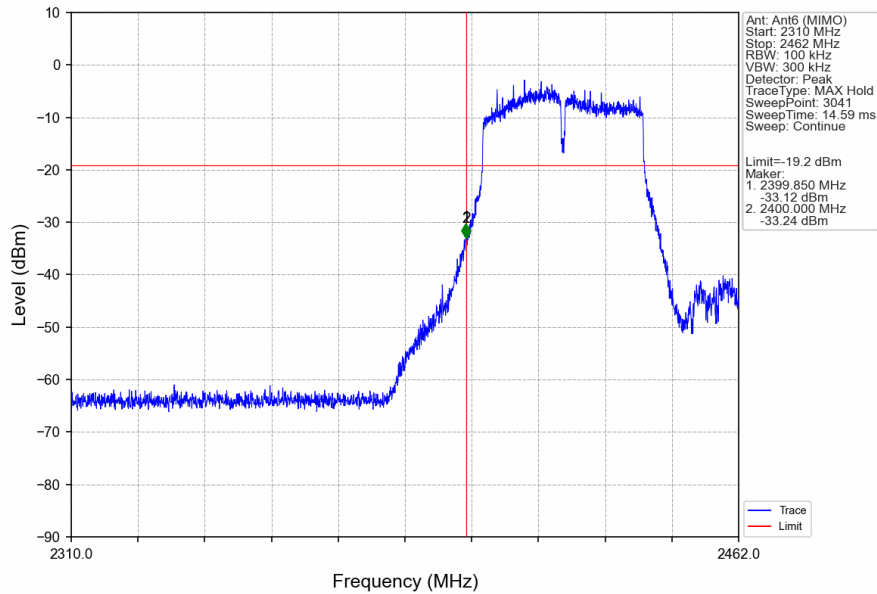
802.11n(HT40)_LCH_2422MHz_Ant6 (MIMO)_NTNV
