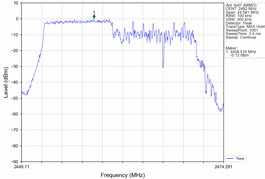
802.11ax(HEW20)_HCH_2462MHz_RU106_Left_Ant7 (MIMO)_NTNV
