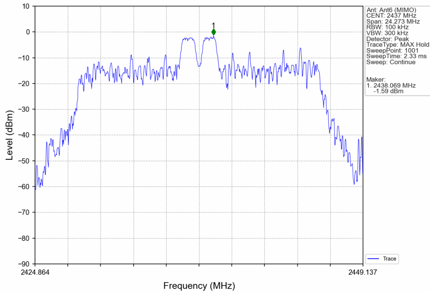
802.11ax(HEW20)_MCH_2437MHz_RU26_Mid_Ant6 (MIMO)_NTNV
