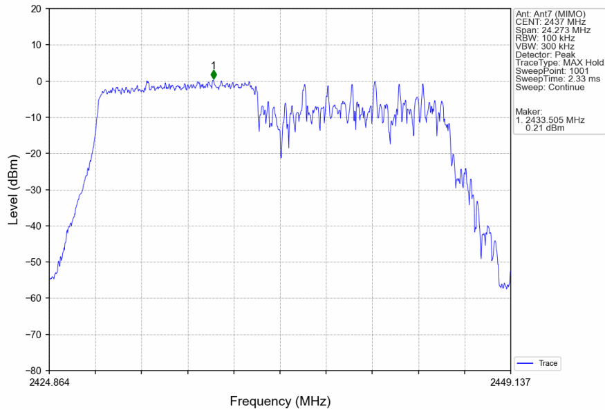
802.11ax(HEW20)_MCH_2437MHz_RU106_Left_Ant7 (MIMO)_NTNV
