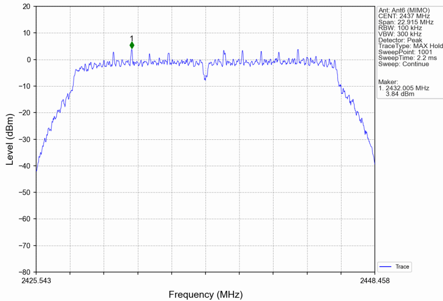
802.11n(HT20)_MCH_2437MHz_Ant6 (MIMO)_NTNV
