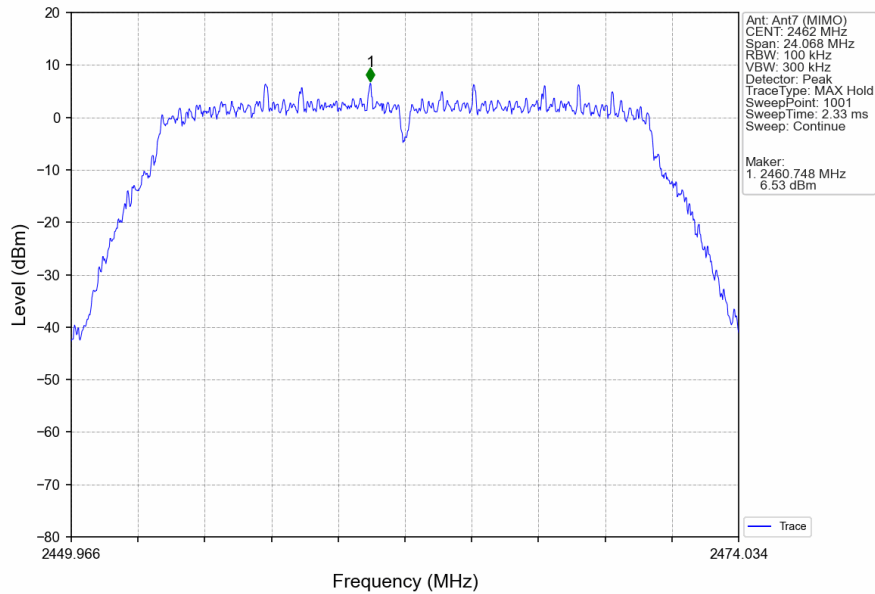
802.11n(HT20)_HCH_2462MHz_Ant7 (MIMO)_NTNV
