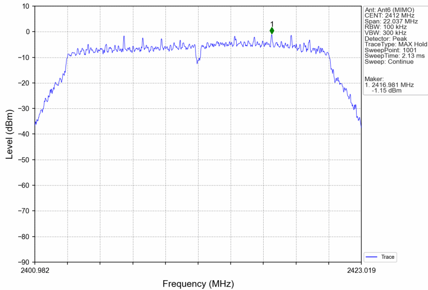
802.11n(HT20)_LCH_2412MHz_Ant6 (MIMO)_NTNV
