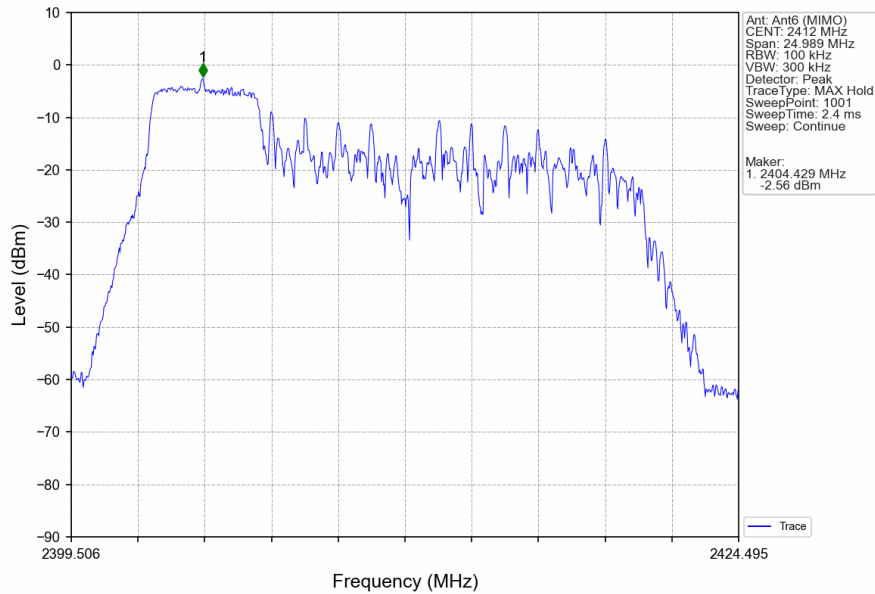
802.11ax(HEW20)_LCH_2412MHz_RU52_Left_Ant6 (MIMO)_NTNV
