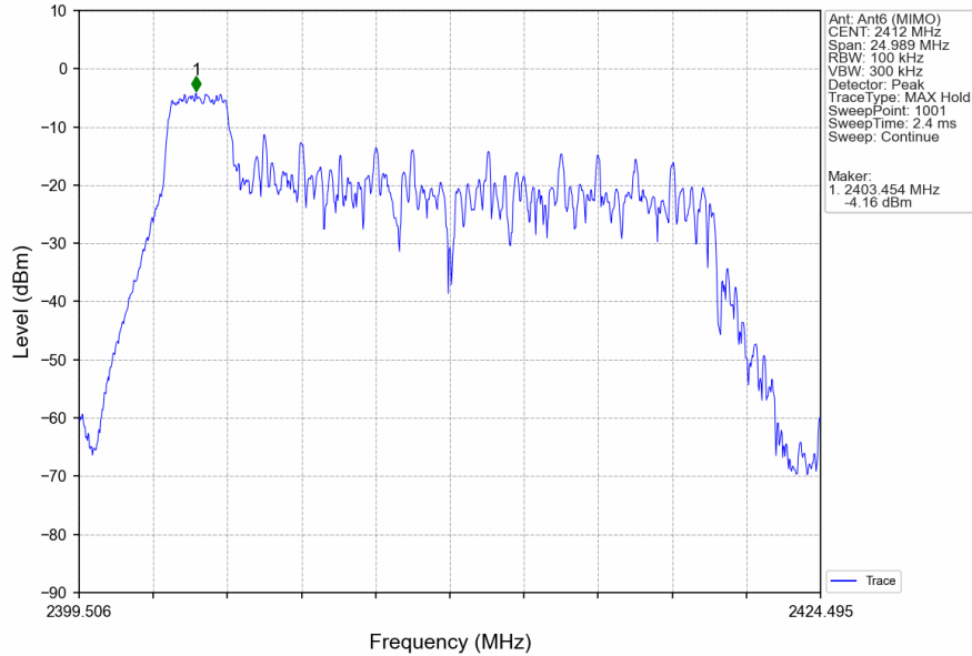
802.11ax(HEW20)_LCH_2412MHz_RU26_Left_Ant6 (MIMO)_NTNV
