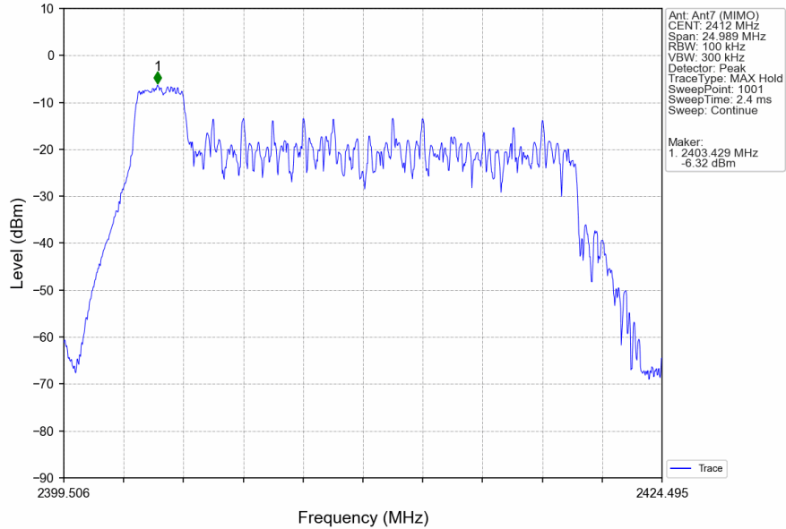
802.11ax(HEW20)_LCH_2412MHz_RU26_Left_Ant7 (MIMO)_NTNV
