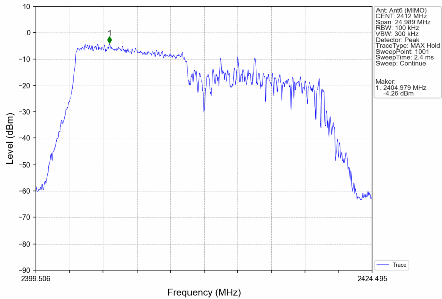
802.11ax(HEW20)_LCH_2412MHz_RU106_Left_Ant6 (MIMO)_NTNV
