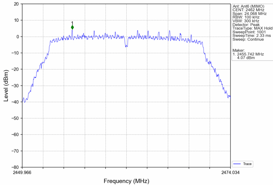
802.11n(HT20)_HCH_2462MHz_Ant6 (MIMO)_NTNV
