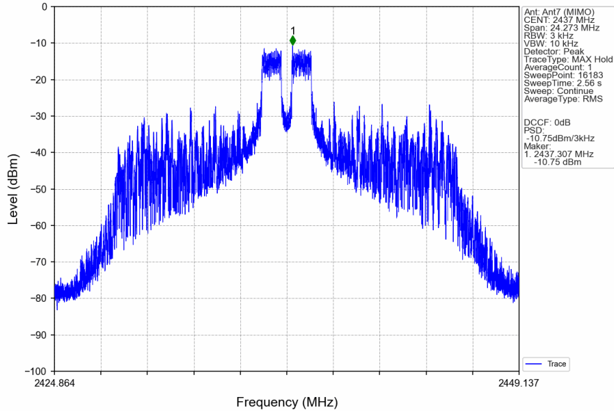
802.11ax(HEW20)_MCH_2437MHz_RU26_Mid_Ant7 (MIMO)_NTNV
