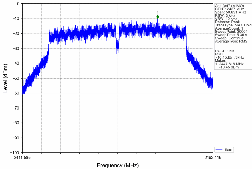
802.11n(HT40)_MCH_2437MHz_Ant7 (MIMO)_NTNV
