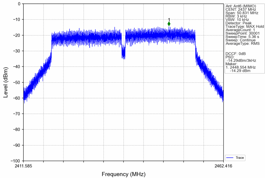
802.11n(HT40)_MCH_2437MHz_Ant6 (MIMO)_NTNV
