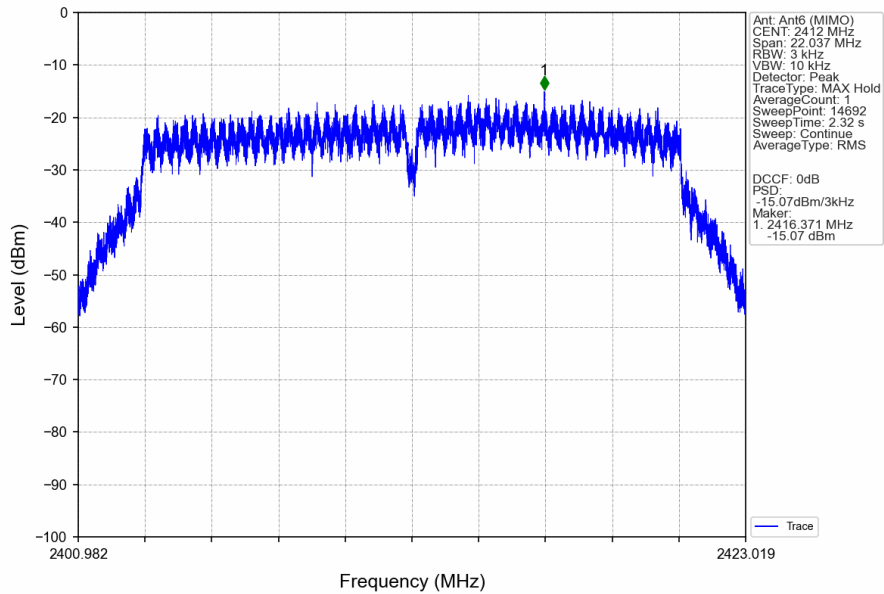
802.11n(HT20)_LCH_2412MHz_Ant6 (MIMO)_NTNV
