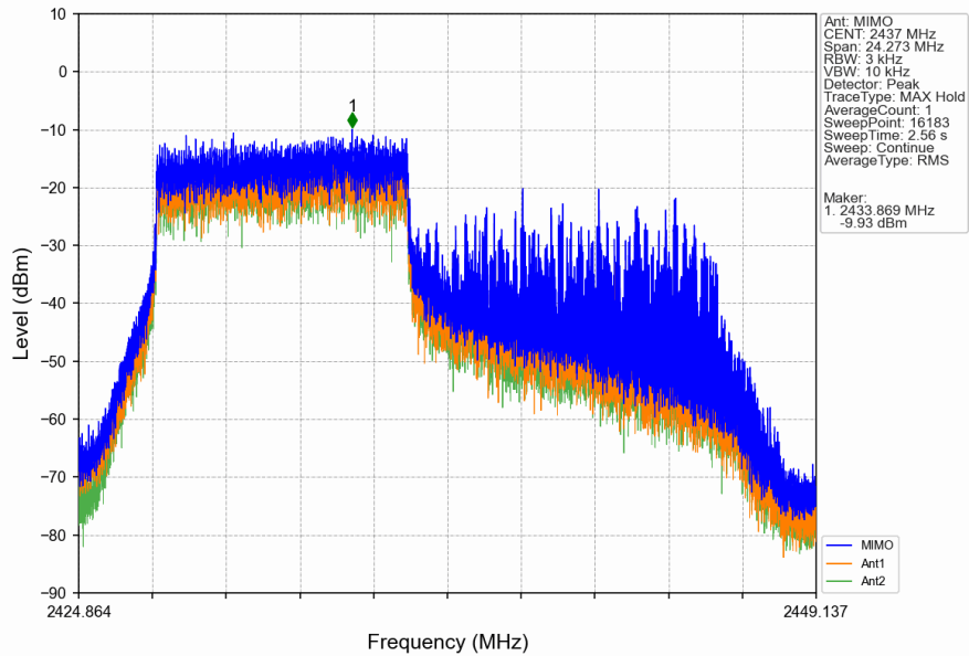
802.11ax(HEW20)_MCH_2437MHz_RU106_Left_MIMO_NTNV
