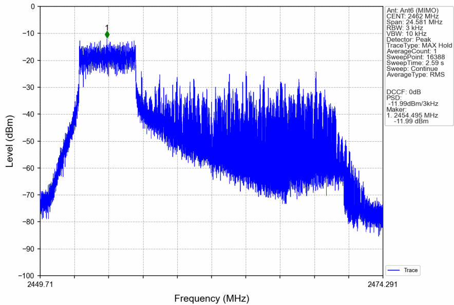
802.11ax(HEW20)_HCH_2462MHz_RU52_Left_Ant6 (MIMO)_NTNV
