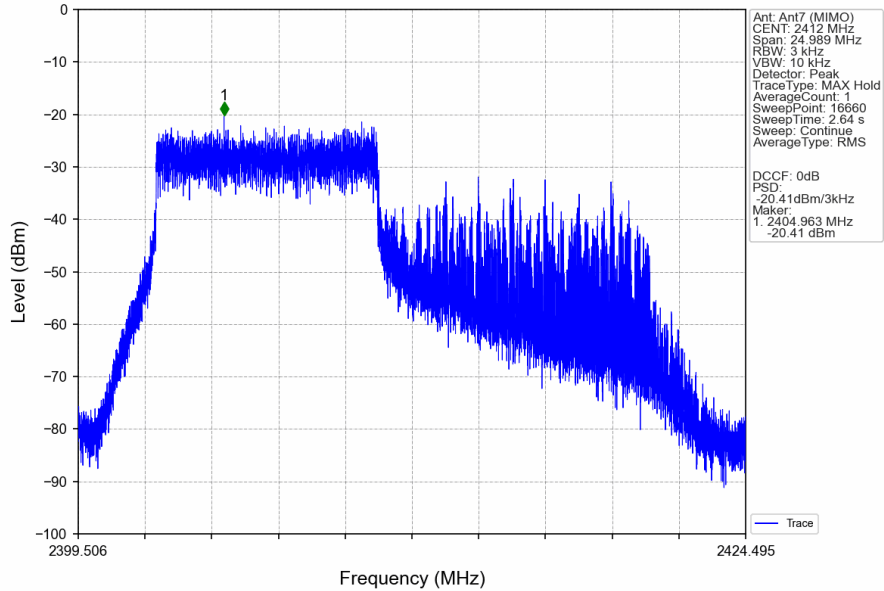
802.11ax(HEW20)_LCH_2412MHz_RU106_Left_Ant7 (MIMO)_NTNV
