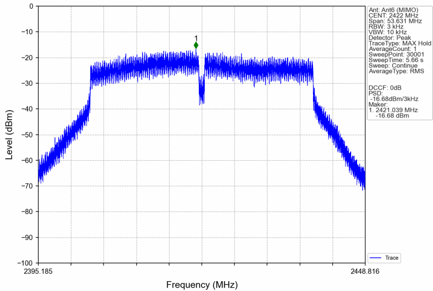
802.11n(HT40)_LCH_2422MHz_Ant6 (MIMO)_NTNV
