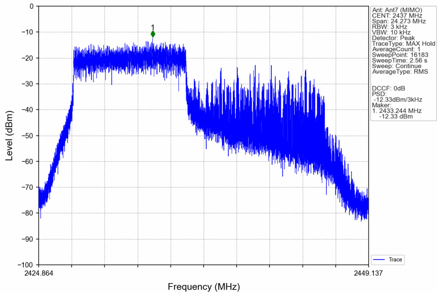
802.11ax(HEW20)_MCH_2437MHz_RU106_Left_Ant7 (MIMO)_NTNV
