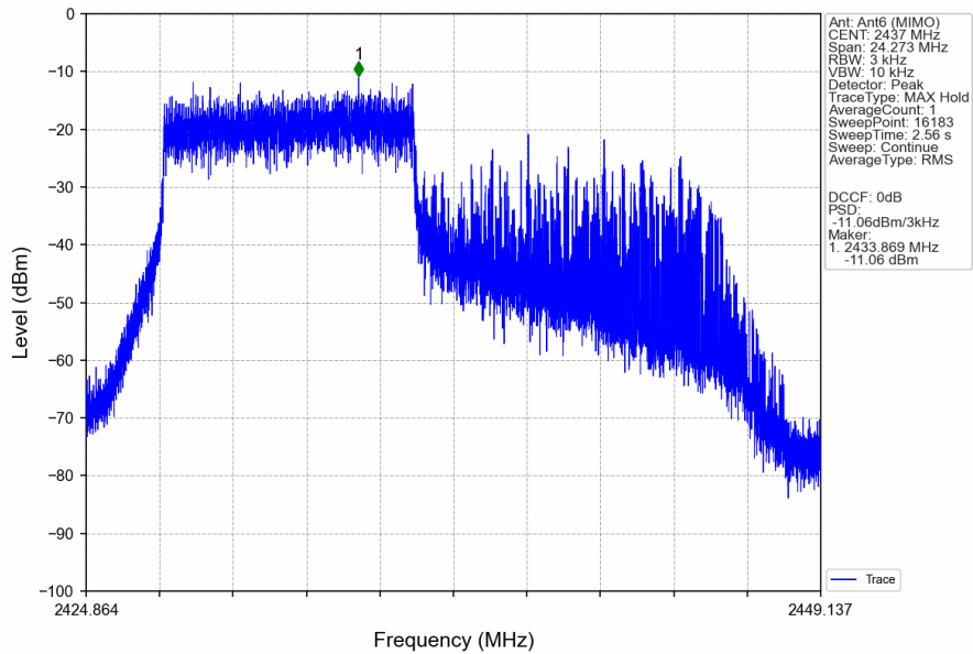
802.11ax(HEW20)_MCH_2437MHz_RU106_Left_Ant6 (MIMO)_NTNV
