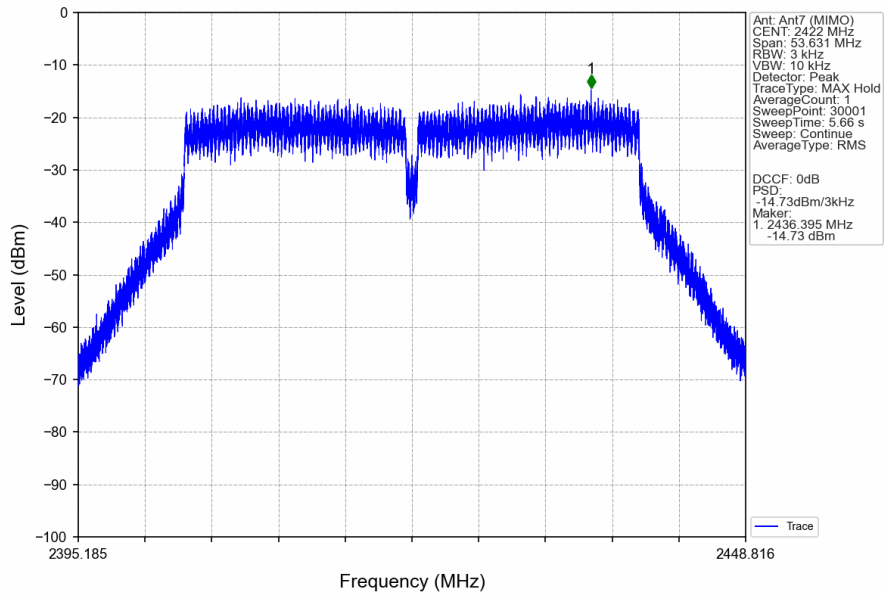
802.11n(HT40)_LCH_2422MHz_Ant7 (MIMO)_NTNV
