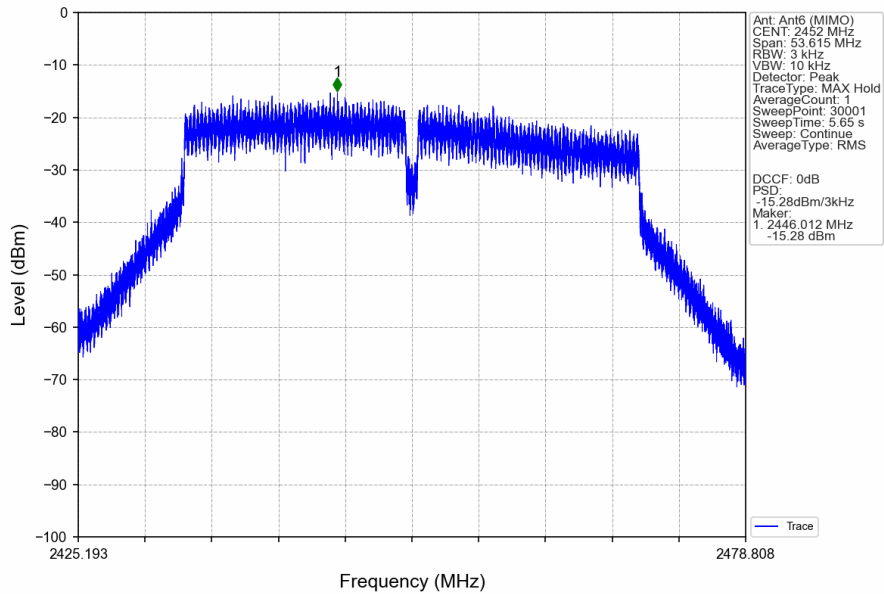
802.11n(HT40)_HCH_2452MHz_Ant6 (MIMO)_NTNV
