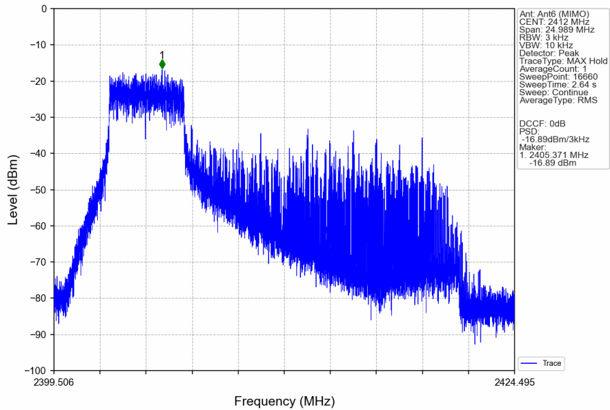
802.11ax(HEW20)_LCH_2412MHz_RU52_Left_Ant6 (MIMO)_NTNV
