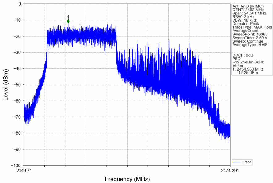
802.11ax(HEW20)_HCH_2462MHz_RU106_Left_Ant6 (MIMO)_NTNV
