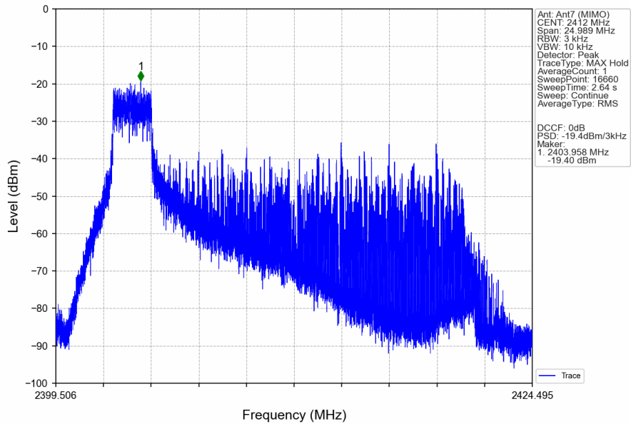
802.11ax(HEW20)_LCH_2412MHz_RU26_Left_Ant7 (MIMO)_NTNV
