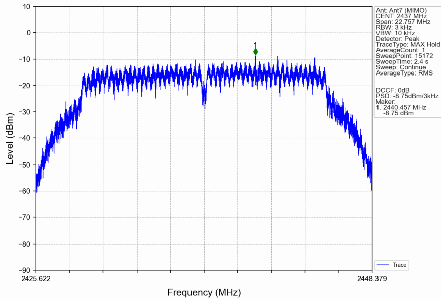
802.11g_MCH_2437MHz_Ant7 (MIMO)_NTNV
