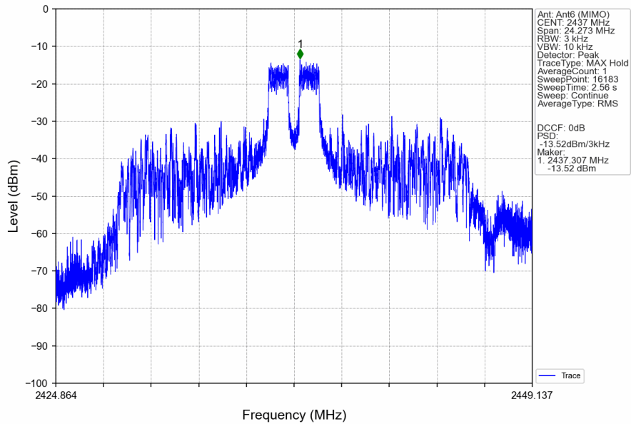
802.11ax(HEW20)_MCH_2437MHz_RU26_Mid_Ant6 (MIMO)_NTNV
