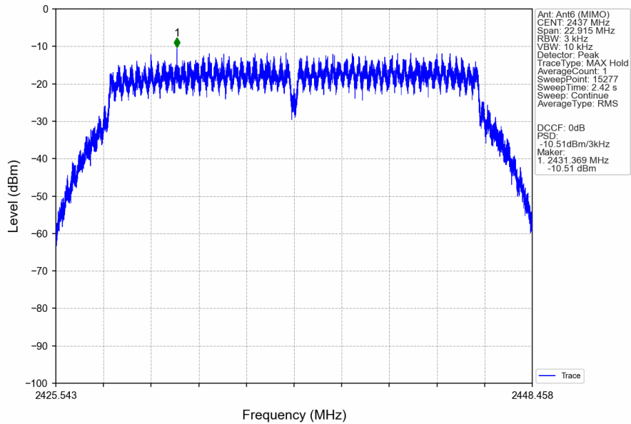
802.11n(HT20)_MCH_2437MHz_Ant6 (MIMO)_NTNV
