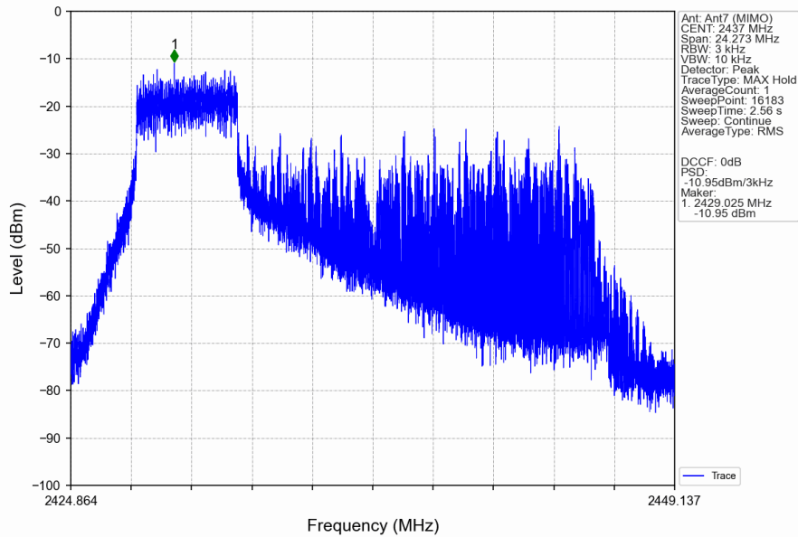
802.11ax(HEW20)_MCH_2437MHz_RU52_Left_Ant7 (MIMO)_NTNV
