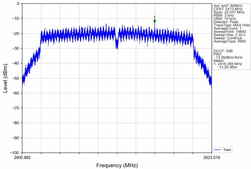
802.11n(HT20)_LCH_2412MHz_Ant7 (MIMO)_NTNV
