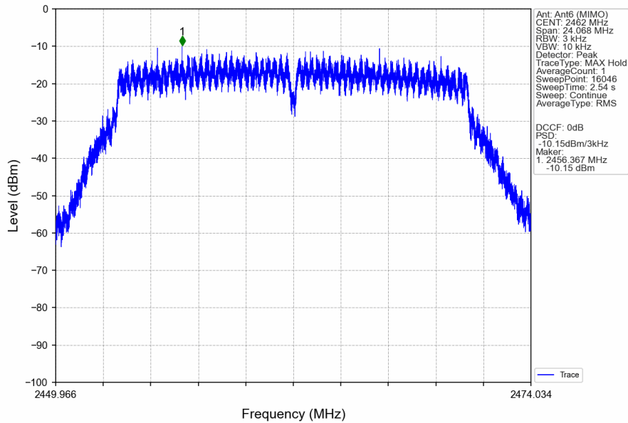
802.11n(HT20)_HCH_2462MHz_Ant6 (MIMO)_NTNV
