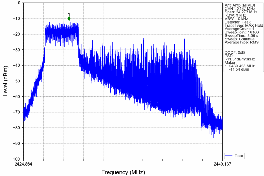
802.11ax(HEW20)_MCH_2437MHz_RU52_Left_Ant6 (MIMO)_NTNV
