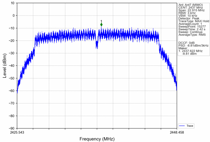
802.11n(HT20)_MCH_2437MHz_Ant7 (MIMO)_NTNV
