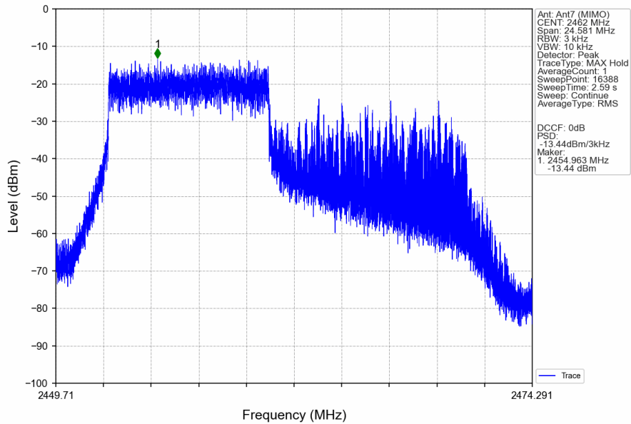
802.11ax(HEW20)_HCH_2462MHz_RU106_Left_Ant7 (MIMO)_NTNV
