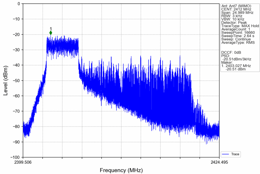
802.11ax(HEW20)_LCH_2412MHz_RU52_Left_Ant7 (MIMO)_NTNV
