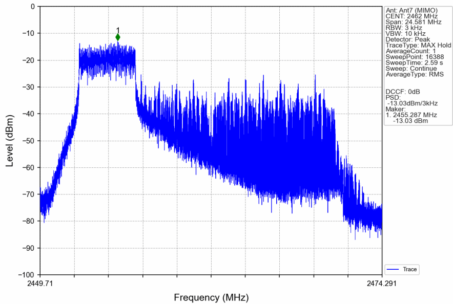
802.11ax(HEW20)_HCH_2462MHz_RU52_Left_Ant7 (MIMO)_NTNV
