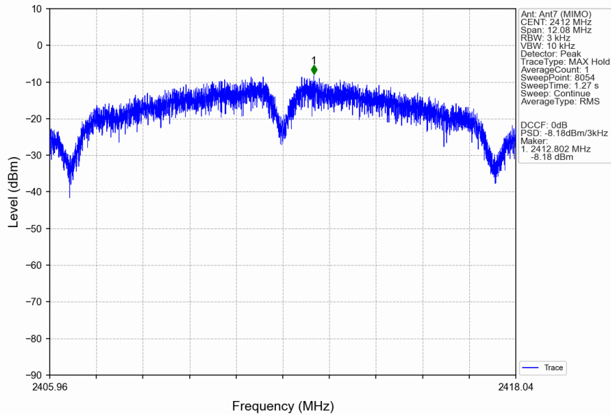
802.11b_LCH_2412MHz_Ant7 (MIMO)_NTNV
