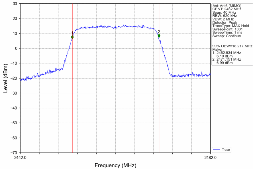
802.11n(HT20)_HCH_2462MHz_Ant6 (MIMO)_NTNV
