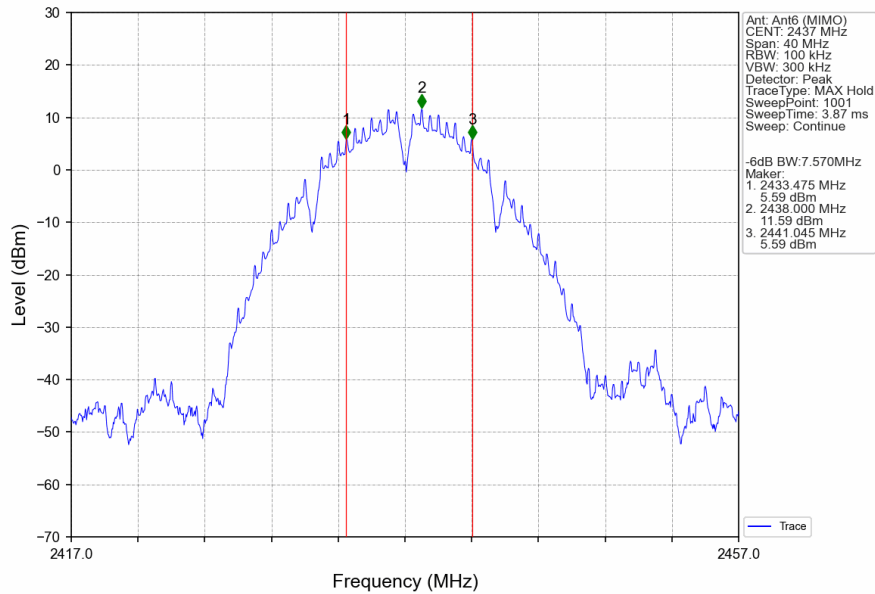
802.11b_MCH_2437MHz_Ant6 (MIMO)_NTNV
