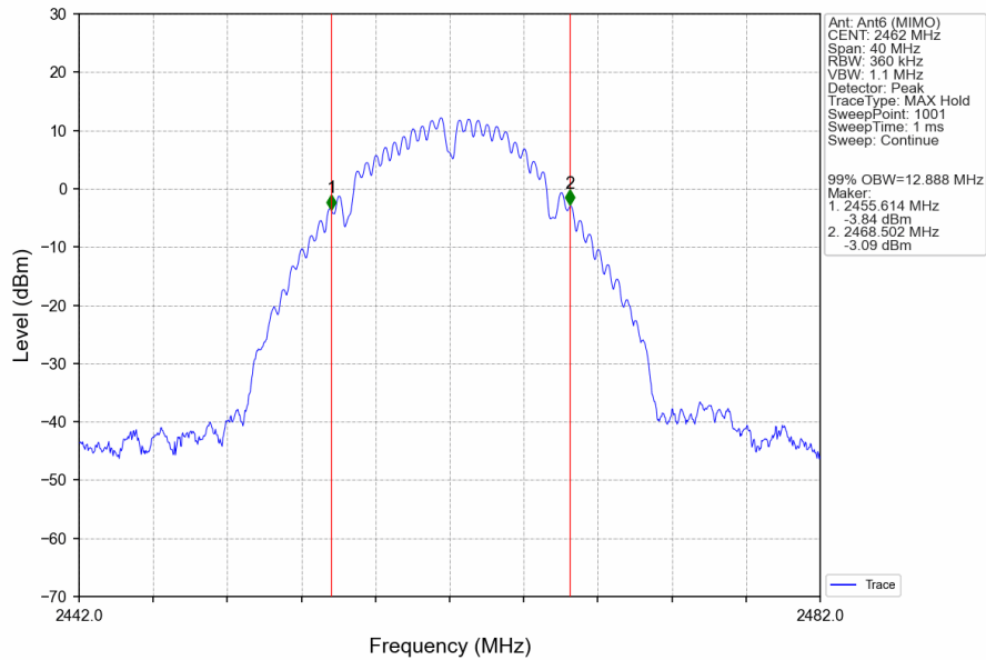
802.11b_HCH_2462MHz_Ant6 (MIMO)_NTNV
