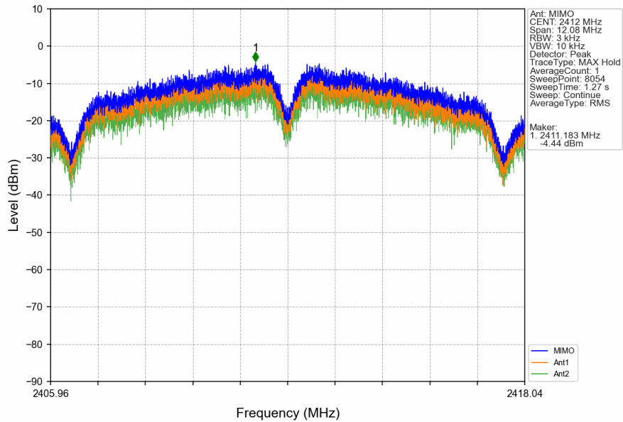
802.11b_LCH_2412MHz_MIMO_NTNV
