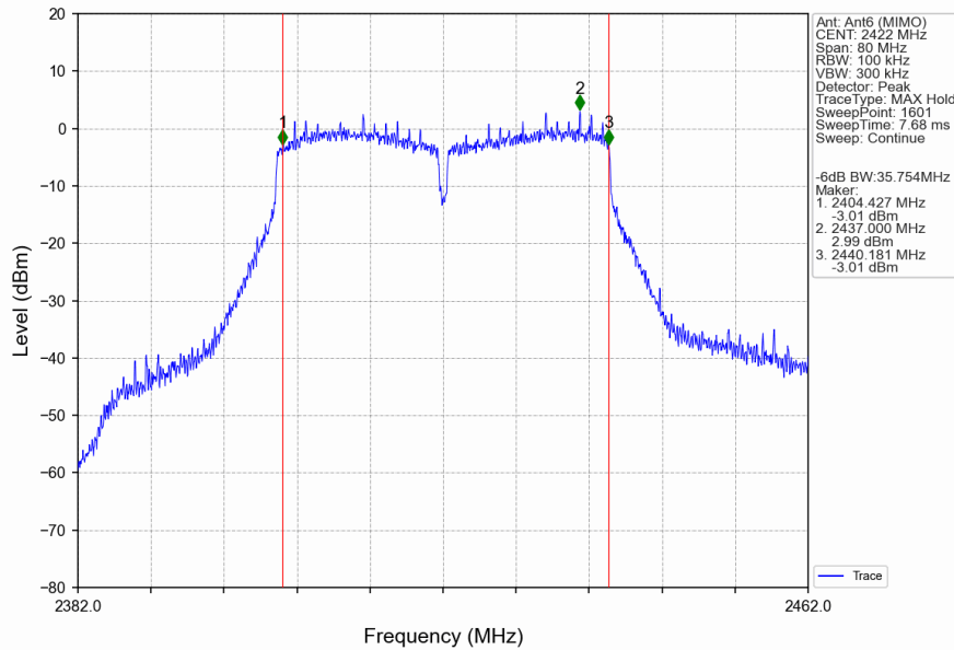
802.11n(HT40)_LCH_2422MHz_Ant6 (MIMO)_NTNV
