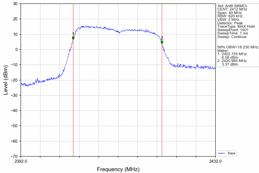
802.11n(HT20)_LCH_2412MHz_Ant6 (MIMO)_NTNV
