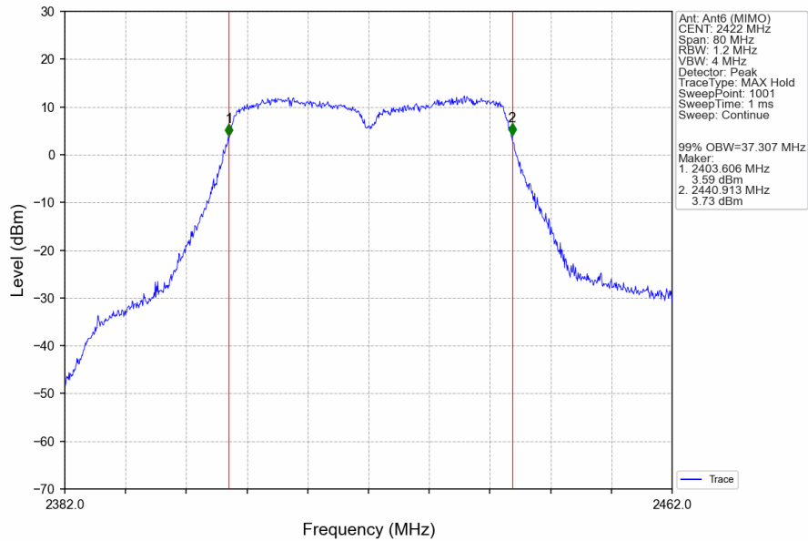
802.11n(HT40)_LCH_2422MHz_Ant6 (MIMO)_NTNV
