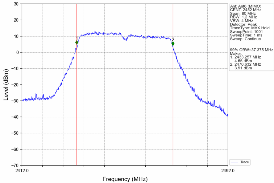
802.11n(HT40)_HCH_2452MHz_Ant6 (MIMO)_NTNV
