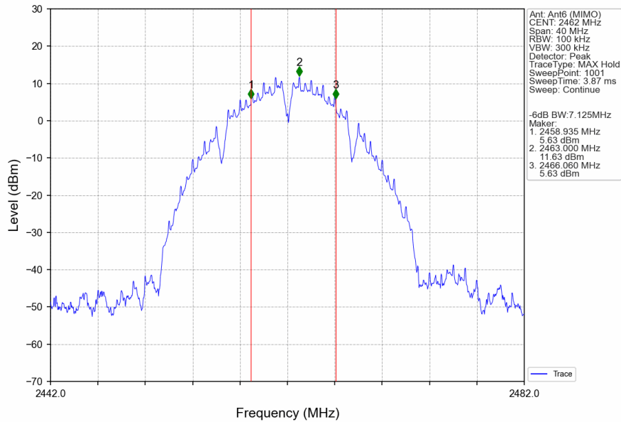
802.11b_HCH_2462MHz_Ant6 (MIMO)_NTNV
