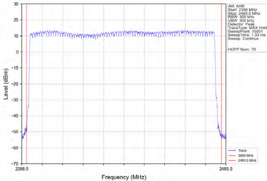
Pi/4DQPSK_2DH5_HOPP_Ant6_NTNV
