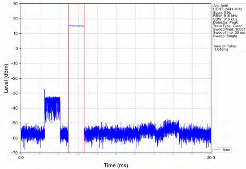
GFSK_DH3_HOPP_Ant6_NTNV
