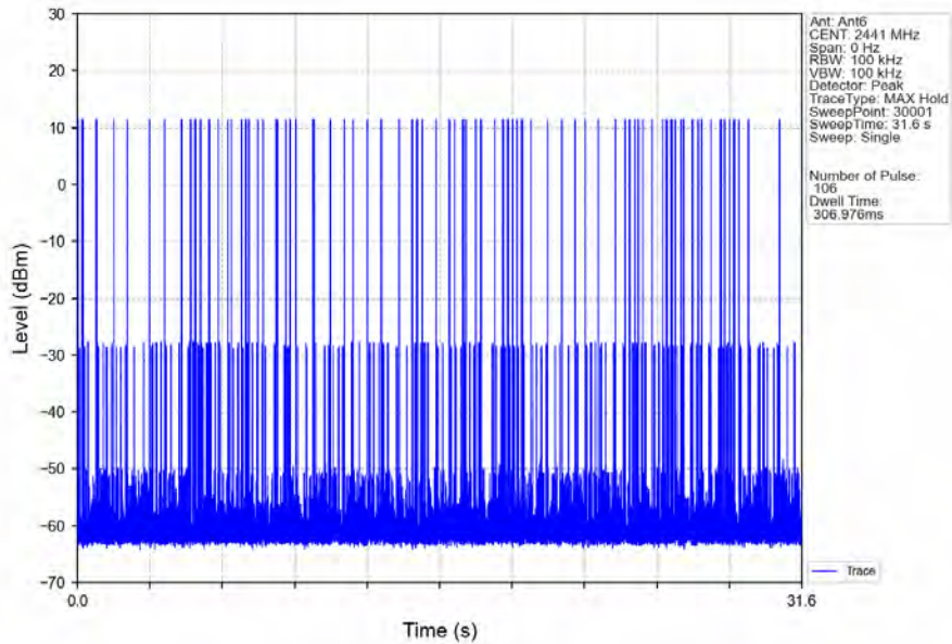
Pi/4DQPSK_2DH5_HOPP_Ant6_NTNV
