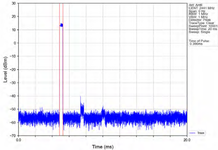
Pi/4DQPSK_2DH1_HOPP_Ant6_NTNV
