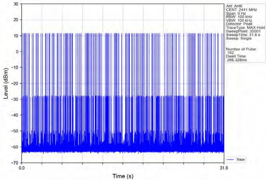
Pi/4DQPSK_2DH3_HOPP_Ant6_NTNV
