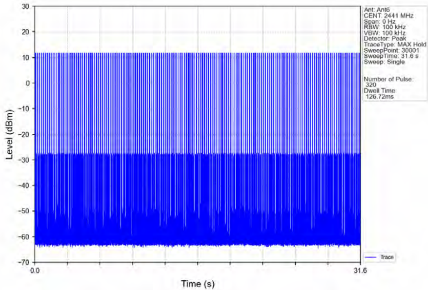
Pi/4DQPSK_2DH1_HOPP_Ant6_NTNV
