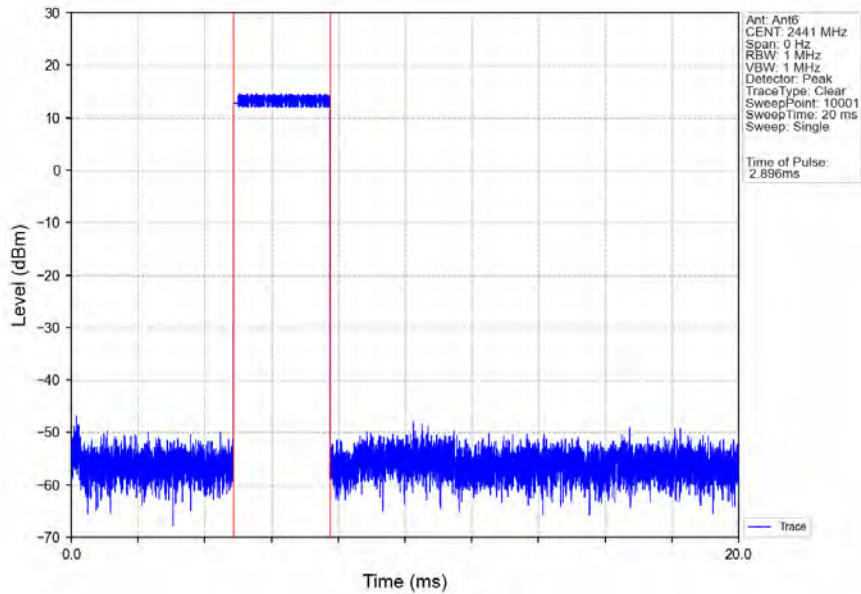
Pi/4DQPSK_2DH5_HOPP_Ant6_NTNV
