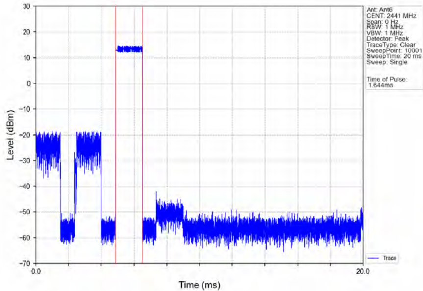
Pi/4DQPSK_2DH3_HOPP_Ant6_NTNV
