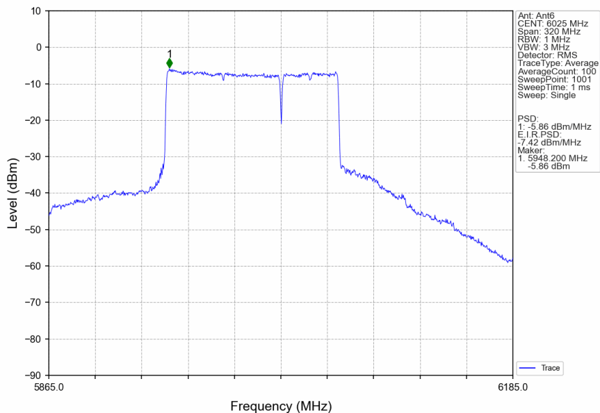
802.11be(EHT160)_LCH_6025MHz_484+996_/_Ant6_NTNV
