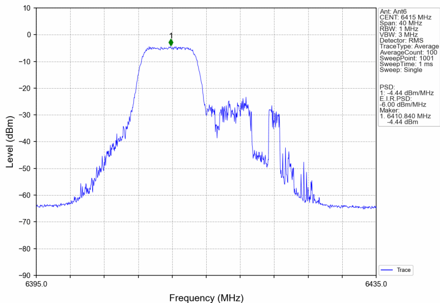
802.11be(EHT20)_HCH_6415MHz_26+52_/_Ant6_NTNV
