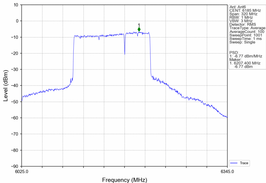
802.11be(EHT160)_MCH_6185MHz_484+996_/_Ant6_NTNV
