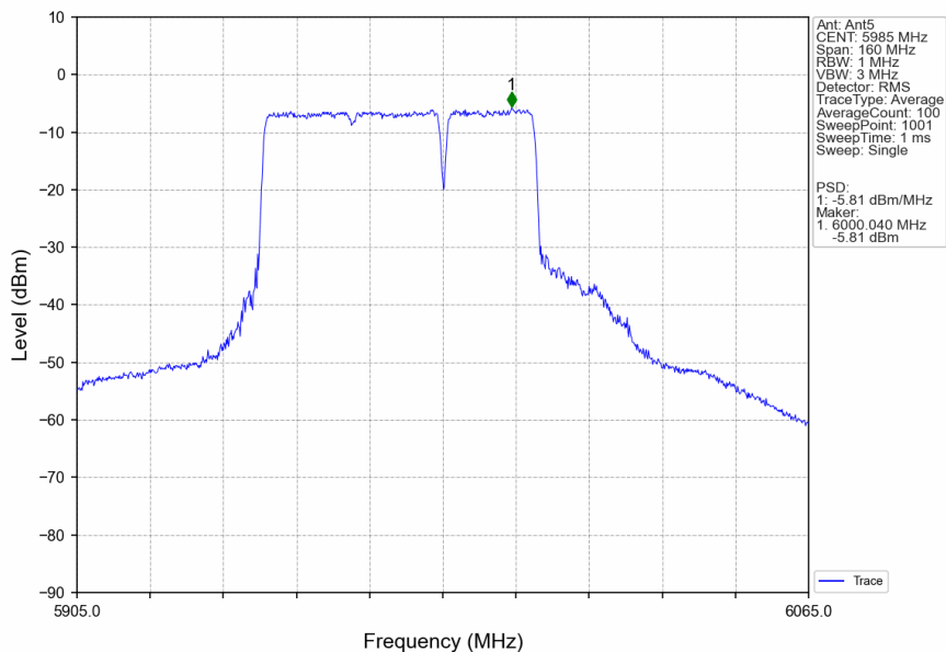
802.11be(EHT80)_LCH_5985MHz_242+484_/_Ant5_NTNV
