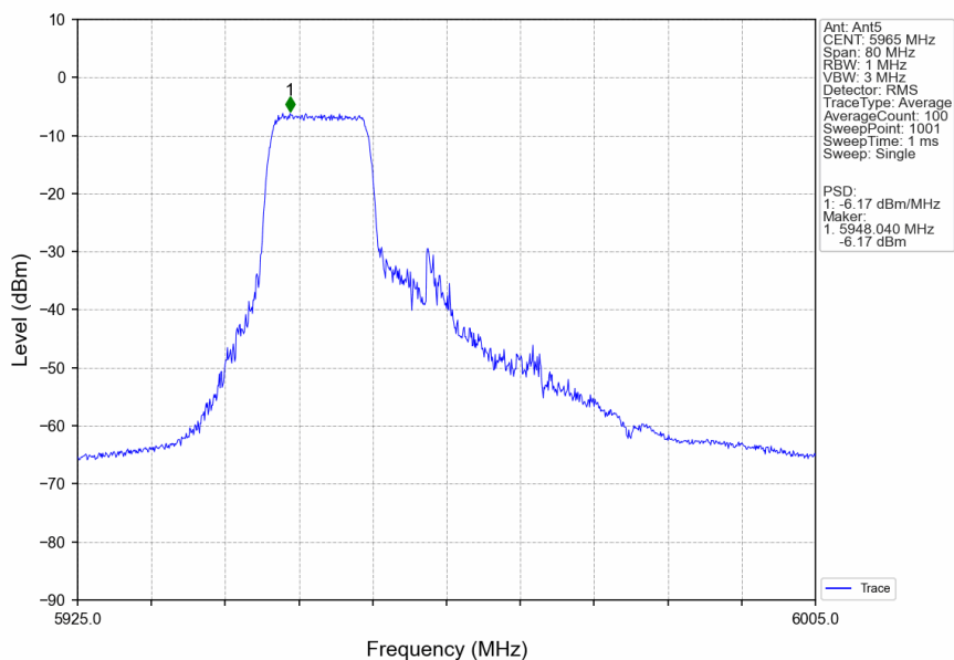
802.11be(EHT40)_LCH_5965MHz_26+106_/_Ant5_NTNV
