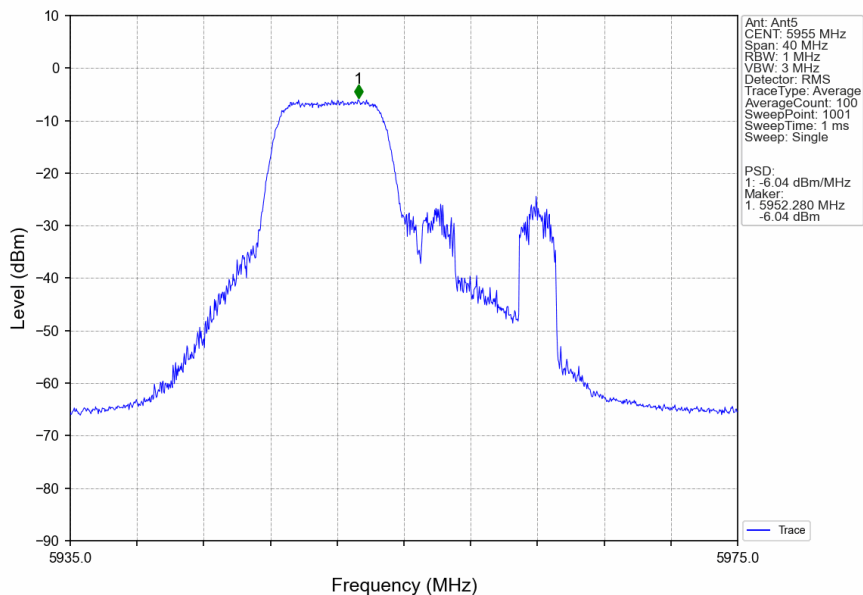
802.11be(EHT20)_LCH_5955MHz_26+52_/_Ant5_NTNV
