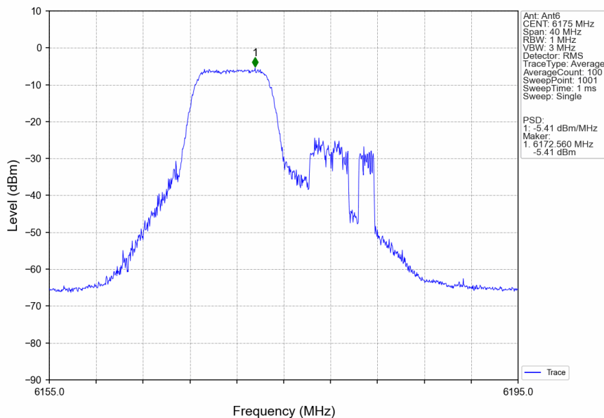
802.11be(EHT20)_MCH_6175MHz_26+52_/_Ant6_NTNV
