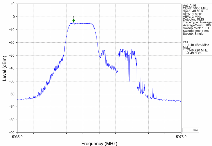
802.11be(EHT20)_LCH_5955MHz_26+52_/_Ant6_NTNV
