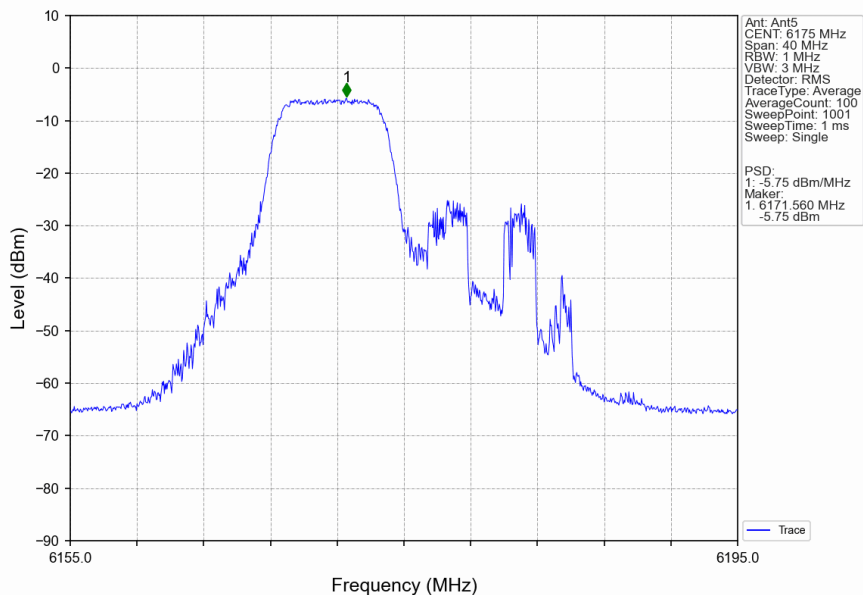
802.11be(EHT20)_MCH_6175MHz_26+52_/_Ant5_NTNV
