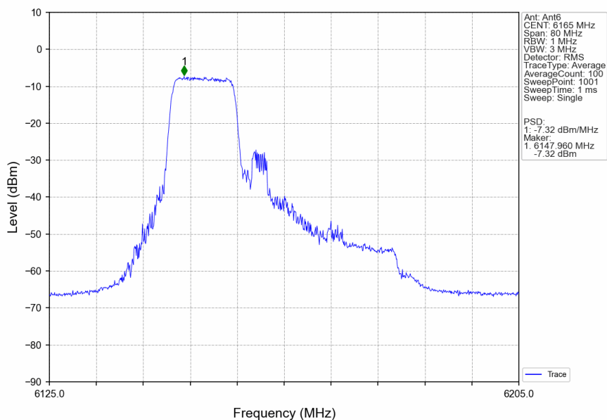
802.11be(EHT40)_MCH_6165MHz_26+106_/_Ant6_NTNV
