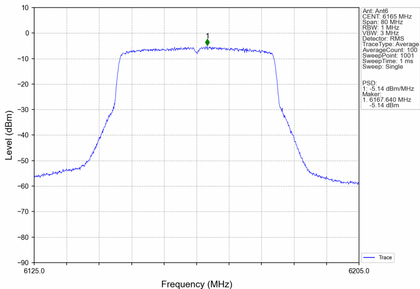
802.11be(EHT40)_MCH_6165MHz_SU_/_Ant6_NTNV
