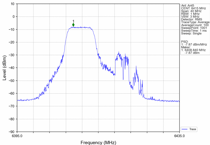
802.11be(EHT20)_HCH_6415MHz_26+52_/_Ant5_NTNV
