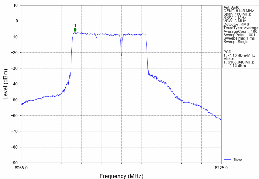
802.11be(EHT80)_MCH_6145MHz_242+484_/_Ant6_NTNV
