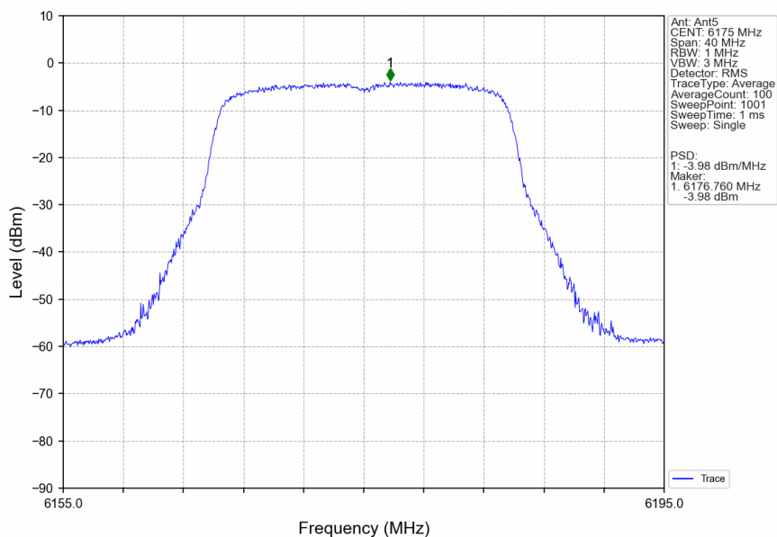
802.11be(EHT20)_MCH_6175MHz_SU_/_Ant5_NTNV
