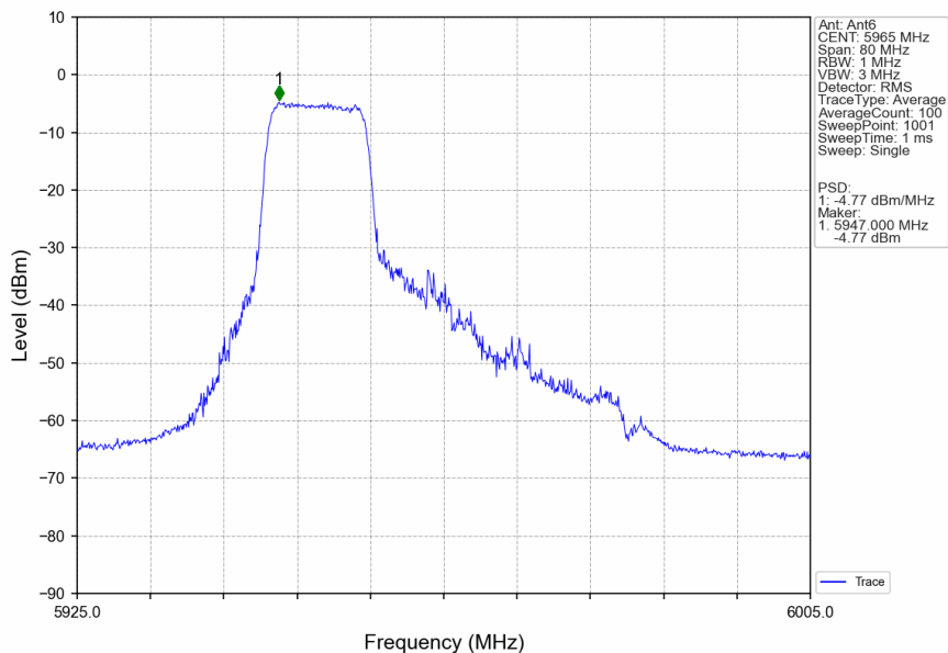
802.11be(EHT40)_LCH_5965MHz_26+106_/_Ant6_NTNV
