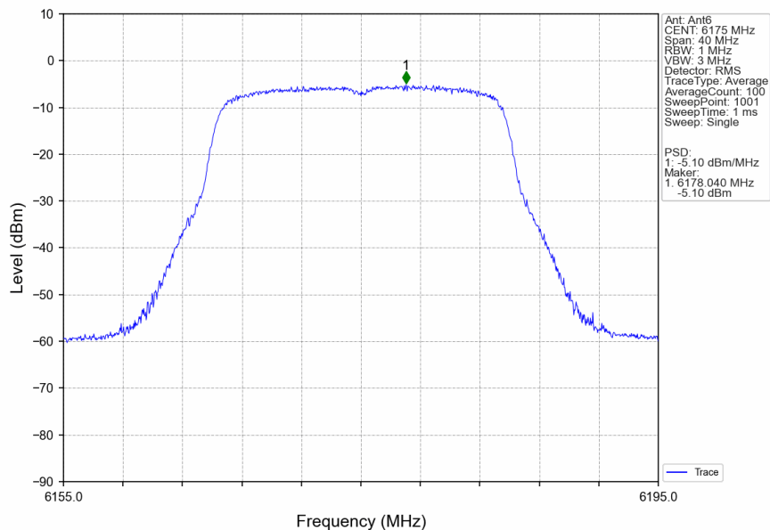
802.11be(EHT20)_MCH_6175MHz_SU_/_Ant6_NTNV
