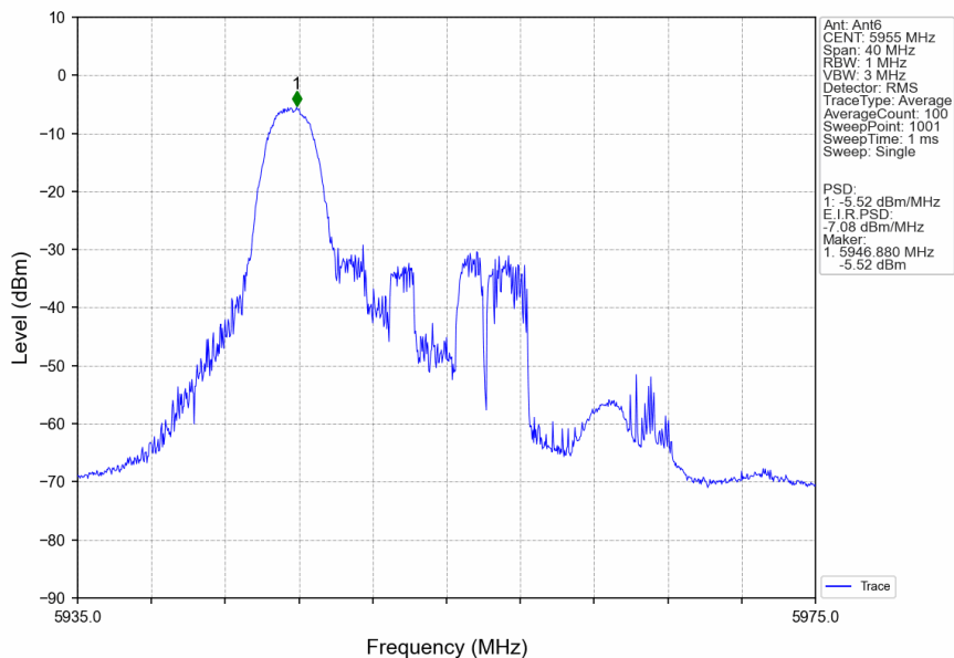
802.11ax(HEW20)_LCH_5955MHz_RU26_Left_Ant6_NTNV
