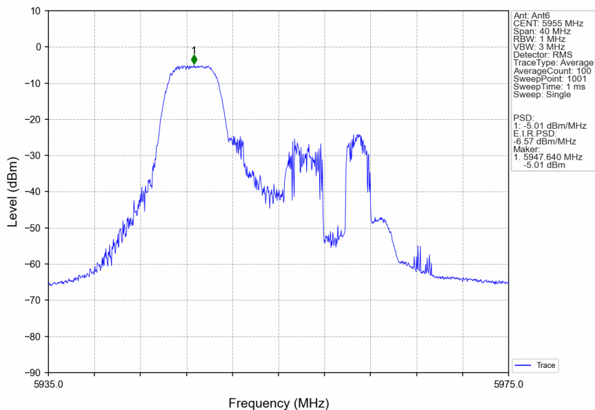
802.11ax(HEW20)_LCH_5955MHz_RU52_Left_Ant6_NTNV
