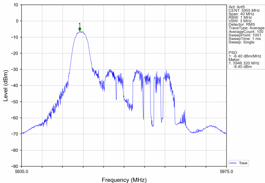
802.11ax(HEW20)_LCH_5955MHz_RU26_Left_Ant5_NTNV
