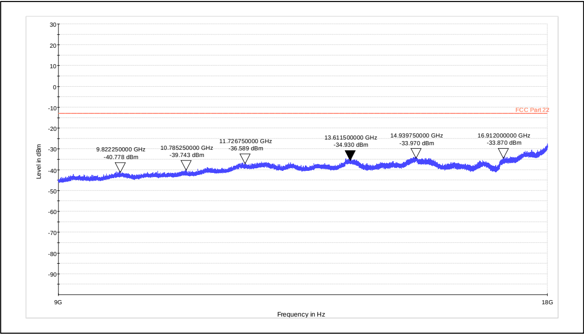
Frequency range: 9GHz-18GHz
