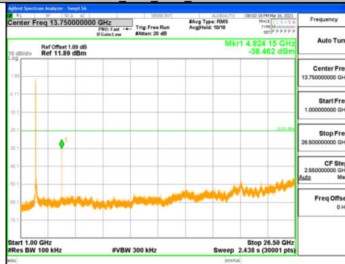
11B_Ant1_2412_1000~26500
