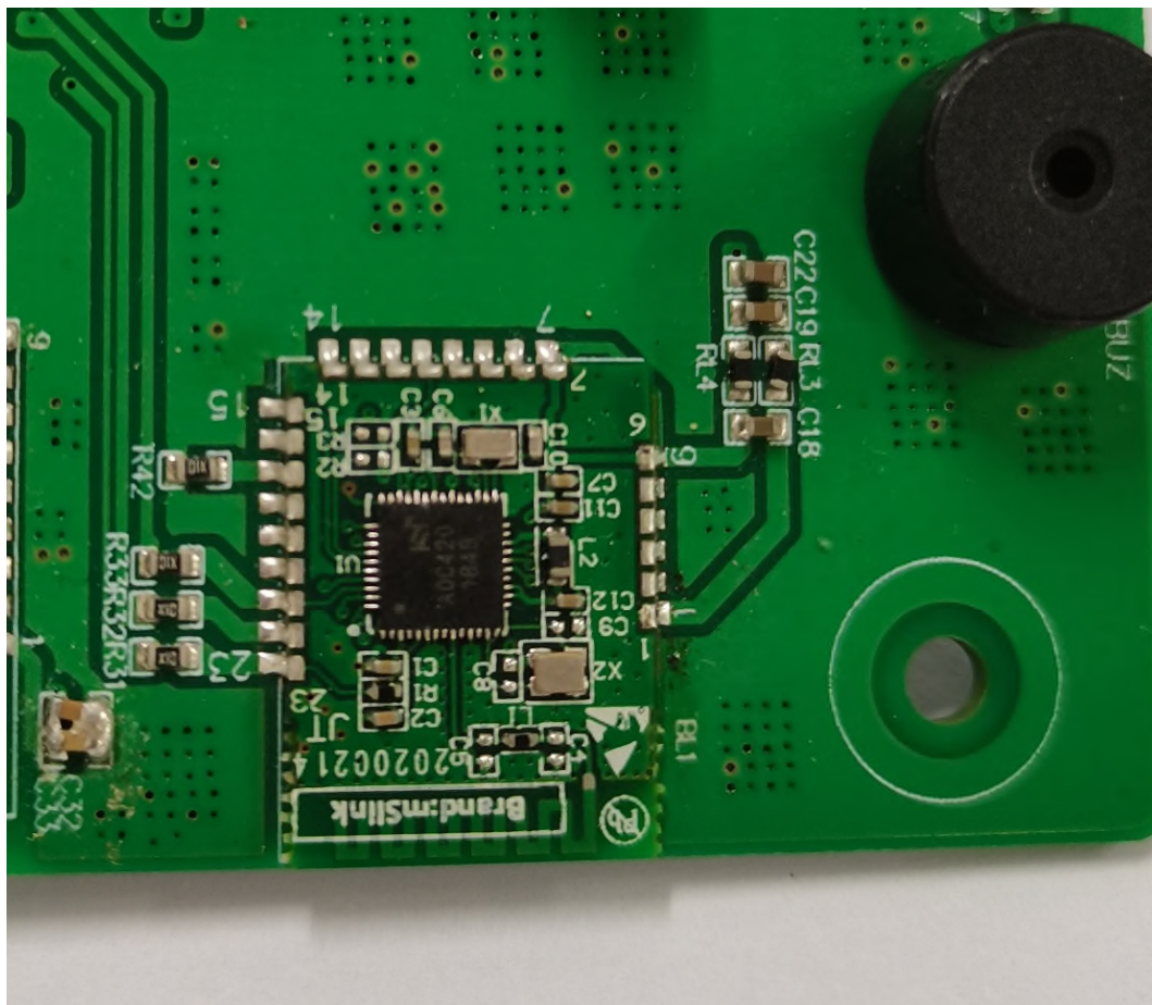
Bluetooth module
