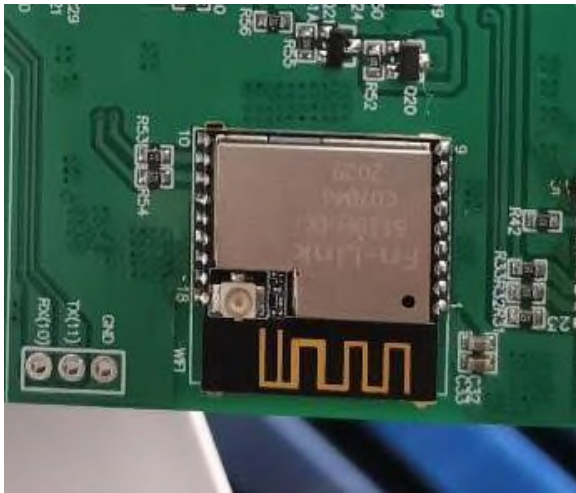
Wi-Fi module
