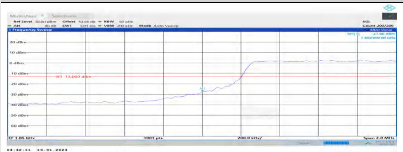
Band2-5MHz-QPSK-19175-1RB#24
