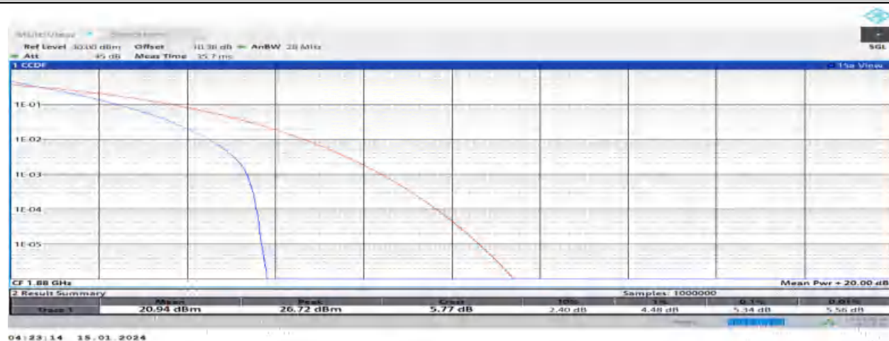
Band2-20MHz-QPSK-19100-100RB#0
