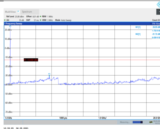
Band66-20MHz-QPSK-132322-1RB#0- Range2:1000~20000MHz
