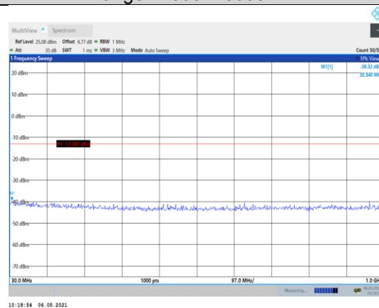
Band4-5MHz-QPSK-20375-1RB#0- Range1:30~1000MHz
