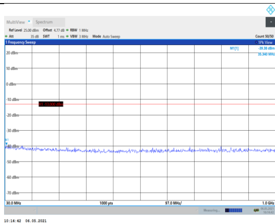
Band4-10MHz-QPSK-20000-1RB#0- Range1:30~1000MHz
