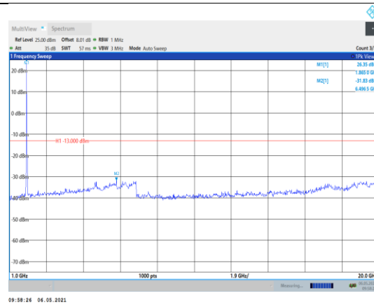
Band2-20MHz-16QAM-18900-1RB#0- Range2:1000~20000MHz
