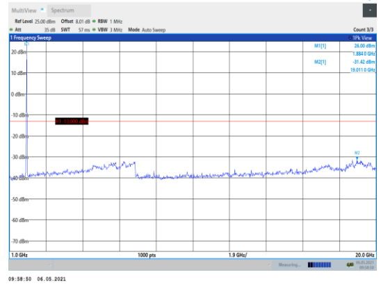
Band2-20MHz-QPSK-19100-1RB#0- Range2:1000~20000MHz
