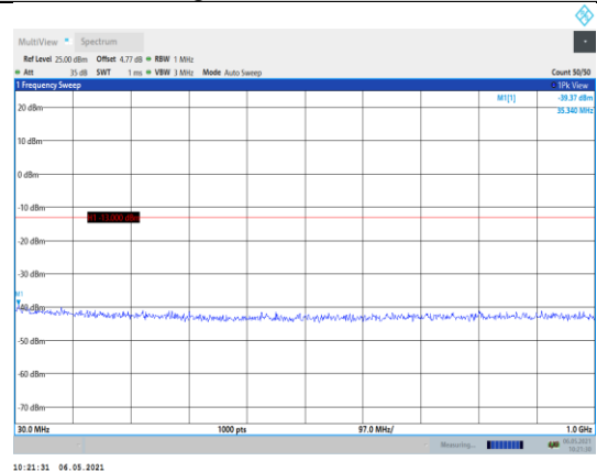
Band4-1.4MHz-QPSK-20393-1RB#0- Range1:30~1000MHz
