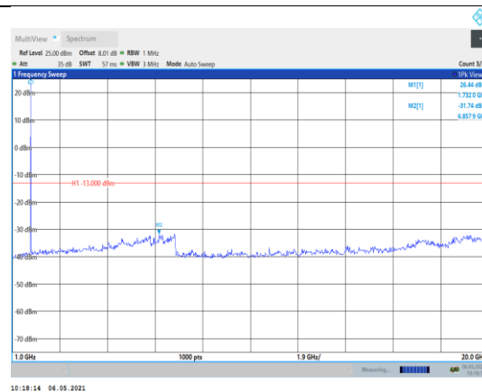
Band4-5MHz-QPSK-20175-1RB#0- Range2:1000~20000MHz
