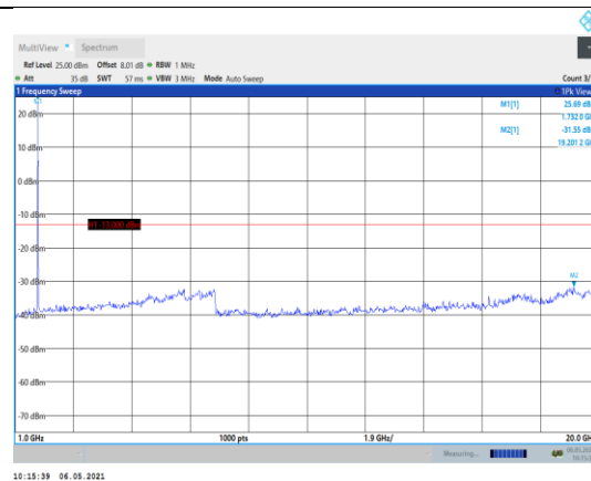
Band4-10MHz-QPSK-20175-1RB#0- Range2:1000~20000MHz
