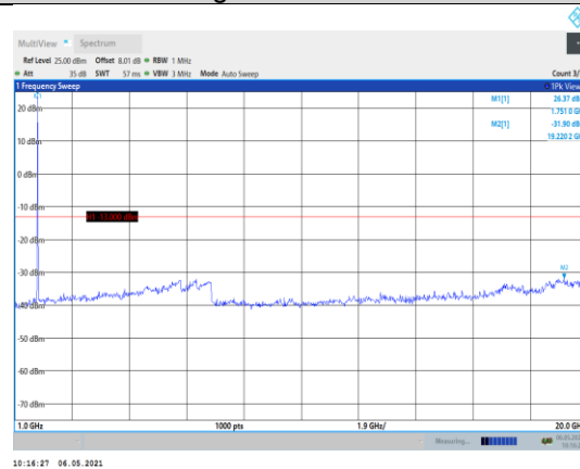
Band4-10MHz-QPSK-20350-1RB#0- Range2:1000~20000MHz
