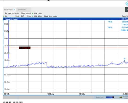
Band66-10MHz-QPSK-132622-1RB#0- Range2:1000~20000MHz
