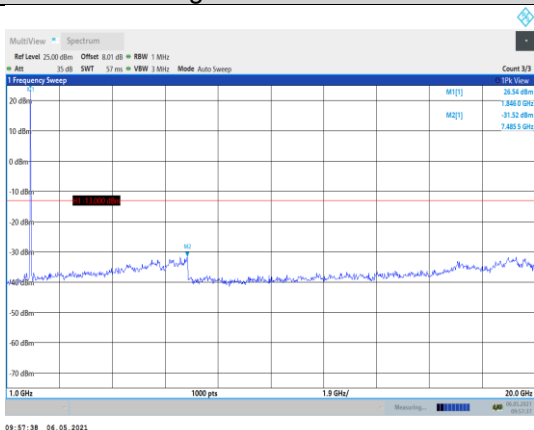
Band2-20MHz-16QAM-18700-1RB#0- Range2:1000~20000MHz
