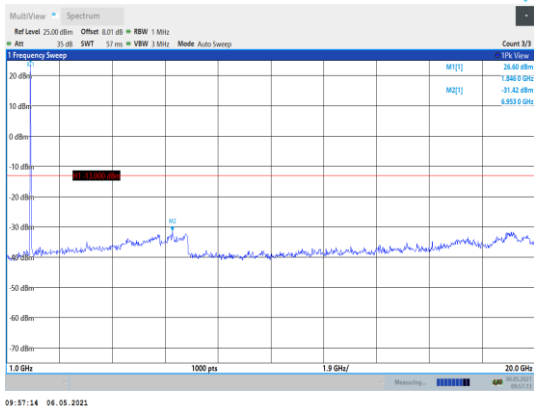
Band2-20MHz-QPSK-18700-1RB#0- Range2:1000~20000MHz
