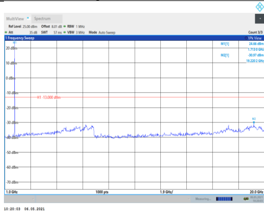
Band4-1.4MHz-QPSK-19957-1RB#0- Range2:1000~20000MHz
