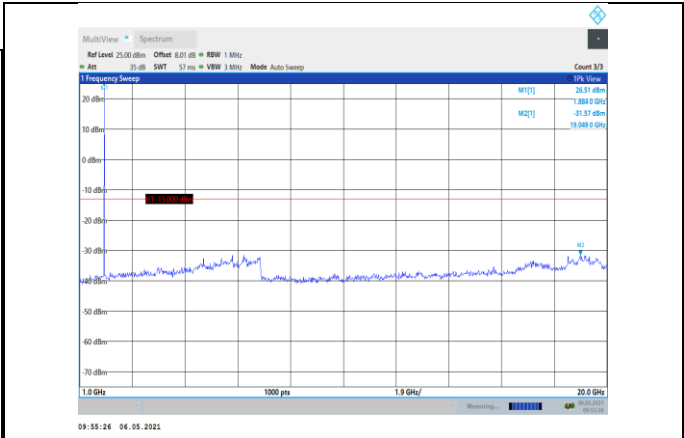
Band2:1.4MHz-QPSK-18900-1RB#0- Range2:1000~20000MHz
