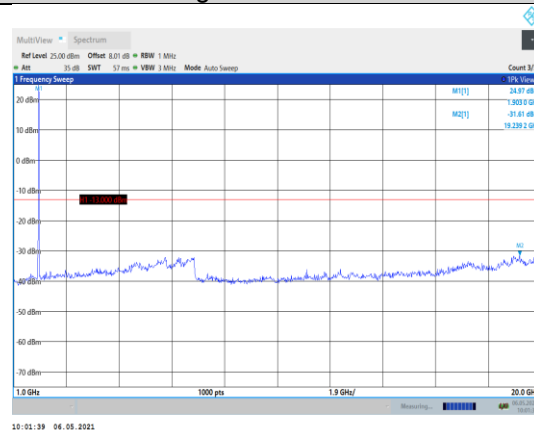
Band2-15MHz-QPSK-19125-1RB#0- Range2:1000~20000MHz
