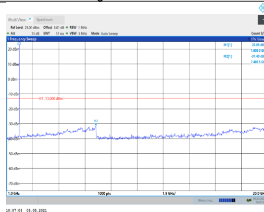
Band2-3MHz-QPSK-19185-1RB#0- Range2:1000~20000MHz
