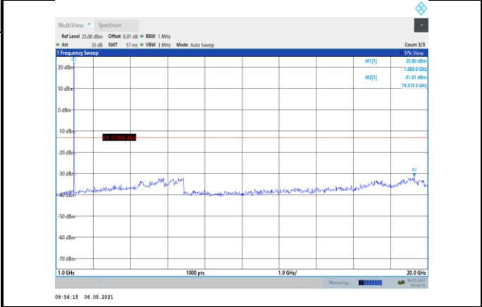
Band2-1.4MHz-QPSK-19193-1RB#0- Range2:1000~20000MHz
