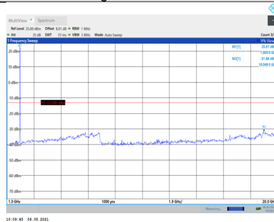
Band2-10MHz-QPSK-19150-1RB#0- Range2:1000~20000MHz
