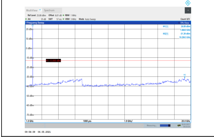
Band2:1.4MHz-QPSK-18607-1RB#0- Range2:1000~20000MHz
