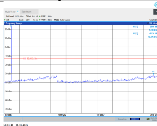
Band2-5MHz-16QAM-19175-1RB#0- Range2:1000~20000MHz
