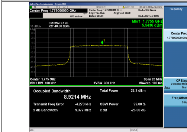
Band66-10MHz-QPSK-132622-50RB#0-8.9214
