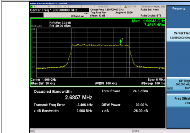
Band2-3MHz-QPSK-19185-15RB#0-2.6857
