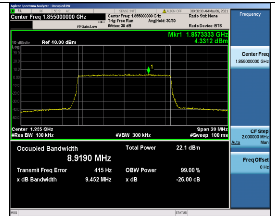
Band2-10MHz-16QAM-18650-50RB#0-8.9190
