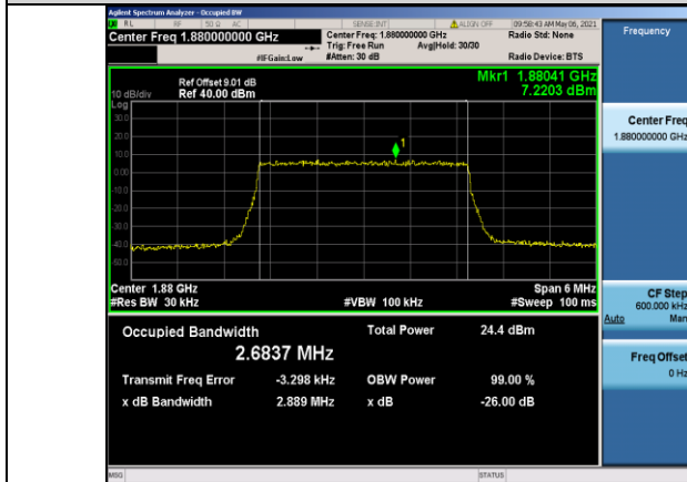
Band2-3MHz-QPSK-18900-15RB#0-2.6837
