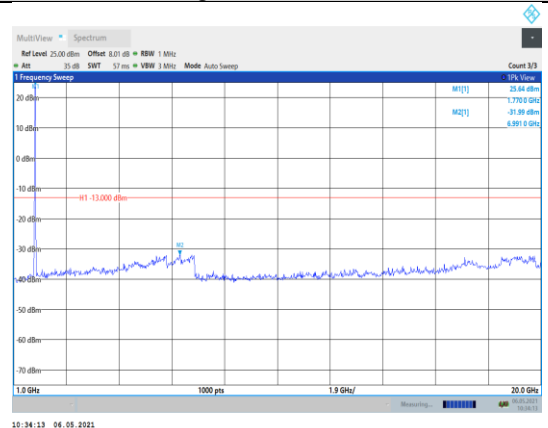
Band66-20MHz-QPSK-132572-1RB#0- Range2:1000~20000MHz
