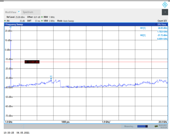
Band66-20MHz-QPSK-132322-1RB#0- Range2:1000~20000MHz
