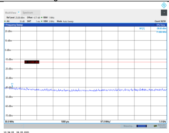
Band66-20MHz-QPSK-132572-1RB#0- Range1:30~1000MHz
