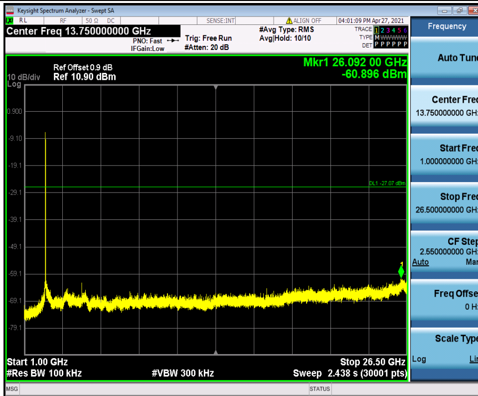
11G_Ant1_2412_1000~26500
