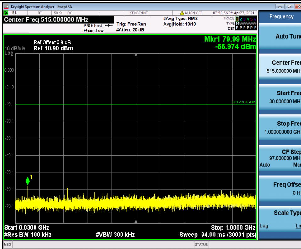
11B_Ant1_2462_30~1000
