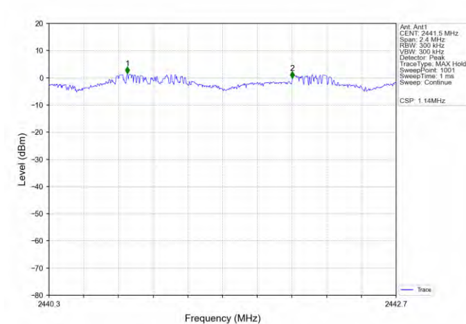
8DPSK_3DH5_HOPP_Ant1_NTNV
