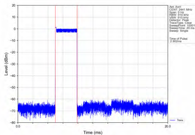
Pi/4DQPSK_2DH5_HOPP_Ant1_NTNV
