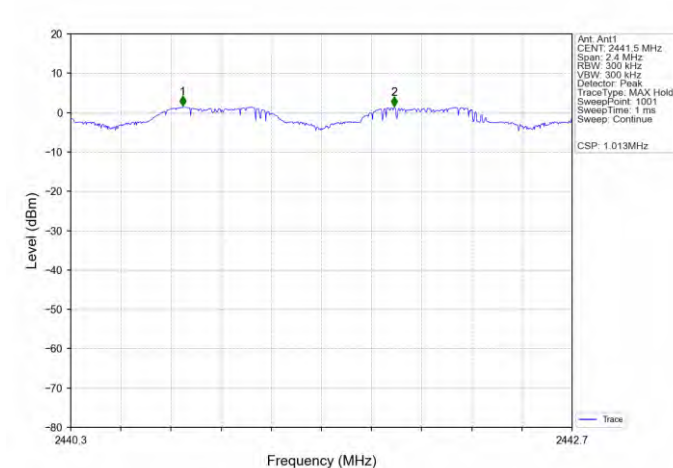
Pi/4DQPSK_2DH5_HOPP_Ant1_NTNV
