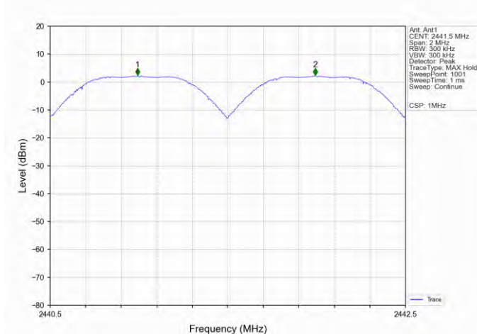
GFSK_DH5_HOPP_Ant1_NTNV
