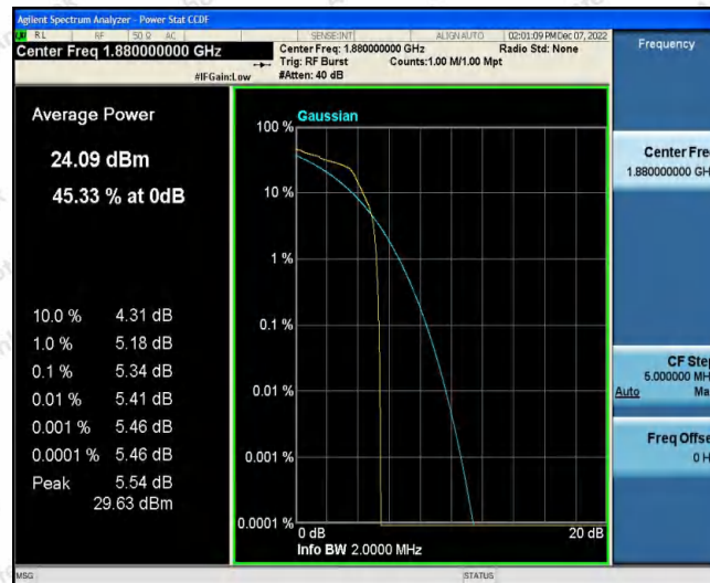
EGPRS1900-810
