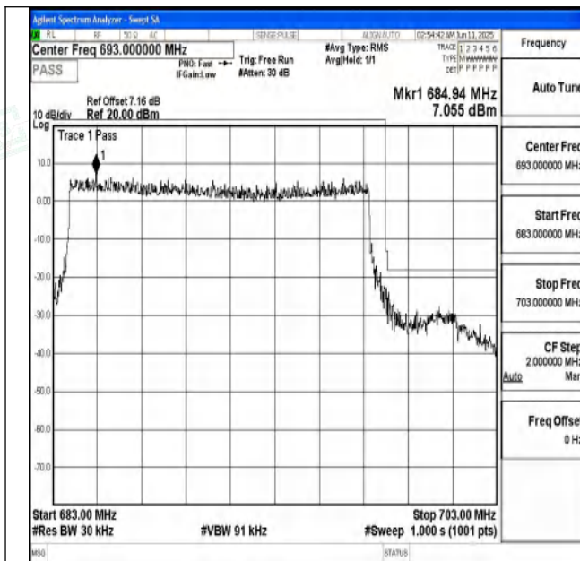
Band71_15MHz_QPSK_133397_75RB#0
