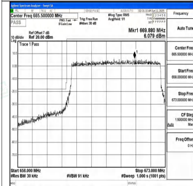
Band71_10MHz_QPSK_133172_50RB#0
