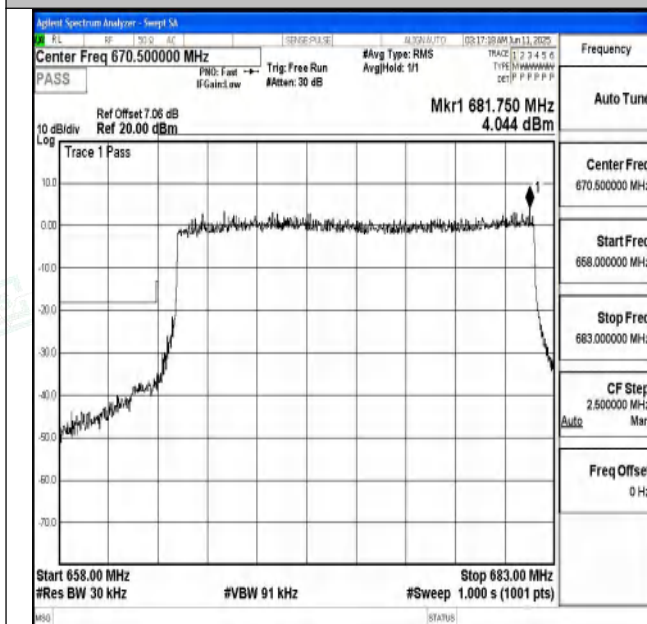
Band71_20MHz_QPSK_133222_100RB#0
