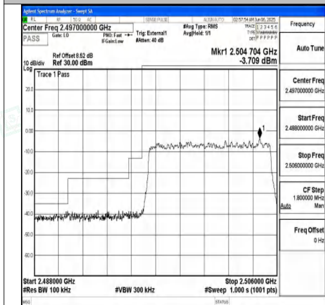
Band41_10MHz_QPSK_39700_50RB#0
