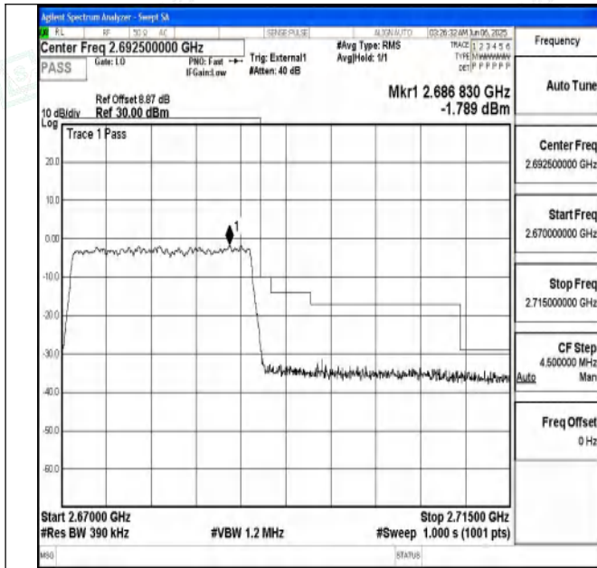
Band41_20MHz_QPSK_41490_100RB#0
