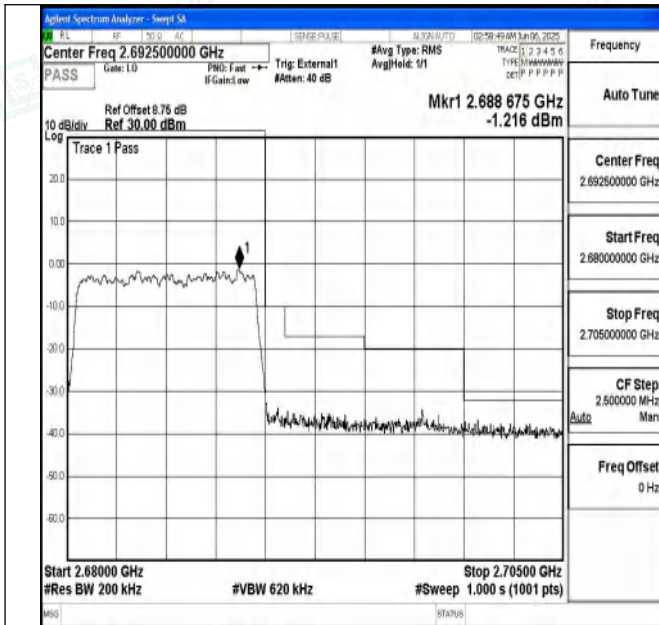
Band41_10MHz_QPSK_41540_50RB#0
