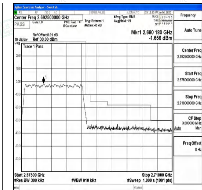
Band41_15MHz_QPSK_41515_75RB#0
