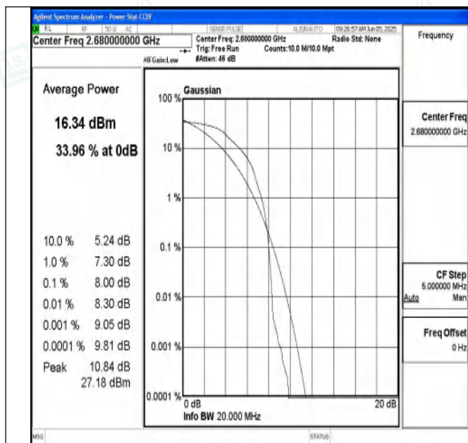
Band41-20MHz-QPSK-41490-1RB#0-PASS
