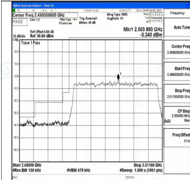
Band41_15MHz_QPSK_39725_75RB#0
