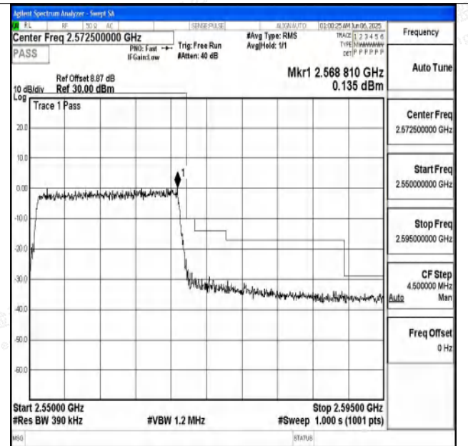
Band7_20MHz_16QAM_21350_100RB#0
