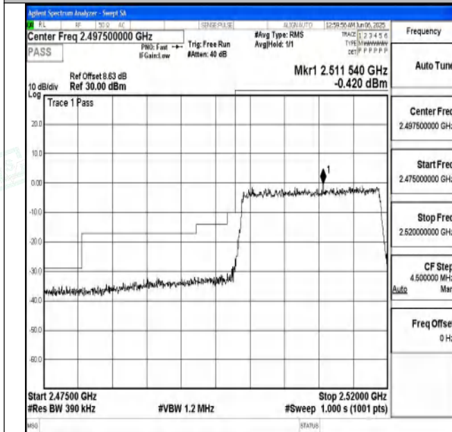
Band7_20MHz_QPSK_20850_100RB#0
