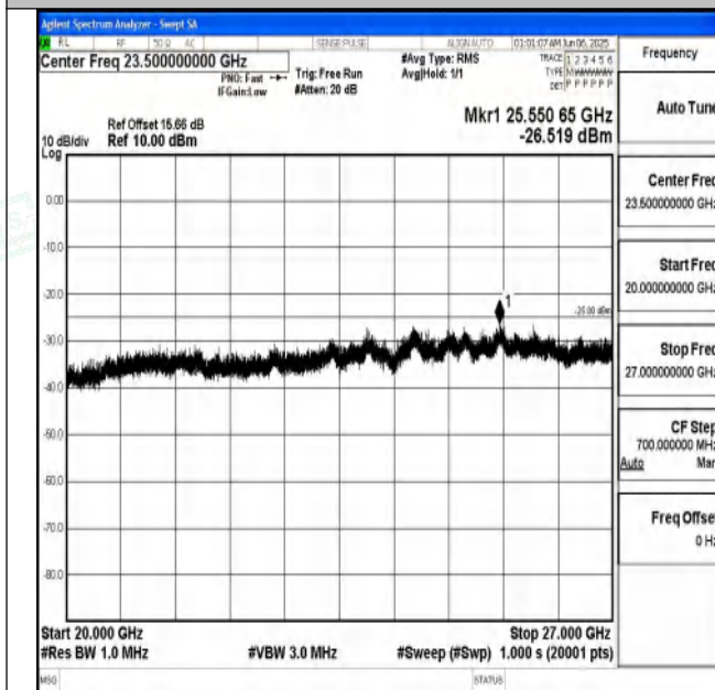
Band7_20MHz_QPSK_20850_1RB#0_20000~27000_20000~27000
