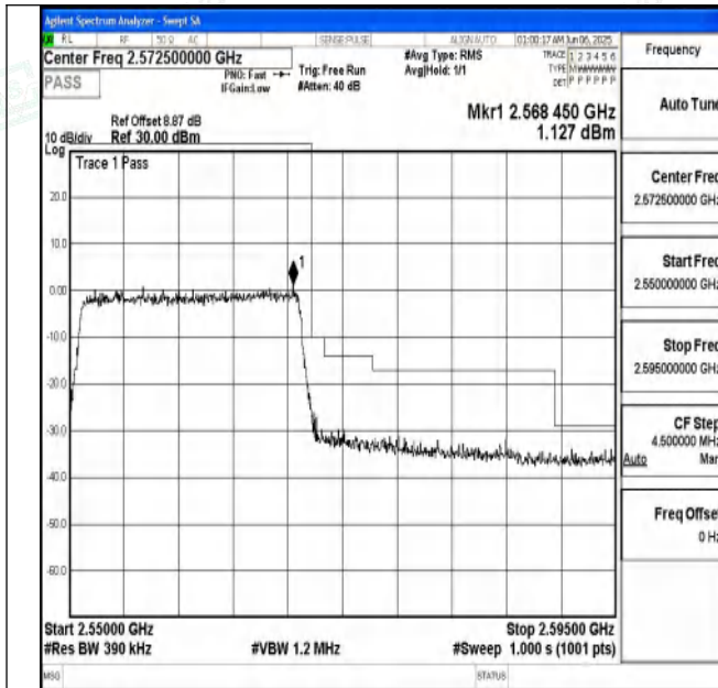
Band7_20MHz_QPSK_21350_100RB#0
