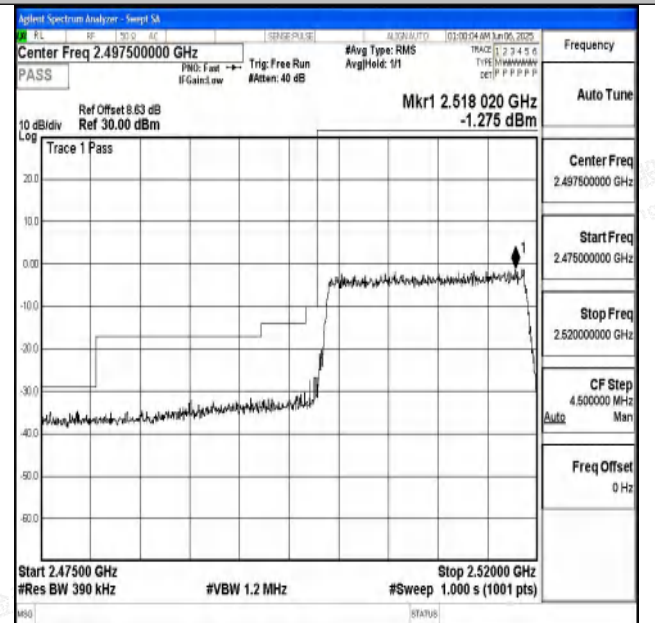
Band7_20MHz_16QAM_20850_100RB#0
